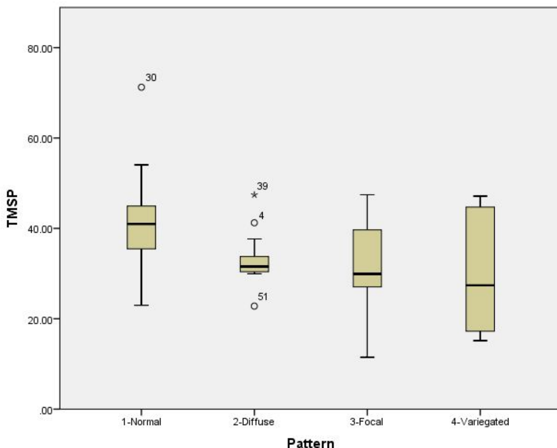
Figure 6.10 Θηκόγραμμα TMSP με Πρότυπο
