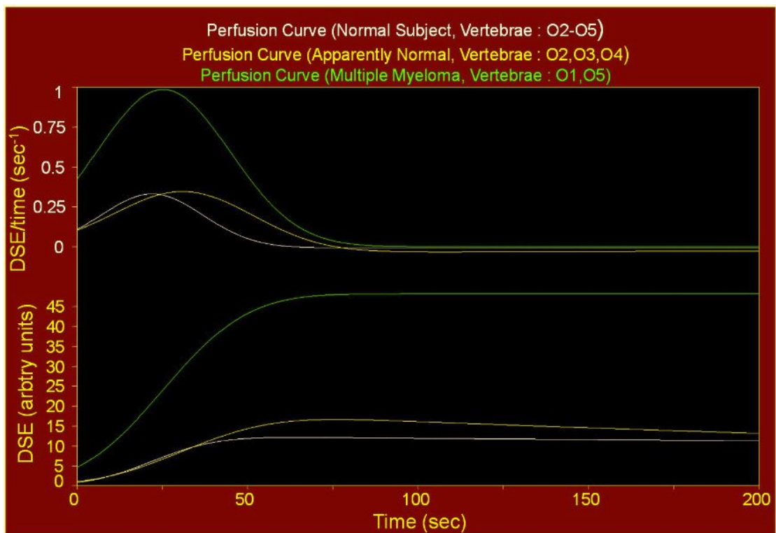
Figure 3.5 Συγκενρωτική Καμπύλη DCE-MRI τριών περιστατικών
