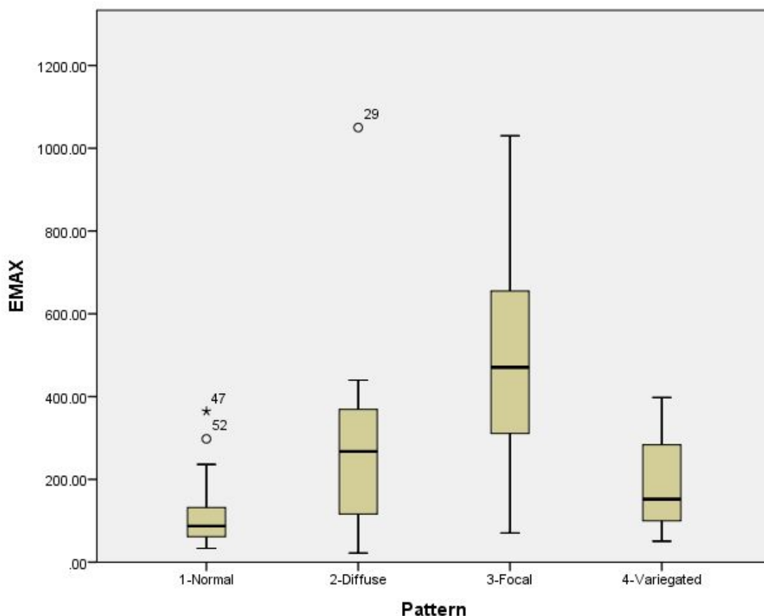
Figure 6.7 Θηκόγραμμα EMAX με Πρότυπο
