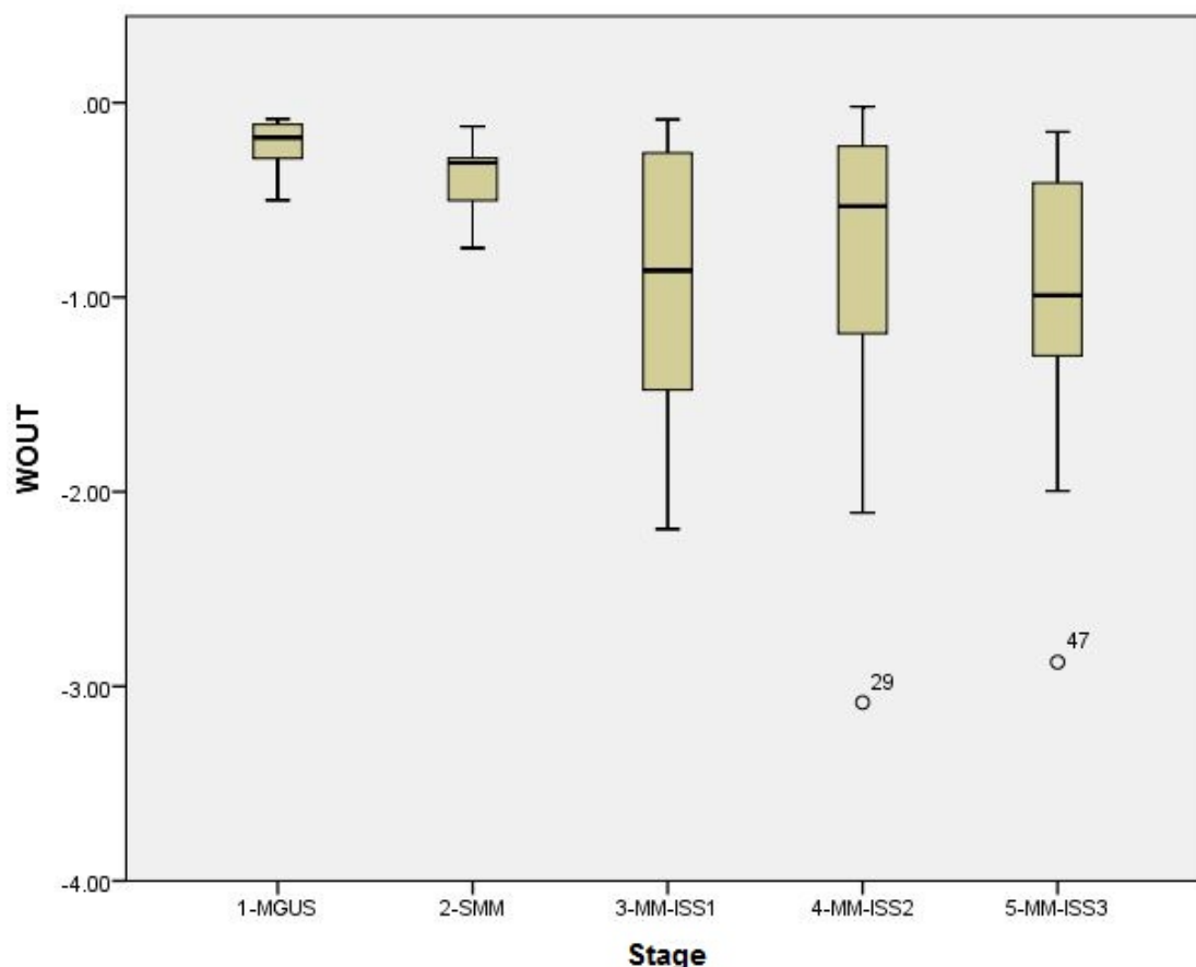
Figure 6.5 Θηκόγραμμα WOUT με Στάδιο ασθένειας
