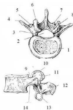
Figure 2.2 Ανατομία του οσφυϊκού σπονδύλου
