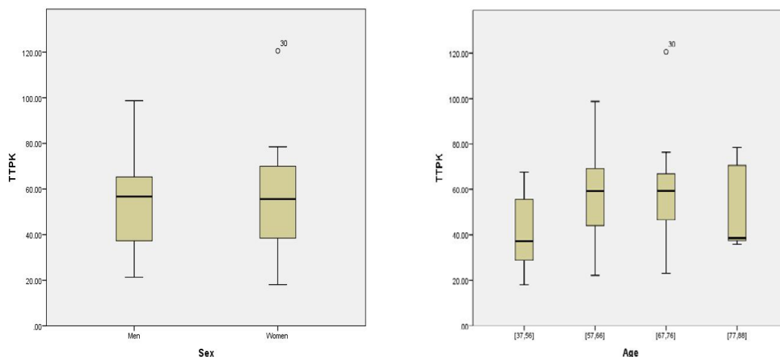
Figure 6.15 Θηκογράμματα TTPK με Φύλο και Ηλικία
