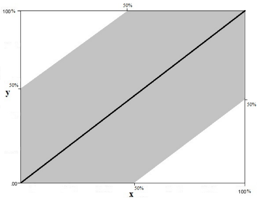
Figure 7.8 Περιοχή πιθανότερης εύρεσης σημείων ( r = 0.5 )
