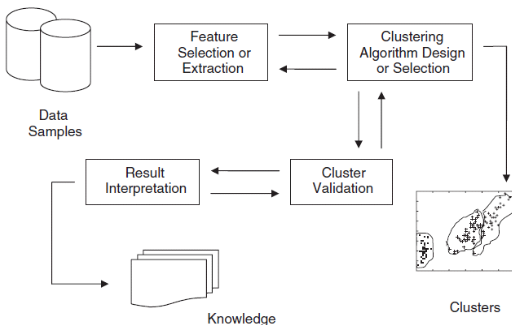
Σχήμα 3.4 Ένα γενικό σχηματικό διάγραμμα Συσταδοποίησης
