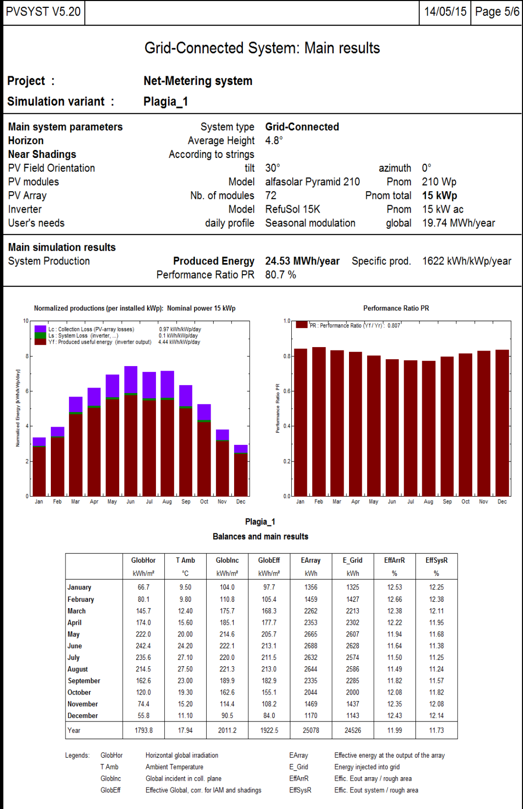
Εικόνα 5.43: Σελίδα 5 της αναφοράς της προσομοίωσης του λογισμικού PVSYST.
