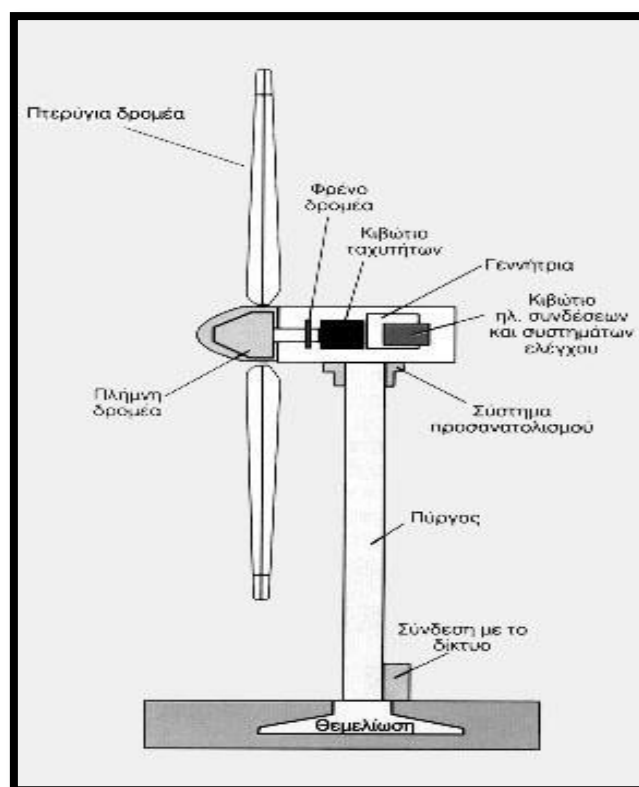
Εικόνα 2.5: Ανεμογεννήτρια
