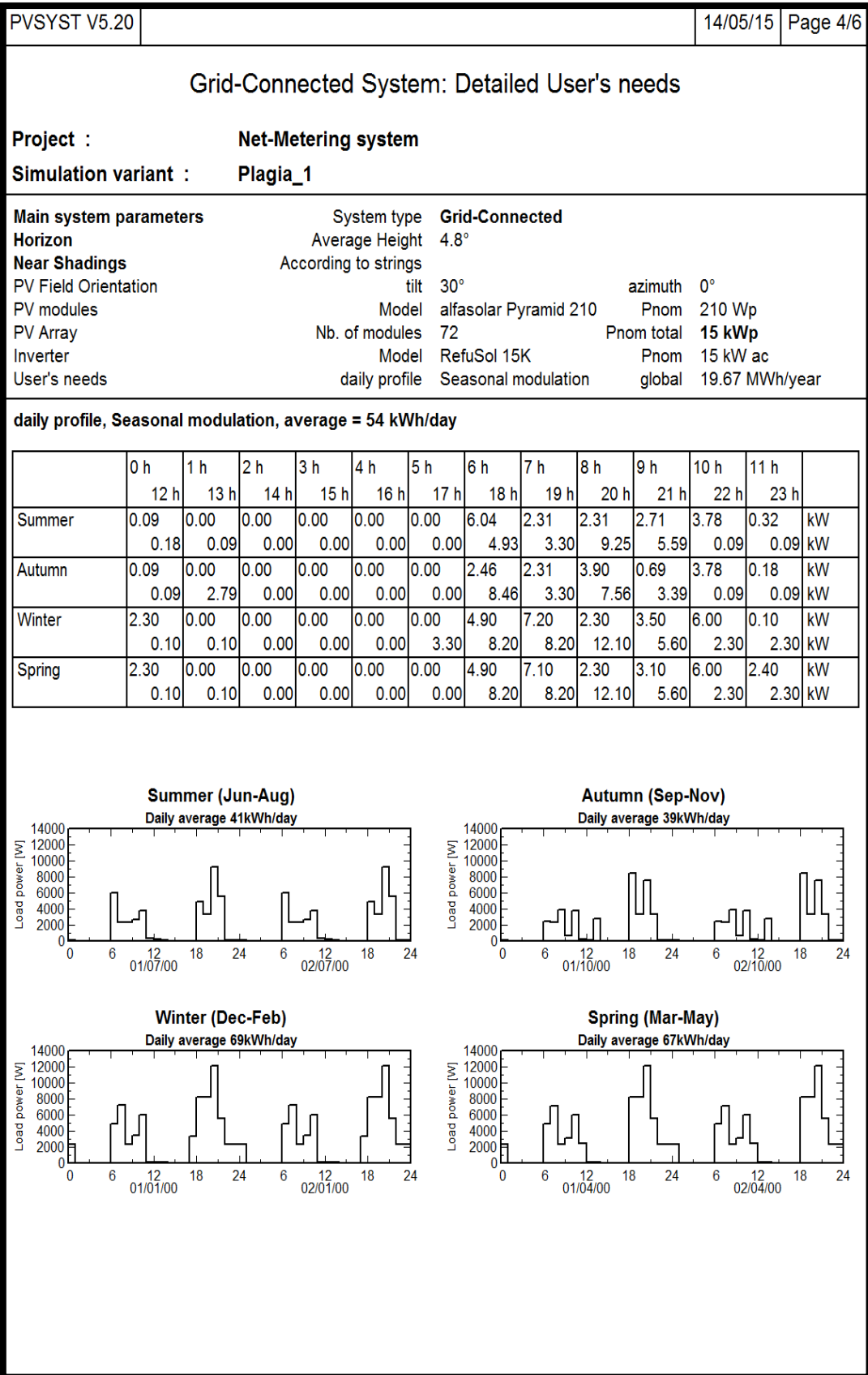
Εικόνα 5.42: Σελίδα 4 της αναφοράς της προσομοίωσης του λογισμικού PVSYST.
