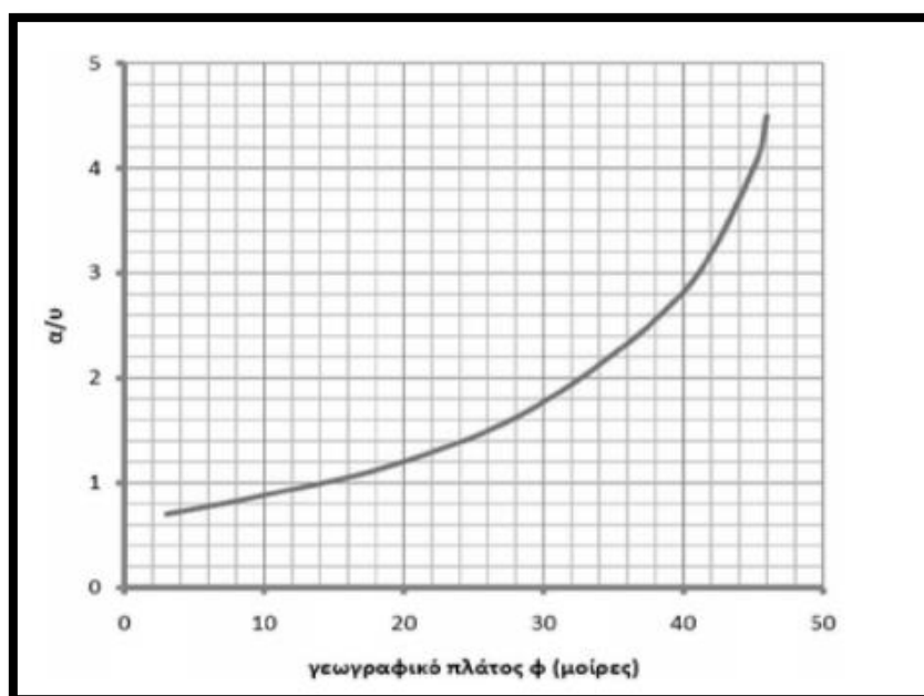
Εικόνα 3.22: Καμπύλη του λόγου \alpha/u σε συνάρτηση με το γεωγραφικό πλάτος \phi του τόπου Πηγή: http://artemis-new.cslab.ece.ntua.gr:8080/jsptui/ [33]
