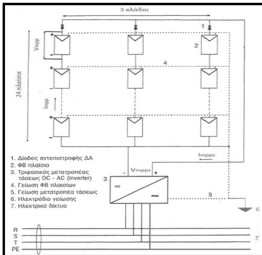
Εικόνα 5.49: Το ΦΒ σύστημα εγκατεστημένης ισχύος 15,1kW p , συνδεδεμένο στο δίκτυο με τον τριφασικό αναστροφέα τάσεως DC-AC.
