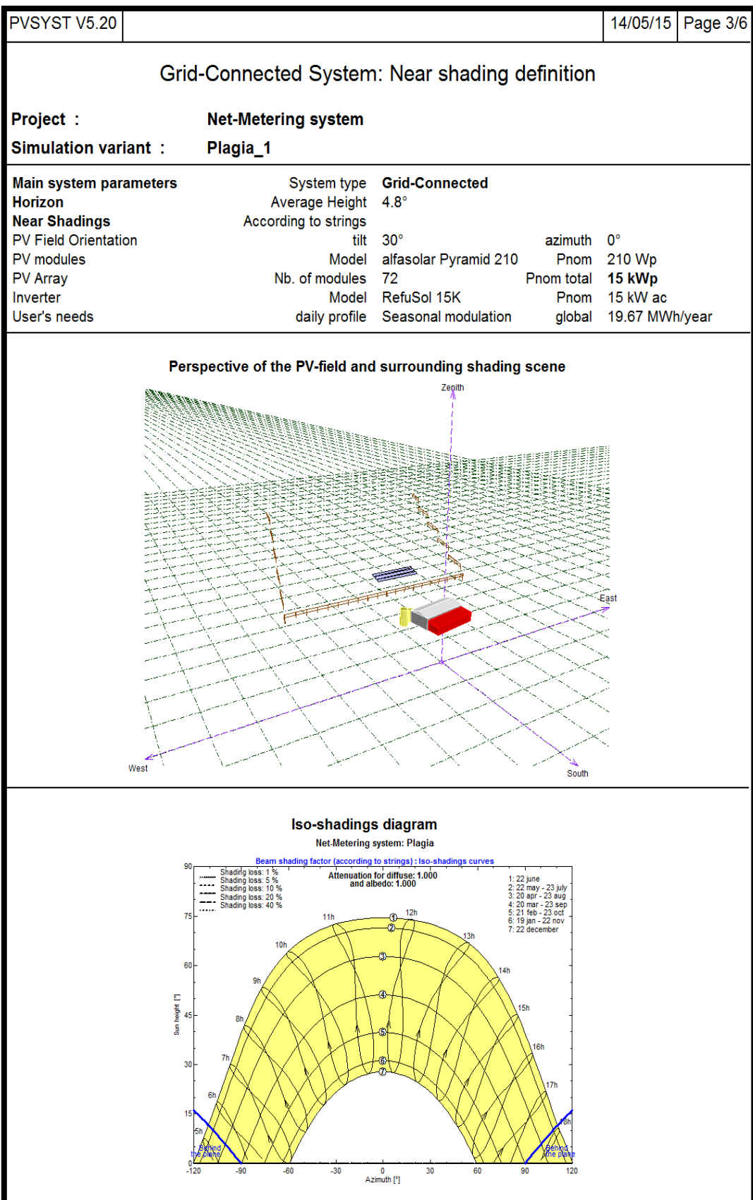
Εικόνα 5.41: Σελίδα 3 της αναφοράς της προσομοίωσης του λογισμικού PVSYST.
