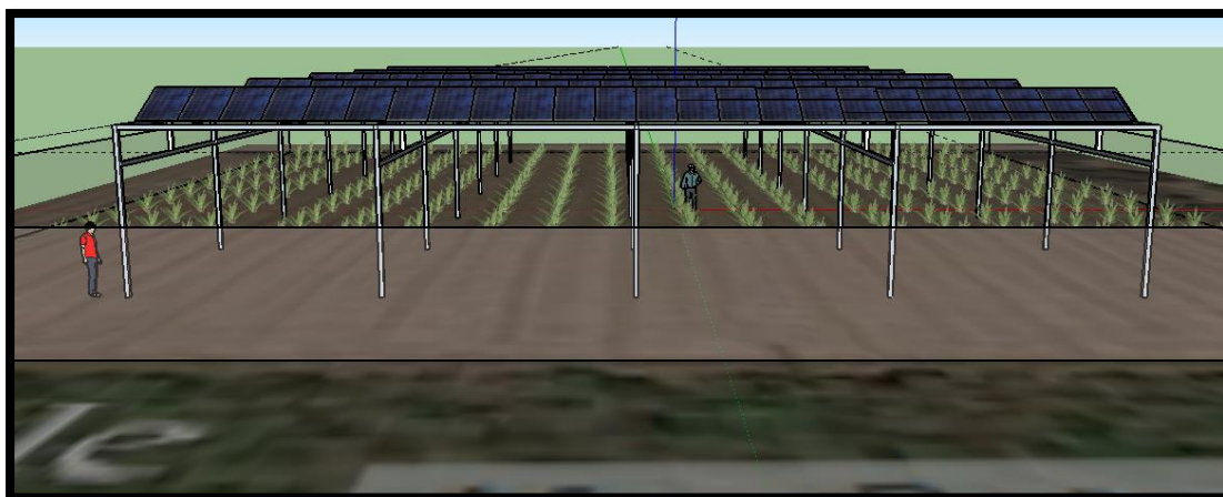
Εικόνα 7.35: Τρισδιάστατη απεικόνιση του ΦΒ συστήματος και της καλλιέργειας switchgrass. Πηγή: Λογισμικό σχεδίασης “Sketcup”.
