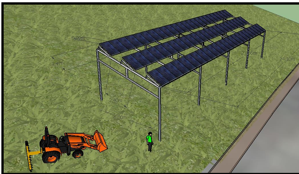
Εικόνα 5.52: Τρισδιάστατη απεικόνιση του ΦΒ συστήματος. Πηγή: Λογισμικό σχεδίασης “Sketcup”.
