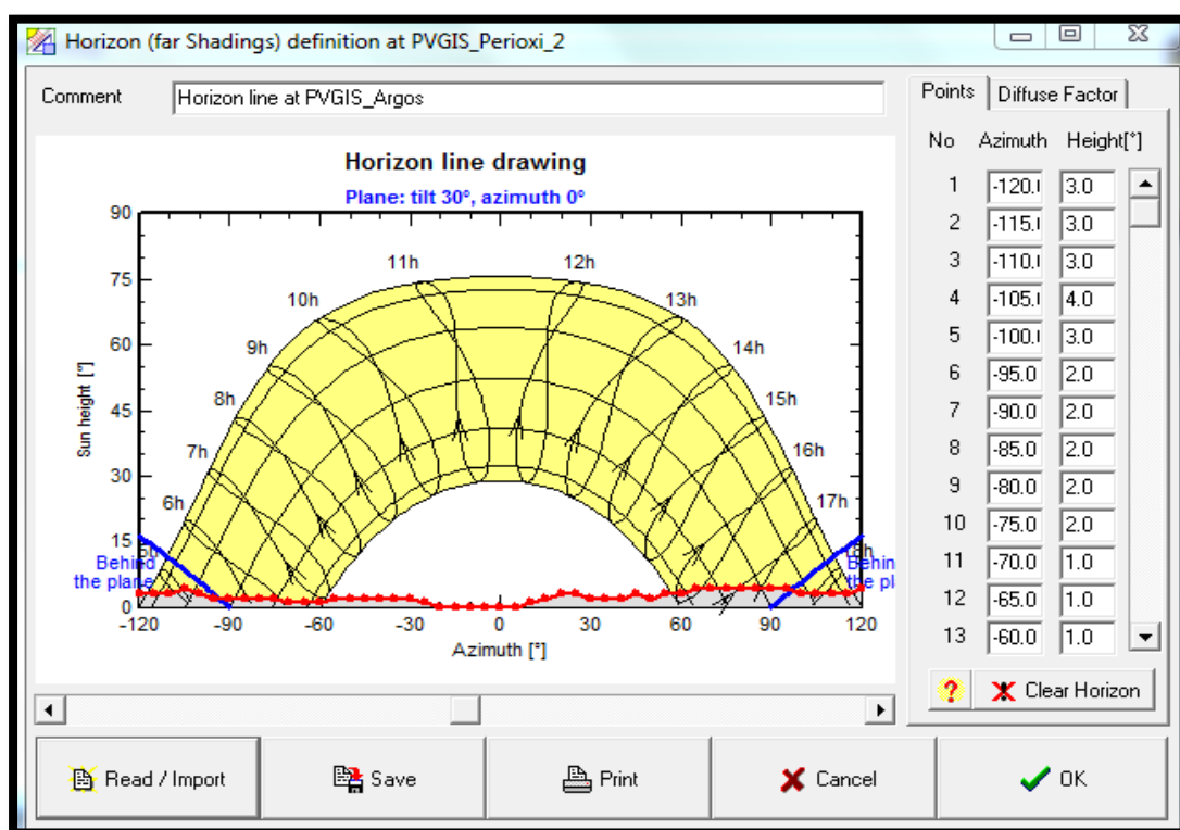
Εικόνα 7.14: Καρτέλα απεικόνισης του πλαισίου “Horizon” του λογισμικού PVSYST.
