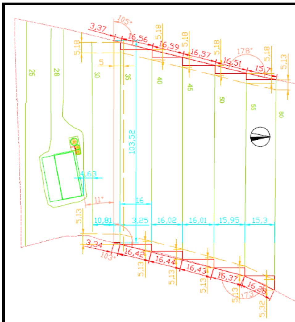
Εικόνα 5.31: Τοπογραφικό διάγραμμα (οριζοντιογραφία) μέρους του οικοπέδου.
