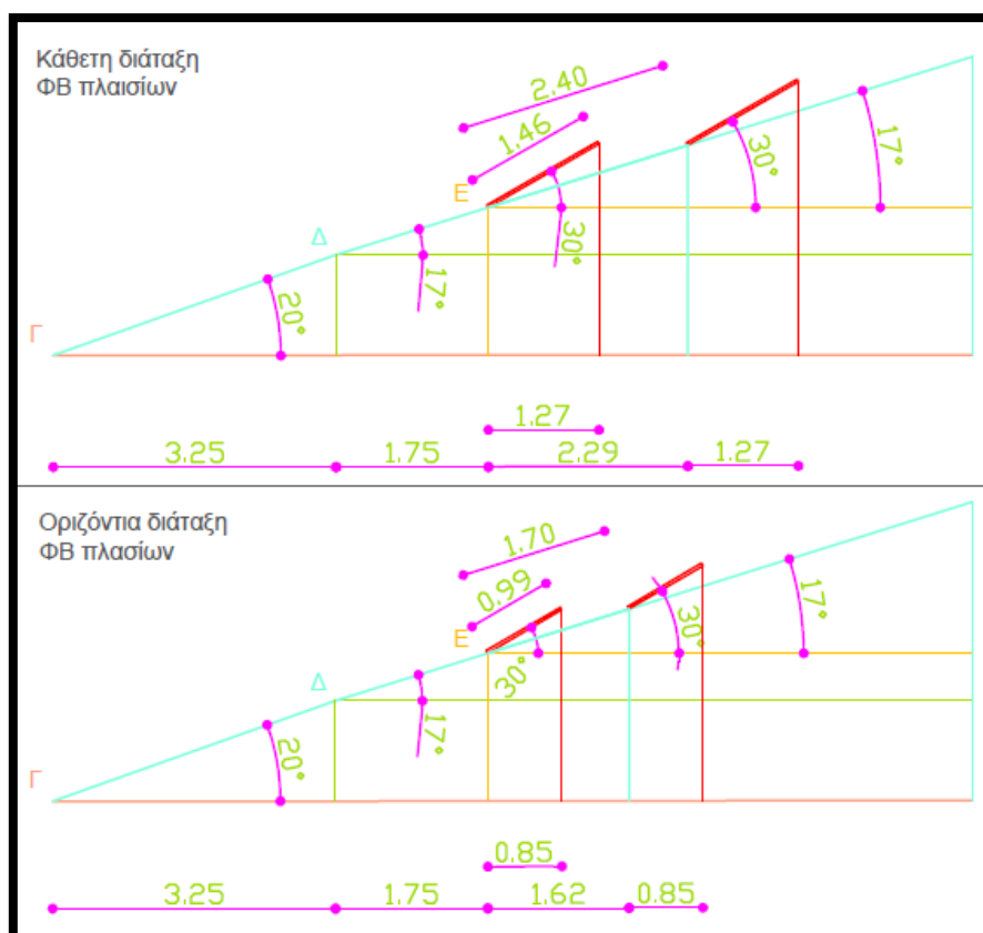
Εικόνα 5.35: Τοπογραφική τομή του εδάφους εγκατάστασης του ΦΒ συστήματος και υπολογισμός της ελάχιστης απόστασης (ε) μεταξύ δύο γειτονικών συστοιχιών, της κλίσης του εδάφους, της κλίσης των ΦΒ πλαισίων και της απόστασης της οριζόντιας προβολής των πλαισίων για κάθετη και οριζόντια διάταξη ΦΒ πλαισίων.
