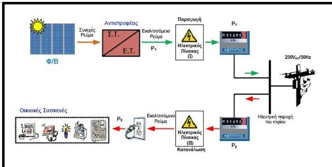
Εικόνα 3.34: Κατανεμημένο φ/β σύστημα συνδεδεμένο στο δίκτυο. Όλη η παραγόμενη ηλεκτρική ενέργεια πωλείται στη ΔΕΗ και όλη η καταναλισκόμενη αγοράζεται από αυτήν.
