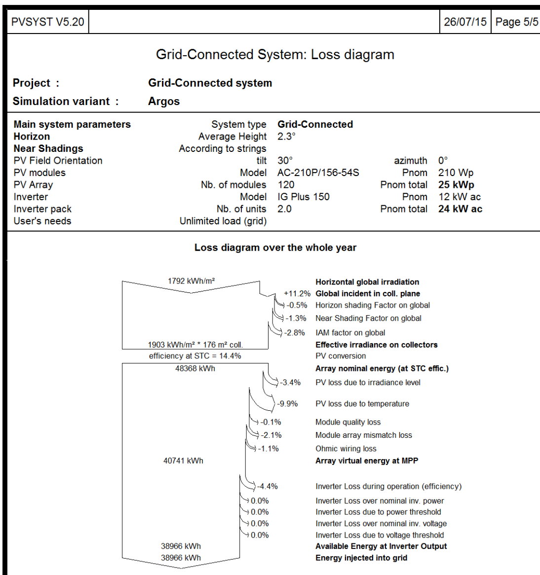
Εικόνα 7.29: Σελίδα 5 της αναφοράς της προσομοίωσης του λογισμικού PVSYST.
