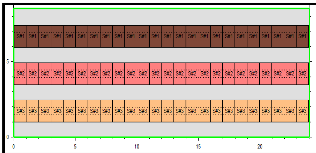
Εικόνα 5.36: Καρτέλα απεικόνισης της επιλογής “Module layout” και αναπαράστασης της χωροθέτησης των ΦΒ πλαισίων σε κάθετη διάταξη. Οι οριζόντιες διακεκομμένες γραμμές συμβολίζουν την παρουσία των διόδων παράκαμψης (3 διόδοι ανά ΦΒ πλαίσιο). Το σύνολο των ΦΒ πλαισίων του ίδιου χρώματος αναπαριστούν μία συστοιχία. Το ΦΒ σύστημα προβάλλεται από γωνία κλίσης 60°.
