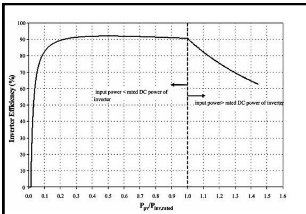
Εικόνα 3.27: Η απόδοση ενός αναστροφέα εξαρτάται από την ισχύ λειτουργίας του
