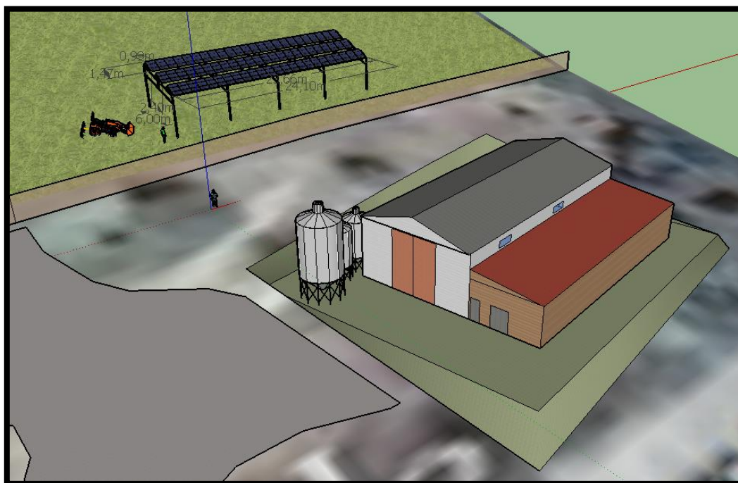
Εικόνα 5.51: Τρισδιάστατη απεικόνιση της κτηνοτροφικής μονάδας και του ΦΒ συστήματος. Πηγή: Λογισμικό σχεδίασης "Sketchup".
