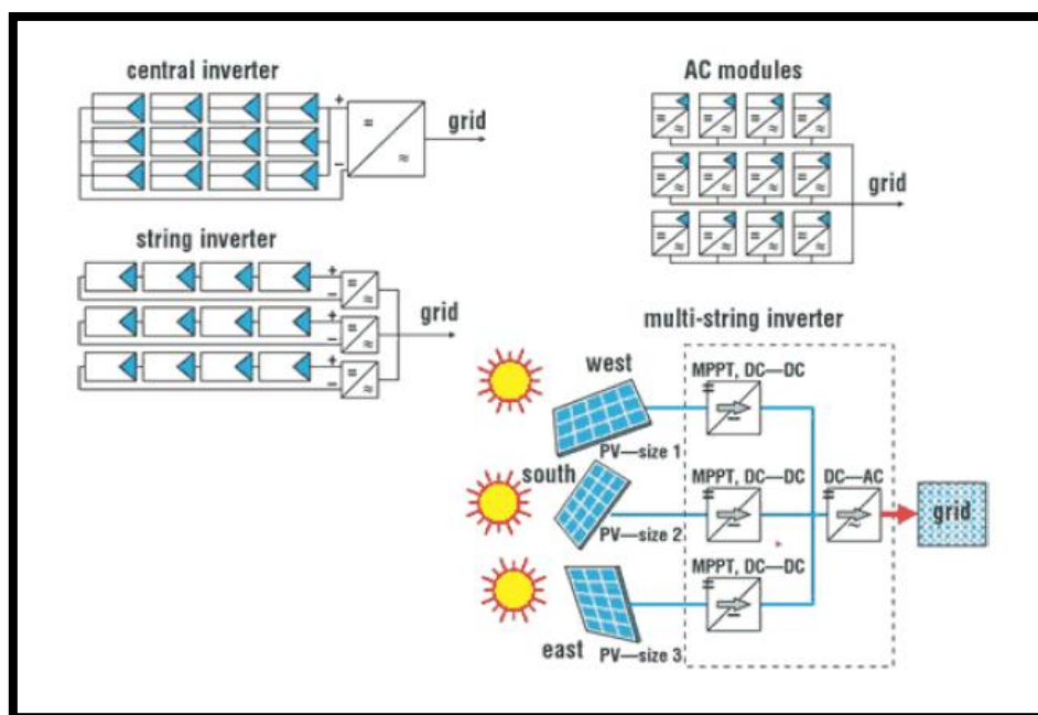
Εικόνα 3.26: Οικογένεια αναστροφών Πηγή: TEE TMK [1]
