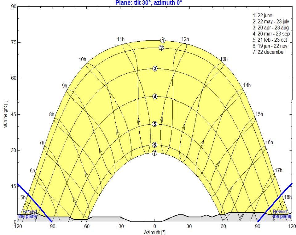
Εικόνα 7.26: Σελίδα 2 της αναφοράς της προσομοίωσης του λογισμικού PVSYST.
