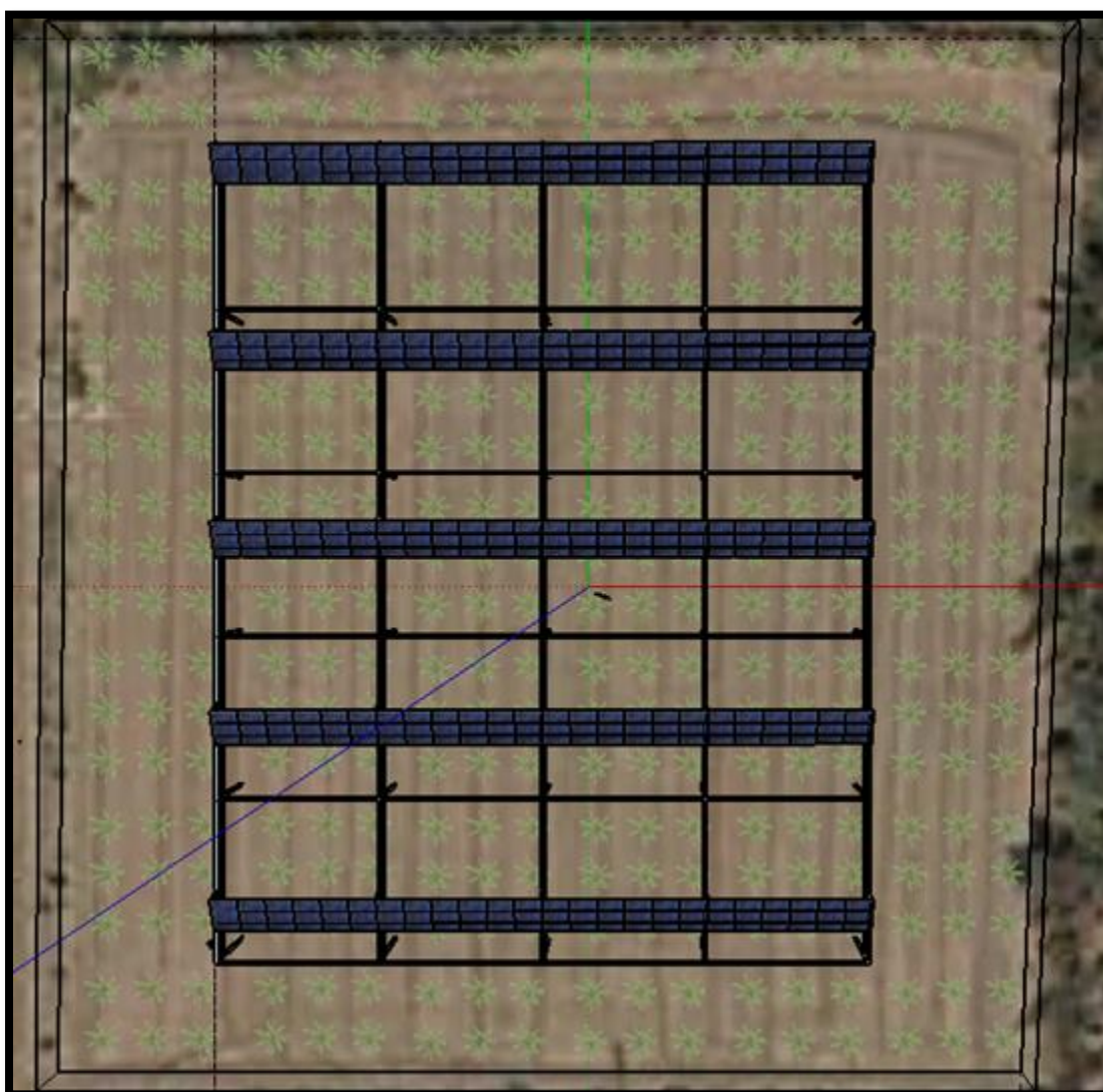
Εικόνα 7.36: Τρισδιάστατη απεικόνιση του ΦΒ συστήματος και της καλλιέργειας switchgrass (κάτοψη). Πηγή: Λογισμικό σχεδίασης “Sketcup”.
