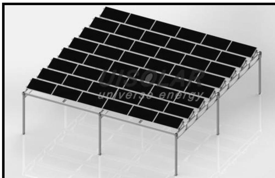
Εικόνα 5.47: Τρισδιάσταση αναπαράσταση του συστήματος στήριξης των ΦΒ πλαισίων.
