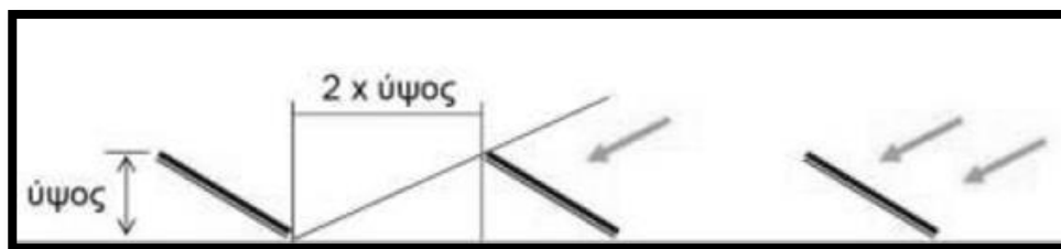
3.25: Χωροθέτηση σειρών πάνελ Πηγή: TEE TMK [1]
