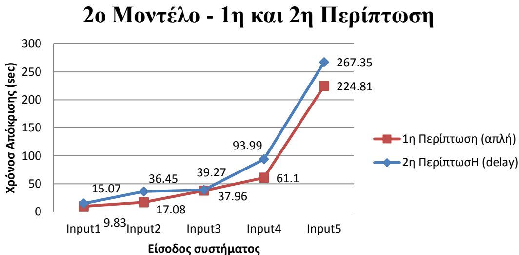
Διάγραμμα 9: Χρονική απόκριση του δευτέρου μοντέλου για κάθε είσοδο, στην πρώτη και την δεύτερη περίπτωση
