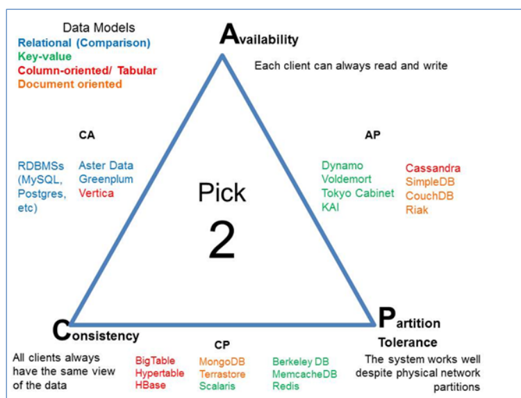
Σχήμα 3.1: CAP Theorem
