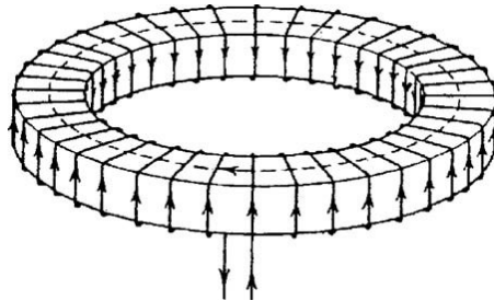
Σχήμα 15: Κατάλληλη τοροειδής μορφή υπεραγωγίου πηνίου για την διατήρηση του μαγνητικού πεδίου στο εσωτερικό του. [18]
