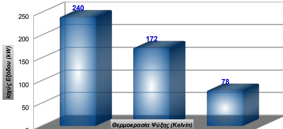
Σχήμα 29: Η ισχύς εξόδου της SDCHM του NSWC με HTS πηνία, που δοκιμάστηκε το 1998 στις ΗΠΑ, σε συνάρτηση με την θερμοκρασία ψύξης του υπεραγωγού. [31]
