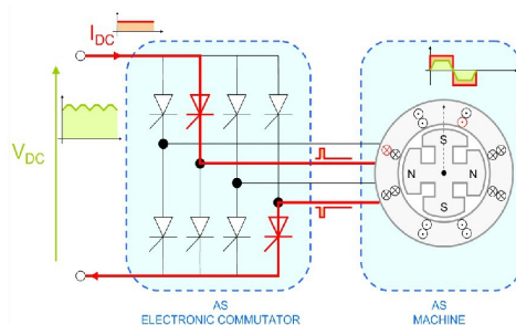
Σχήμα 18: Σύνδεση των θυρίστορ με τον στάτη τετραφασικής μηχανής για έλεγχο του ρεύματος στα τυλίγματα. [19]
