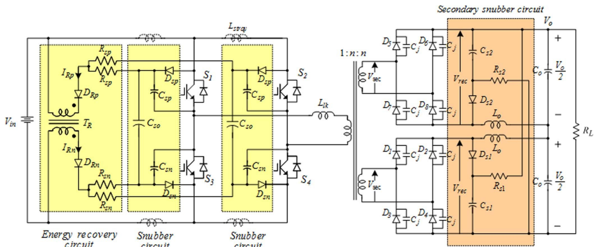
Σχήμα 9: Η τοπολογία του DC/DC μετατροπέα που προτείνεται στο [30].
