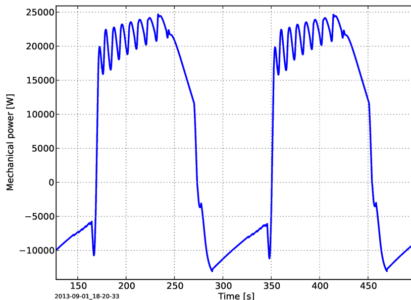
Σχήμα 36: Η μετρούμενη μηχανική ισχύς εξομοίωσης συστήματος τύπου με αλεξίπτωτο πλαγιάς για δύο κύκλους λειτουργίας. [28]
