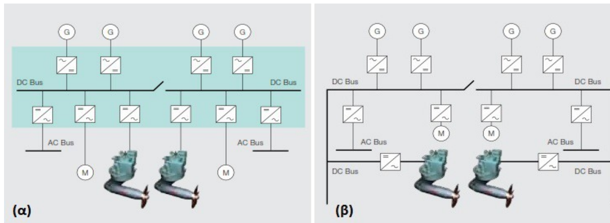
Σχήμα 9: (α) Η multidrive και (β) η κατανομημένη προσέγγιση για το dc δίκτυο της ABB. [5]
