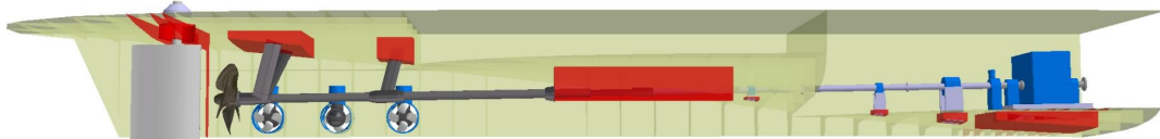
Σχήμα 2: Διάταξη αξονικής ηλεκτροπρόωσης όπου φαίνεται ο ηλεκτροκινητήρας (αριστερά), ο άξονας, οι μηχανικοί σύνδεσμοι και τα στηρίγματα. [3]
