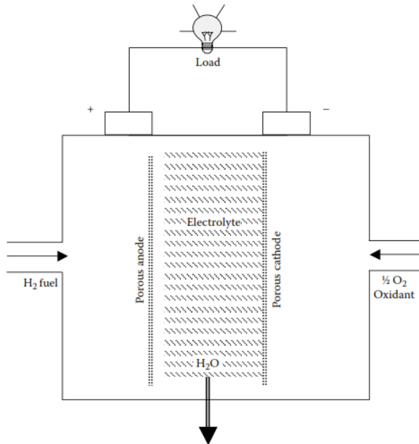
Σχήμα 19: Σχηματική αναπαράσταση των βασικών στοιχείων κυψέλης καυσίμου. [20]
