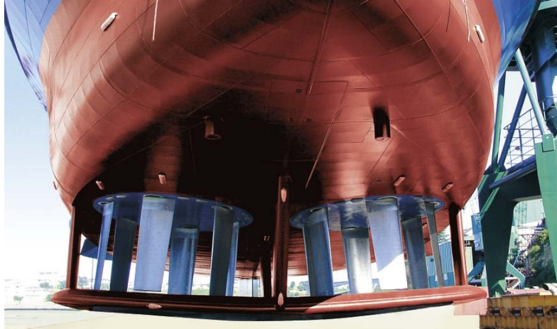
Σχήμα 6: Παράδειγμα εγκατάστασης προπέλας Voith Schneider [7].
