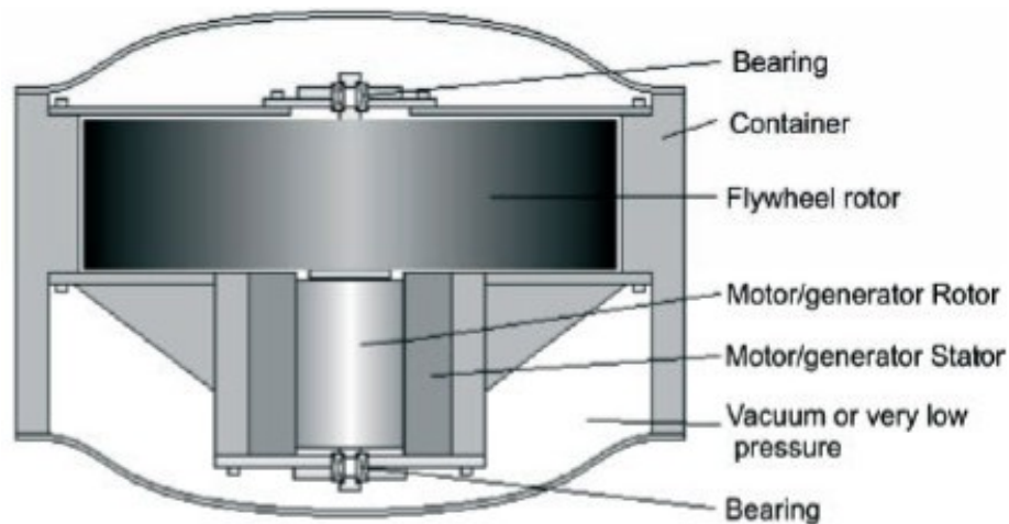
Σχήμα 5: Βασική διάταξη του σφονδύλου.[22]
