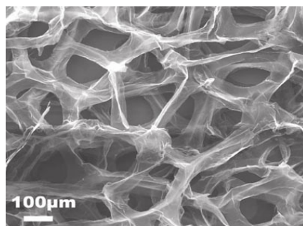
Σχήμα 10: Μεγέθυνση της επιφάνειας φύλλου γραφενίου που χρησιμοποιείται σε υπερπυκνωτή. [24]
