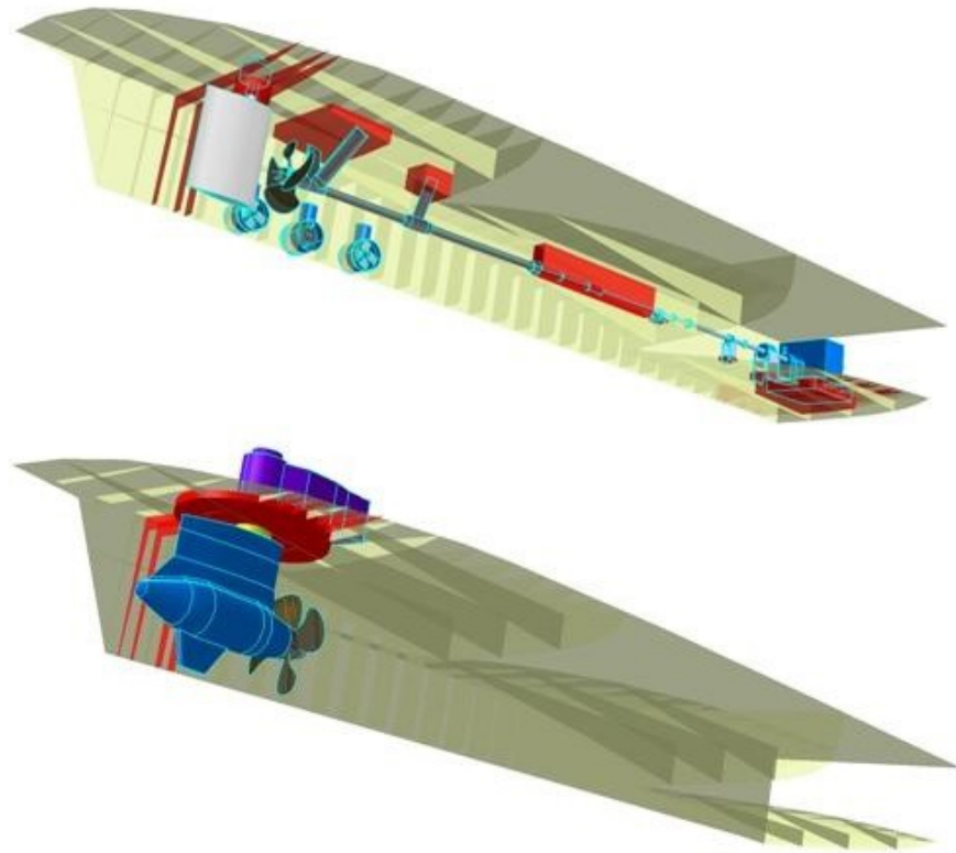
Σχήμα 7: Οπτική απεικόνιση της αξονικής (πάνω) και της rodded ηλεκτρικής πρόωσης για το ίδιο πλοίο. [3]
