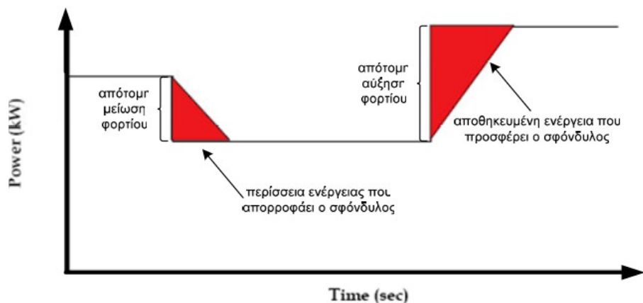
Σχήμα 6: Οι κόκκινες περιοχές δείχνουν τα συμπληρώματα ενέργειας που παρέχονται από το σφόνδυλο. [22]
