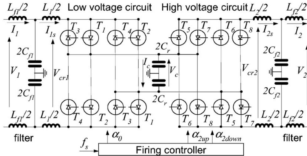
Σχήμα 6: Παράδειγμα DC/DC μετατροπέα αμφίδρομου συντονισμού με αμφίδρομα θυρίστορ. [21]
