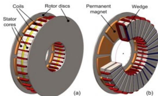
Σχήμα 15: Σχηματικό διάγραμμα μηχανής μόνιμου μαγνήτη με αξονικό μαγνητικό πεδίο (a) τελική σύνθεση, (b) το εσωτερικό μετά την απομάκρυνση ενός ρότορα-δίσκου και μερικών τμημάτων στάτορα και πηνίων. [13]
