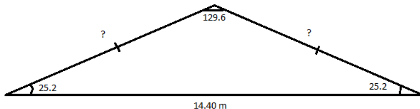
Εικόνα 5.6 : Πλάγια όψη στέγης για υπολογισμό των κεκλιμένων επιφανειών.
