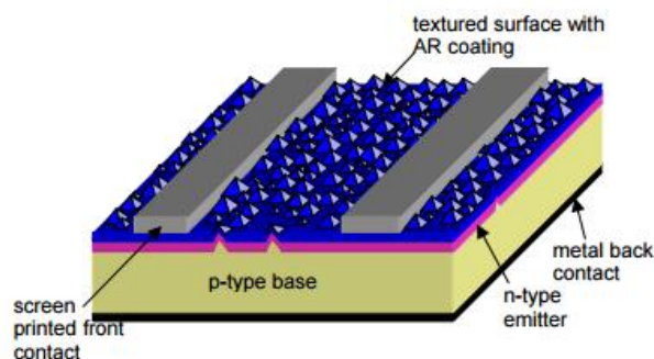
Εικόνα 3.10 : Σχηματική αναπαράσταση ενός τυπικού μονοκρυσταλλικού ηλιακού στοιχείου.
