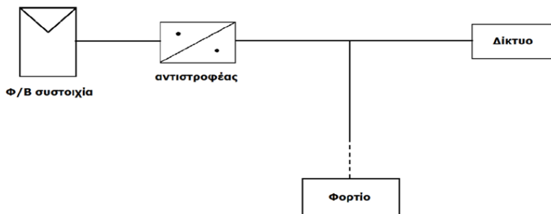
Εικόνα 3.14 : Τοπολογία διασυνδεδεμένου ΦΒ συστήματος.
