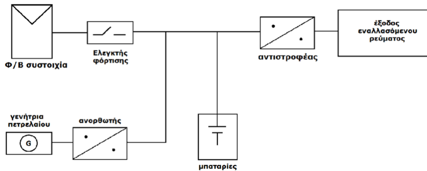
Εικόνα 3.16 : Τοπολογία υβριδικού ΦΒ συστήματος.
