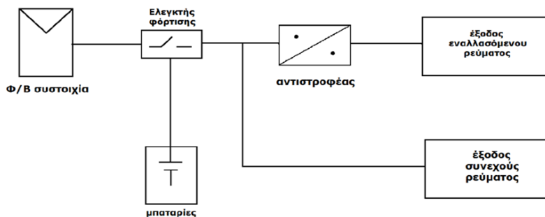
Εικόνα 3.15 : Τοπολογία αυτόνομου ΦΒ συστήματος.
