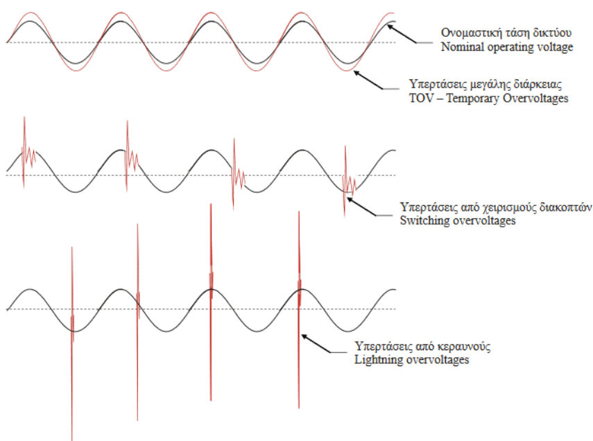
Εικόνα 4.5 : Μορφές υπερτάσεων.
