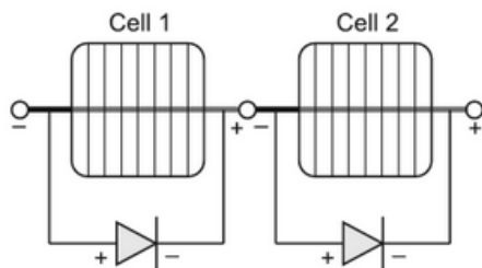
Εικόνα 4.1 : Δίοδος αντεπιστροφής συνδεόμενη παράλληλα και με αντίστροφη πολικότητα με το ΦΒ κελί.
