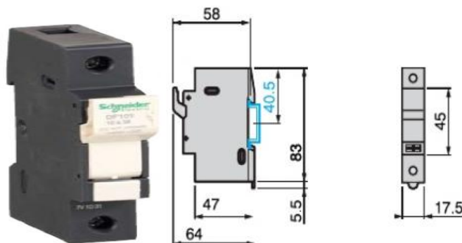
Εικόνα 4.11 : Ασφάλεια Tesys DF101PV.
