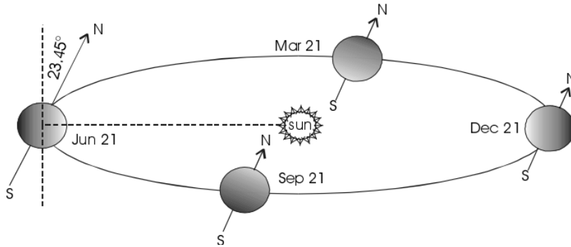
Εικόνα 2.2 : Η τροχιά της γης και η απόκλιση της σε διάφορες χρονικές τιμές του χρόνου.
