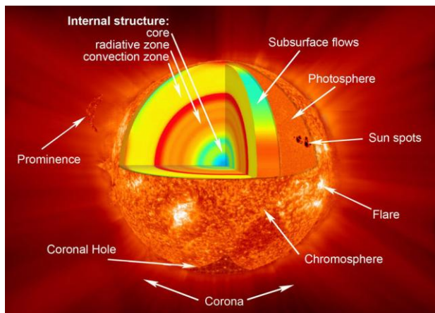
Εικόνα 2.1 : Περιοχές του ηλίου.
