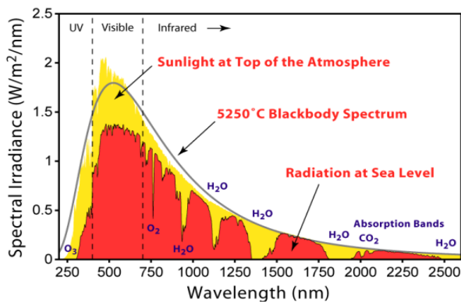
Εικόνα 2.4 : Φάσμα ηλιακής ενέργειας.
