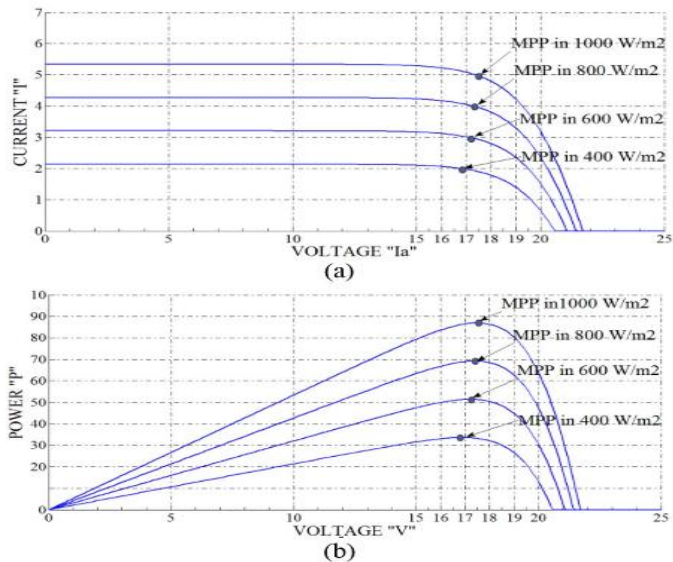
Εικόνα 3.20 : Χαρακτηριστικά εξόδου ΦΒ πλαισίου το οποίο εκτίθεται σε κανονικές συνθήκες : (α) Χαρακτηριστικές ρεύματος-τάσης I-V και (β) χαρακτηριστικές ισχύος-τάσης P-V.
