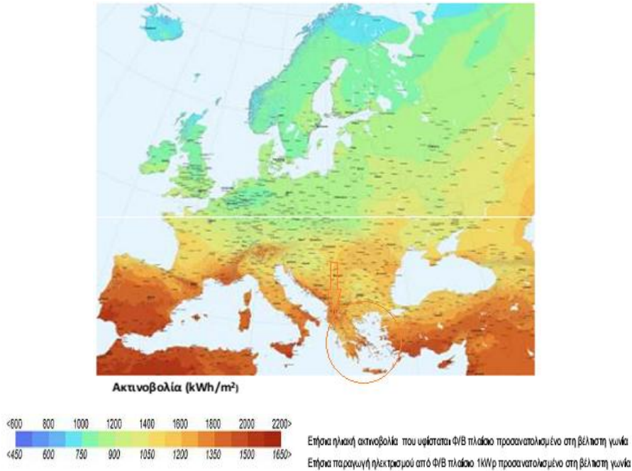
Εικόνα 2.7 : Ετήσιο ηλιακό ηλεκτρικό δυναμικό στην Ευρώπη.
