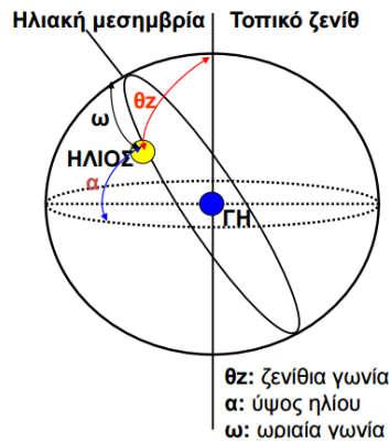
Εικόνα 2.6 : Ζενίθια γωνία, ύψος ηλίου, ωριαία γωνία.
