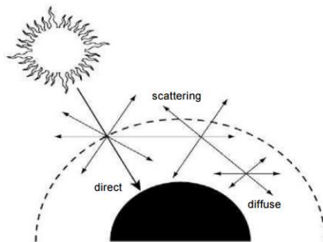
Εικόνα 2.5 : Σκέδαση στην ατμόσφαιρα, οδηγεί σε διάχυτη ακτινοβολία.
