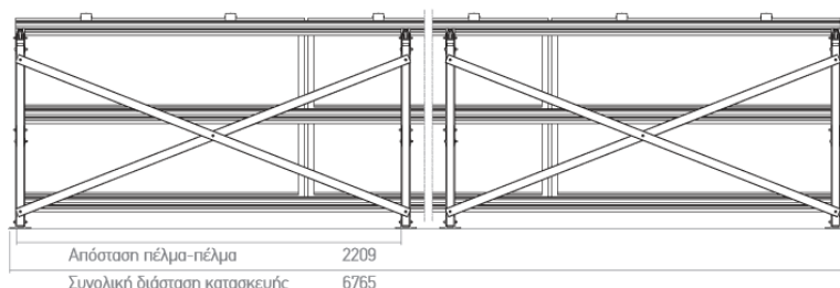
Εικόνα 3.18 : Πίσω όψη συστήματος στήριξης ΦΒ παλίσίων σε επίπεδες οροφές της εταιρείας Aluminco.
