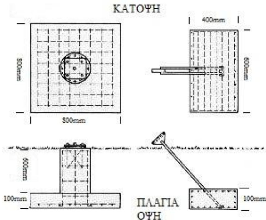
Σχήμα 6.6. Κατόψεις και πλάγιες όψεις των σημείων όπου θα τοποθετηθεί οπλισμένο σκυρόδεμα
