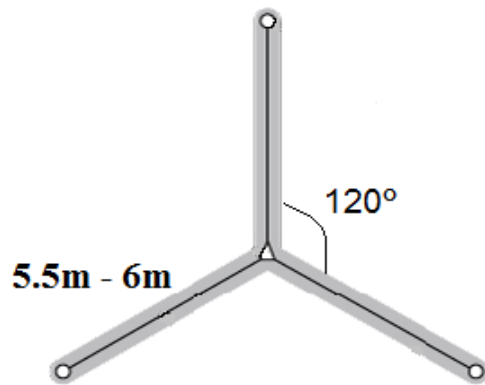
Σχήμα 6.5. Κάτοψη στήριξης πυλώνα ανεμογεννήτριας
