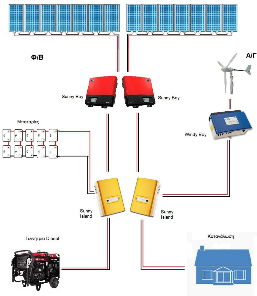
Σχήμα 5.8. Διάγραμμα του υβριδικού φ/β συστήματός μας
