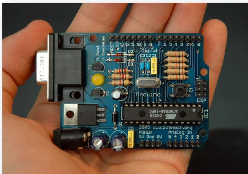
Εικόνα 1: Μικροελεγκτής Arduino
