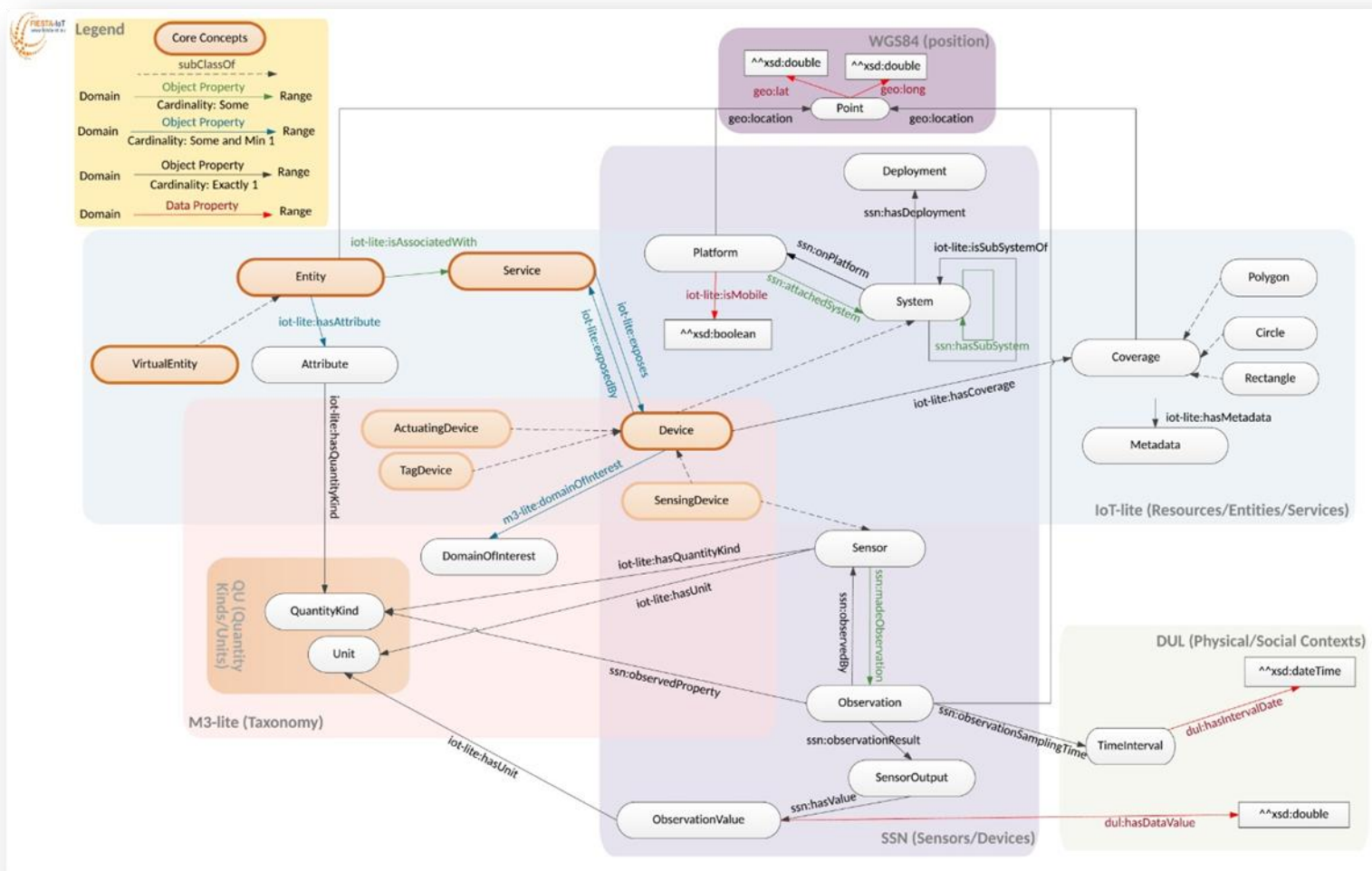
Σχήμα 26: Βασικός γράφος της Fiesta-IoT οντολογίας
