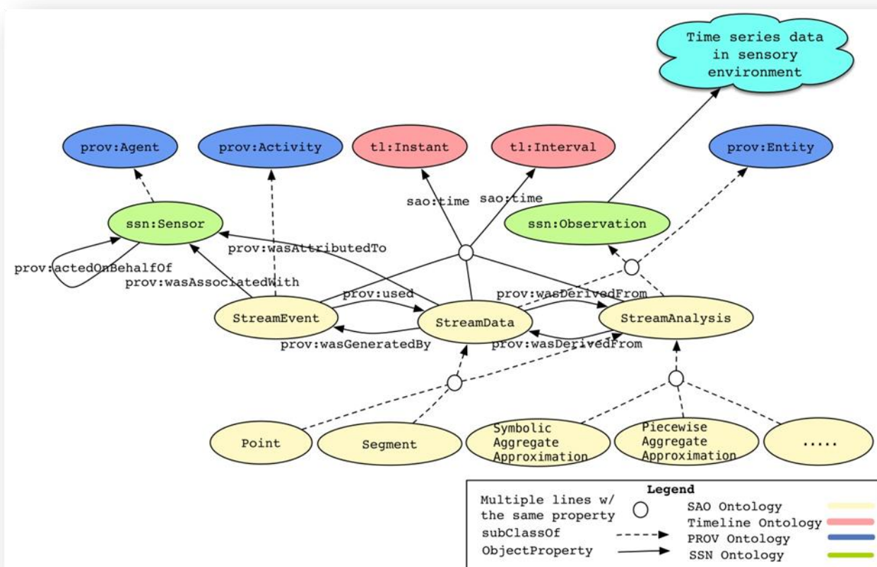
Σχήμα 29: Βασικοί γράφοι της Stream Annotation οντολογίας
