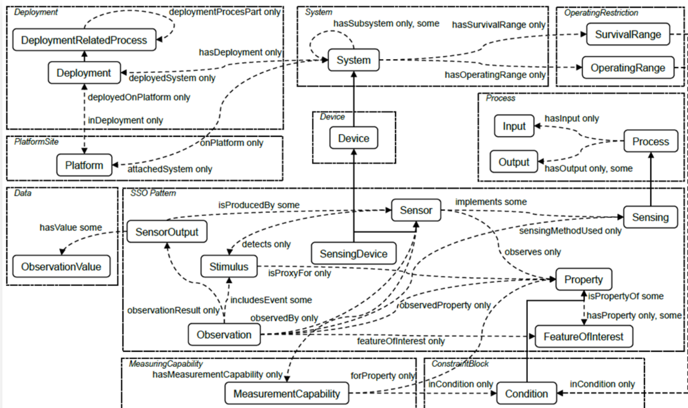
Σχήμα 35: Βασικές κλάσεις και ιδιότητες της SSN
