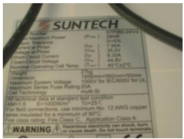
Φωτογραφία 4: Πινακίδα στοιχείων Φ/Β πάνελ
