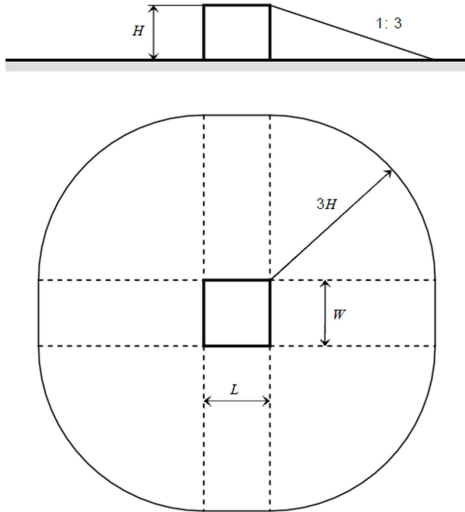
Διάγραμμα κατασκευής της ισοδύναμης επιφάνειας
