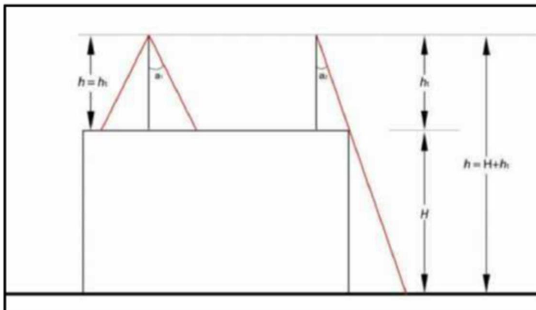
Σχήμα 2 Καθορισμός του ύψους h σύμφωνα με τη μέθοδο της γωνίας προστάσιας.
