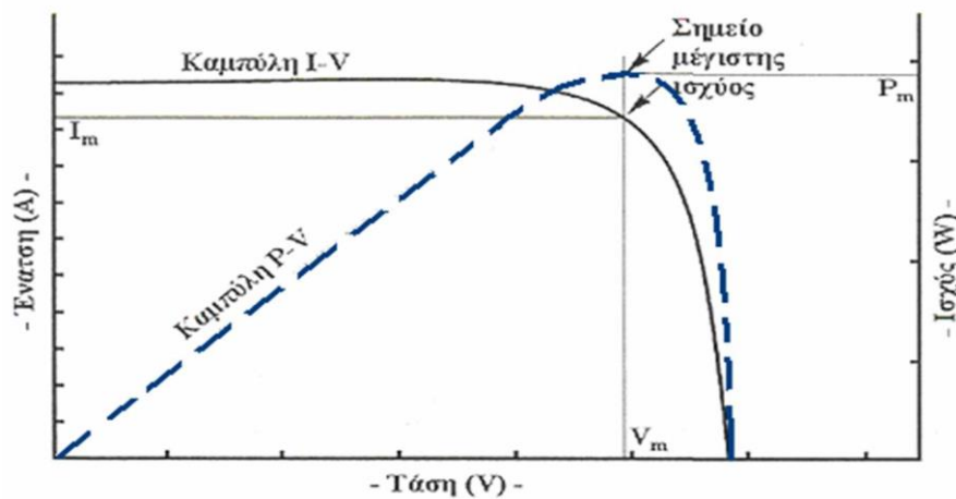
I-V χαρακτηριστική του \Phi/B κυττάρου
