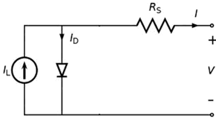
Τελικό ισοδύναμο κύκλωμα \Phi/B κυττάρου
