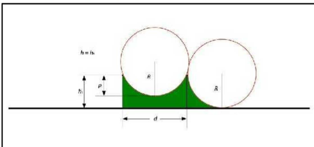
Ζώνη προστασίας δύο παράλληλων τεταμένων συρμάτων.
