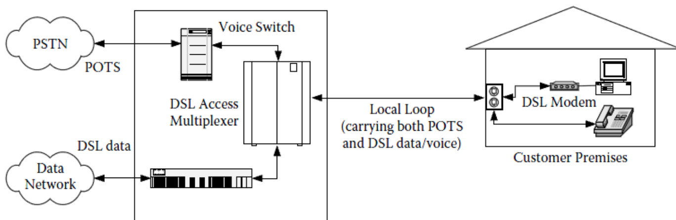
Σχήμα 1.1.1 Σχηματική αναπαράσταση τοπολογίας παροχής τηλεφωνικών και ευρυζωνικών υπηρεσιών
