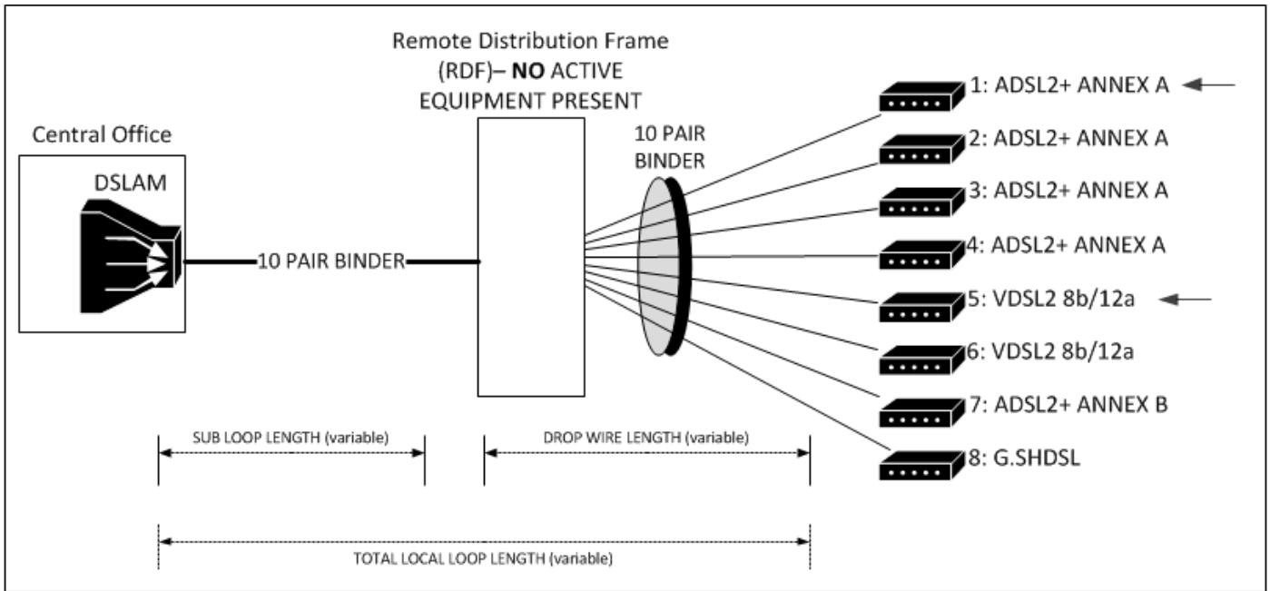
Σχήμα 4.1.4 Αρχιτεκτονική Σεναρίου 1 – Υποσενάριο 2 (VDSL2 στο AK)
