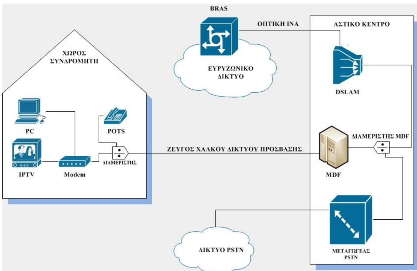
Σχήμα 1.3.3 Παροχή ευρυζωνικών υπηρεσιών μέσω δικτύου χαλκού
