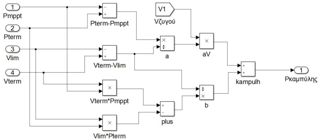
Εικόνα 6.3 : Υλοποίηση της καμπύλης droop στο Matlab/Simulink.
