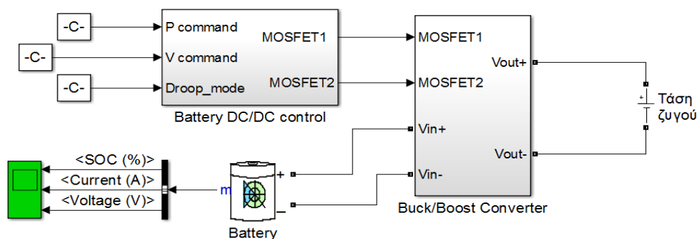
Εικόνα 3.6 : Η μπαταρία στο Matlab/Simulink.
