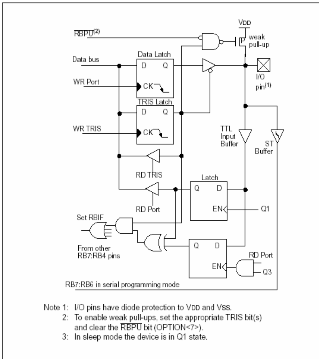
Σχήμα 4.22 Ακροδέκτες RB7:RB4 μονάδας εισόδου/ εξόδου (I/O) PORT B
