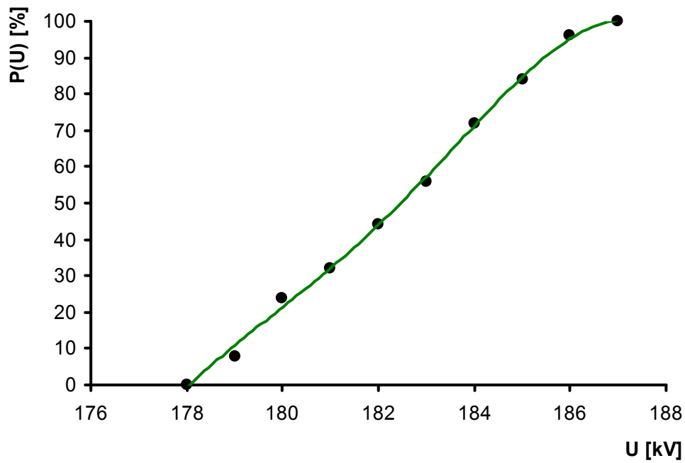
Σχήμα 6.15: Εύρεση της U_{50} ( d=30cm , r=1mm Φ22, \varphi=8g/m^3 )
