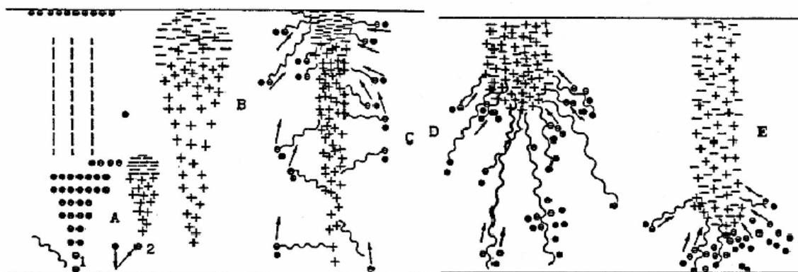
Σχήμα 2.3: Σχηματισμός του θετικού streamer. A: εκκίνηση της αρχικής στοιβάδας, B: η αρχική στοιβάδα φθάνει στην άνοδο, C: θετικό φορτίο εκκινά ένα streamer, D,E: πρόοδος του streamer
