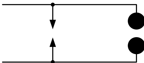
Σχήμα 2.15: Διάκενα ανομοιογενούς και ομοιογενούς πεδίου εν παραλλήλω
