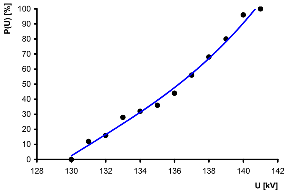
Σχήμα 6.7: Εύρεση της U_{50} ( d=20cm , r=1mm Φ16, \varphi=11g/m^3 )
