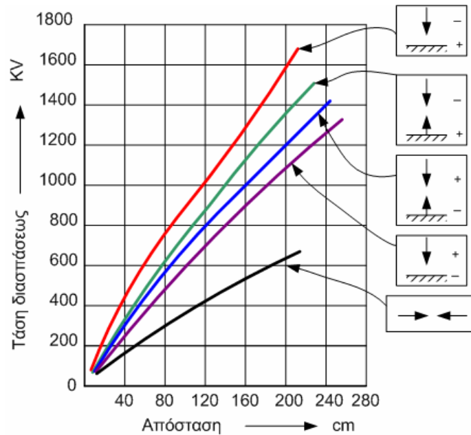
Σχήμα 2.20: Αντοχή διαφόρων διατάξεων υπό κρουστικές τάσεις 1,5/40\mu s σε 20^{\circ}C , 760mmHg και 11g/m^3 υγρασίας. Προς σύγκριση δίνεται και η καμπύλη διάσπασης (μαύρη γραμμή) διάταξης δύο ακίδων υπό τάση 50kV .
