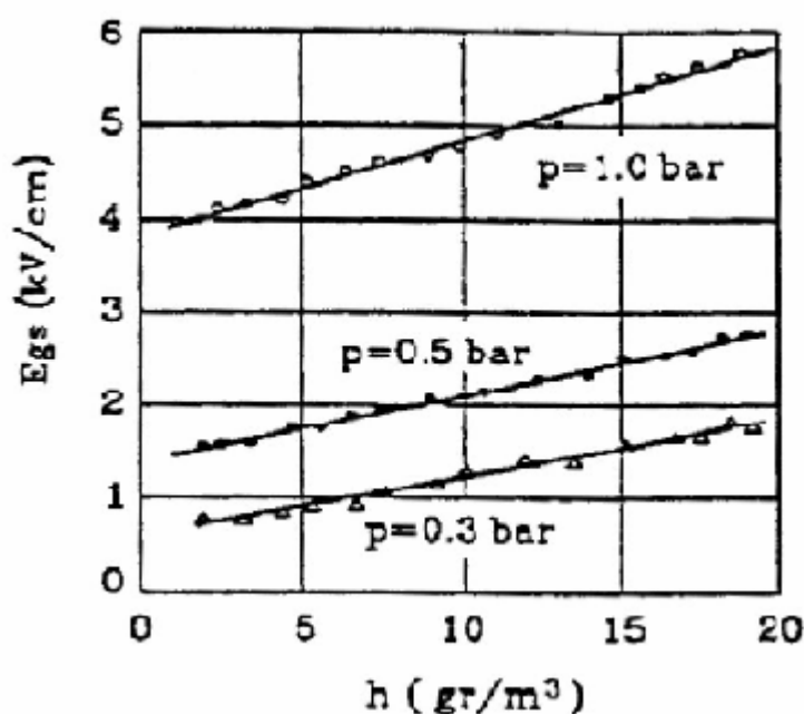
Σχήμα 2.12: Κρίσιμο πεδίο των streamers συναρτήσει της απόλυτης υγρασίας για τρεις τιμές της πίεσης
