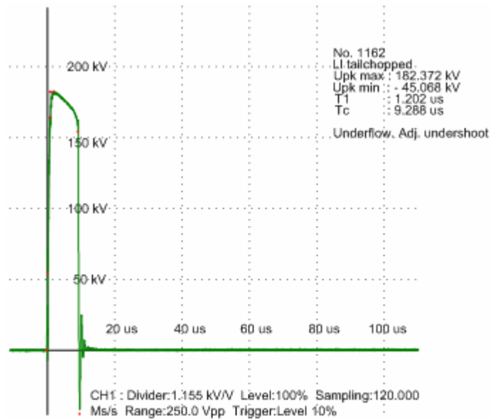
Σχήμα 6.6: Διάσπαση δοκιμίου
