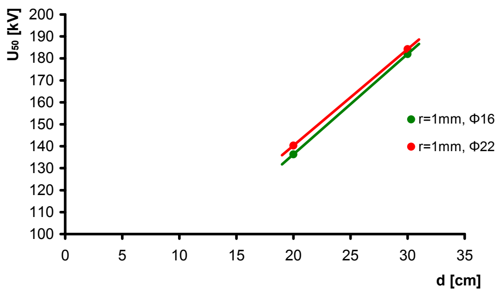
Σχήμα 6.11: Μεταβολή της U_{50} συναρτήσει του διακένου d του σπινθηριστή (r=1mm,Φ16 και r=1mm,Φ22)
