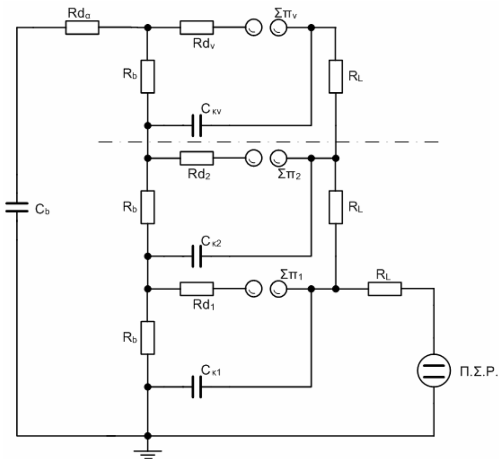
Σχήμα 5.1: Συνδεσμολογία n βαθμίδων της γεννήτριας κρουστικών τάσεων
