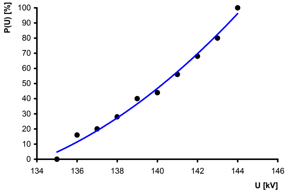
Σχήμα 6.8: Εύρεση της U_{50} ( d=20\text{cm} , r=1\text{mm} Φ22, \varphi=11\text{g/m}^3 )
