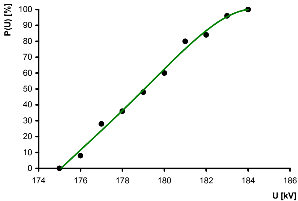
Σχήμα 6.14: Εύρεση της U_{50} ( d=30cm , r=1mm Φ22, \phi=6g/m^3 )
