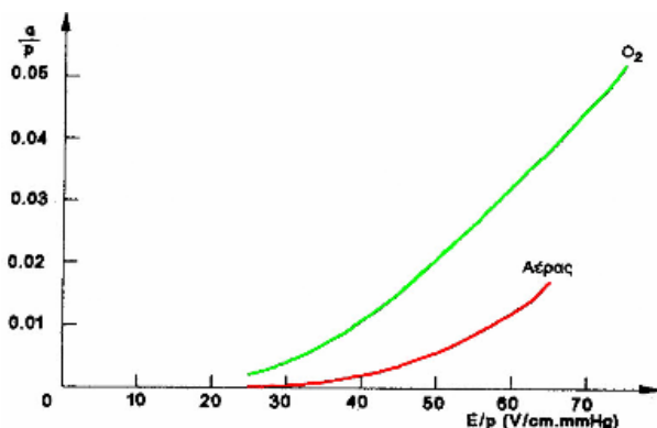
Σχήμα 2.2: Καμπύλη του Sanders
