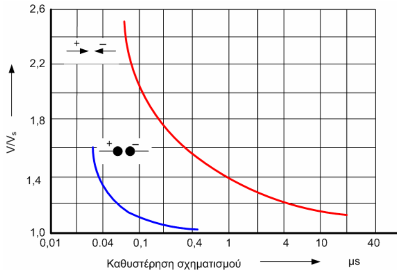
Σχήμα 2.16: Καθυστέρηση σχηματισμού μεταξύ των ηλεκτροδίων σε απόσταση 3cm
