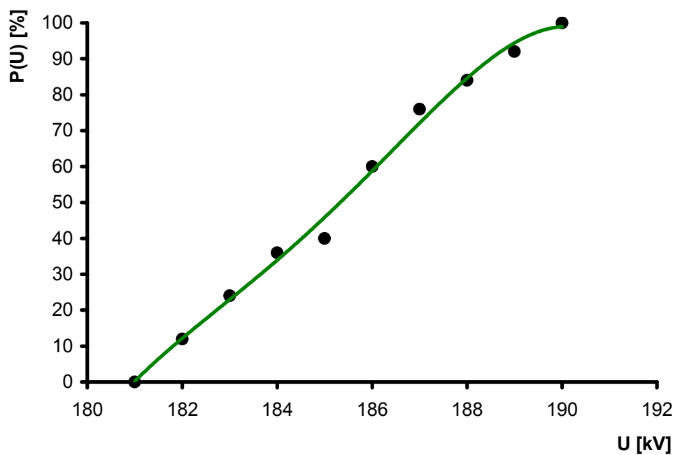
Σχήμα 6.16: Εύρεση της U_{50} ( d=30cm , r=1mm Φ22, \varphi=15g/m^3 )
