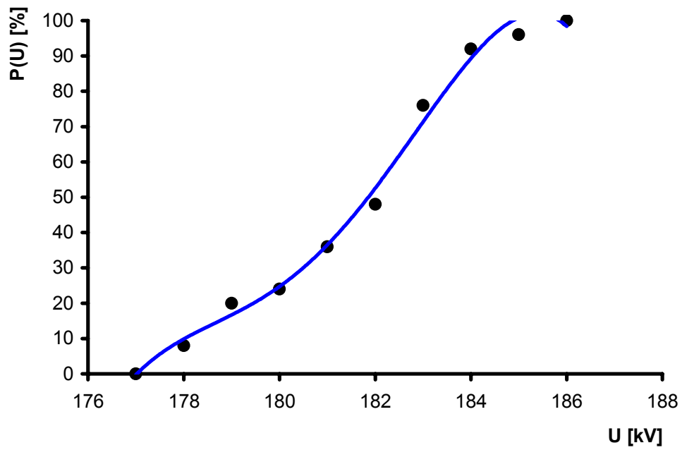
Σχήμα 6.9: Εύρεση της U_{50} ( d=30\text{cm} , r=1\text{mm} Φ16, \varphi=11\text{g/m}^3 )
