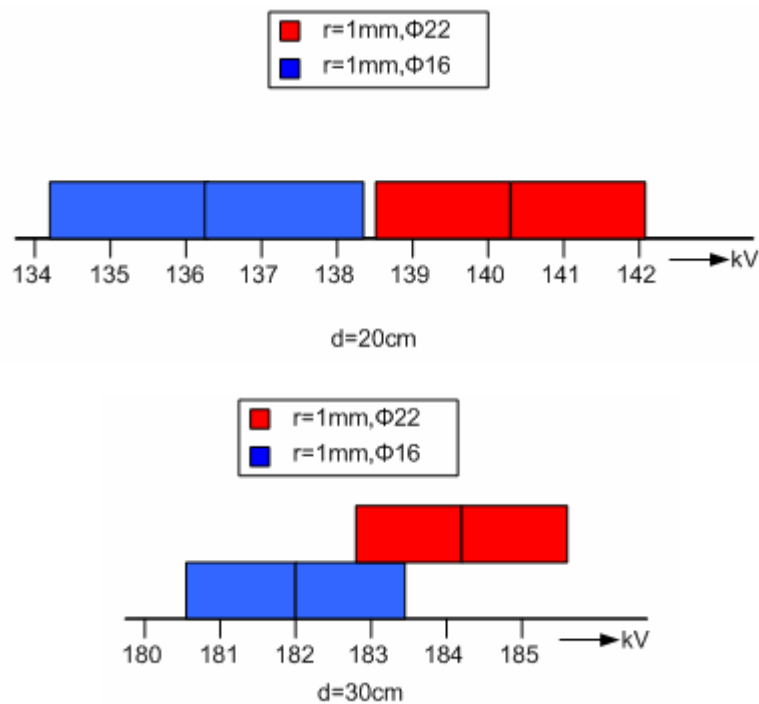
Σχήμα 6.13: Περιοχές αξιοπιστίας 95% των τάσεων διάσπασης U_{50} του πίνακα 6.1 για μήκος διακένου 20cm και 30cm.
