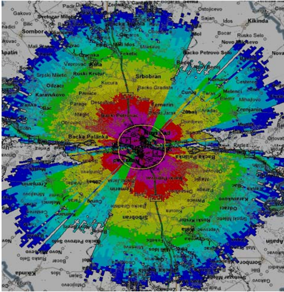
Υπόδειγμα χάρτη κάλυψης μίας κεραίας κινητής τηλεφωνίας. Οι βυθίσεις οφείλονται στην μορφολογία του εδάφους
