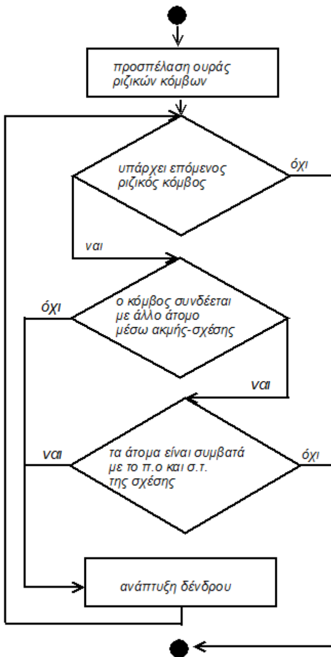
εκτέλεση αλγορίθμου tableau
