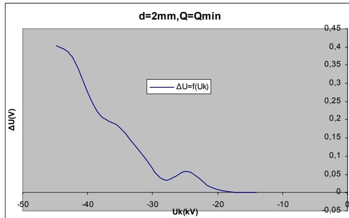
Σχήμα Β 2.12.1 Μεταβολή Άλματος Δυναμικού σε συνάρτηση με την Κρουστική Τάση
