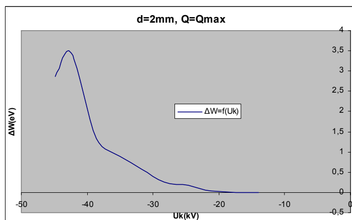
Σχήμα Β 2.11.3 Μεταβολή Ενέργειας Η/Μ Ακτινοβολίας σε συνάρτηση με την Κρουστική Τάση
