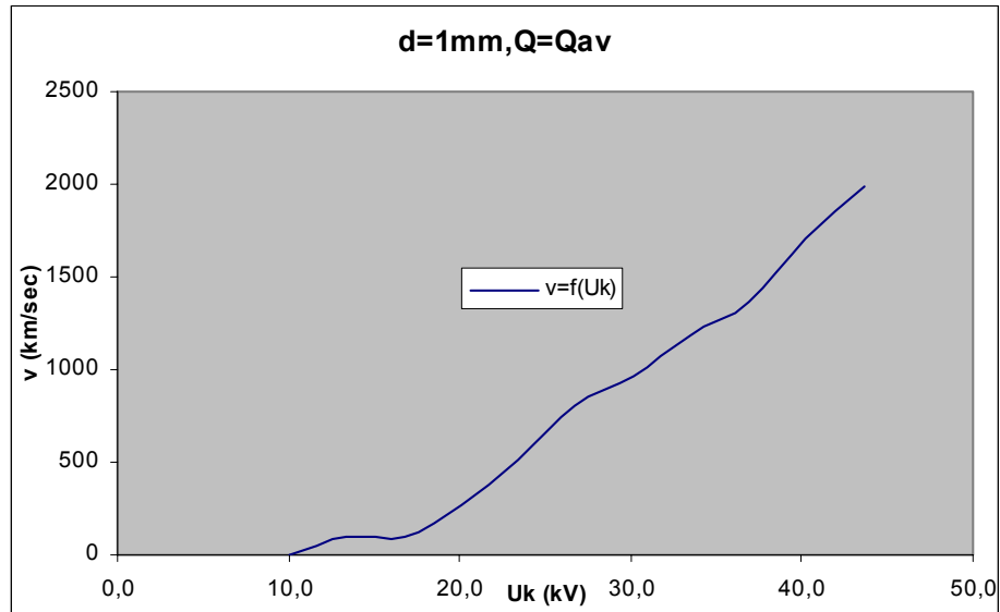
Σχήμα Β 2.1.5 Μεταβολή Ταχύτητας Ηλεκτρονίων σε συνάρτηση με την Κρουστική Τάση
