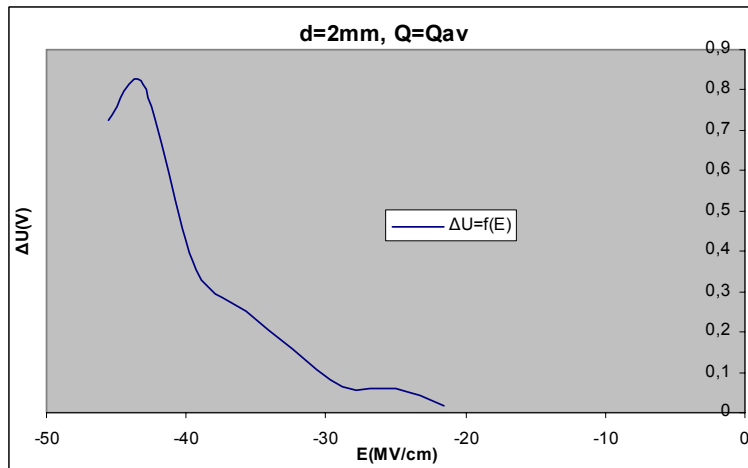
Σχήμα B 2.4.1 Μεταβολή Άλματος Δυναμικού σε συνάρτηση με την Κρουστική Τάση
