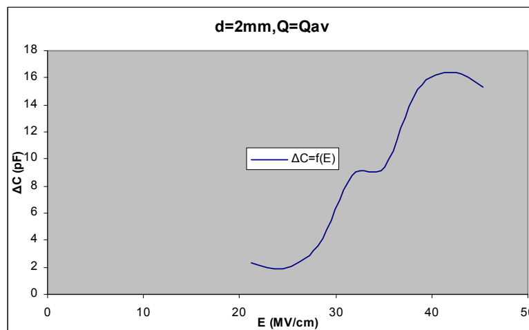
Σχήμα Β 2.3.8 Μεταβολή Χωρητικότητας σε συνάρτηση με την Ένταση του Ηλεκτρικού Πεδίου
