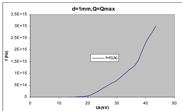
Σχήμα Β 2.5.11 Μεταβολή Συχνότητας σε συνάρτηση με την Κρουστική Τάση
