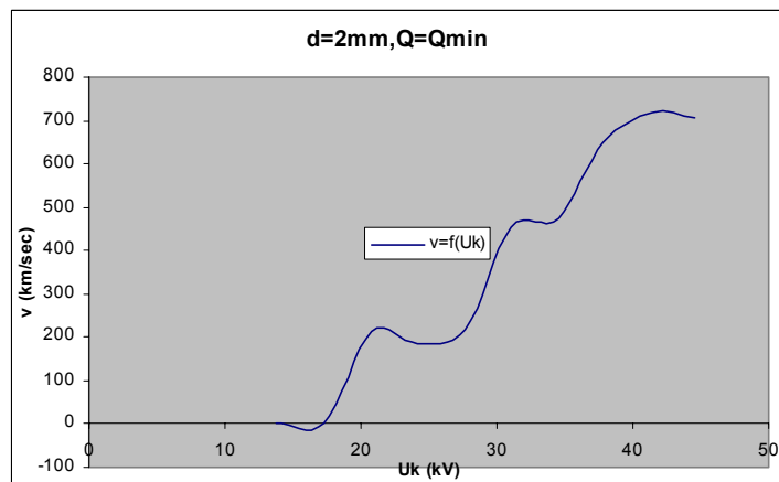
Σχήμα Β 2.10.5 Μεταβολή Ταχύτητας Ηλεκτρονίων σε συνάρτηση με την Κρουστική Τάση
