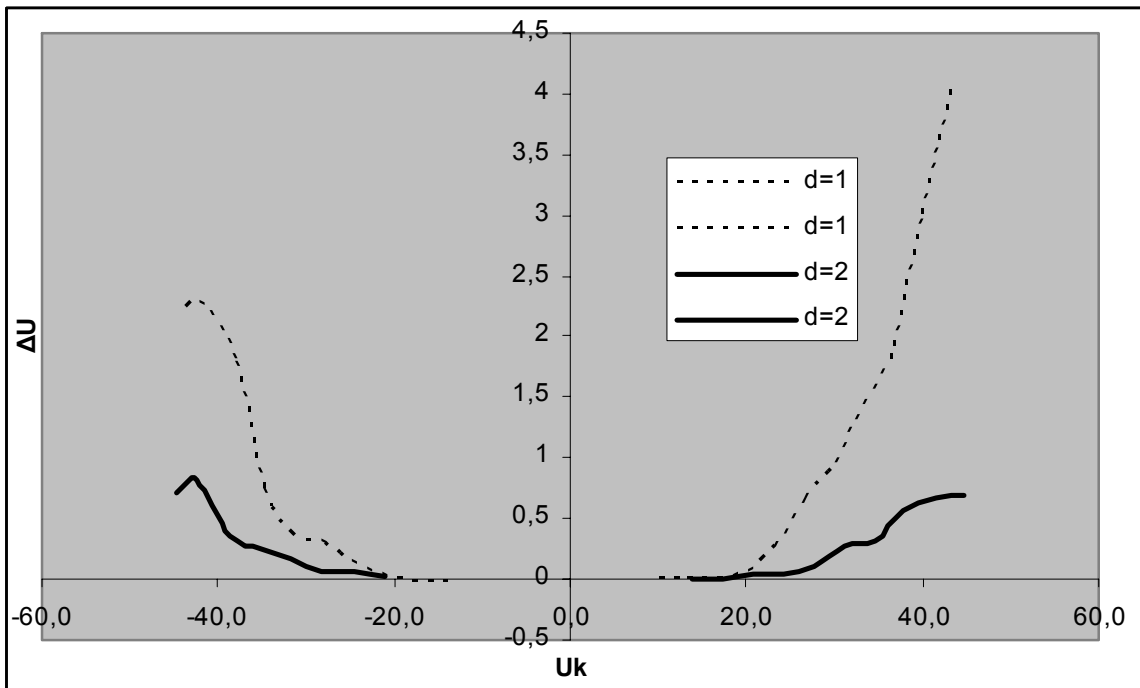
Σχήμα Δ.1 Επίδραση πάχους δοκιμίου και πολικότητας κρουστικής τάσης στα άλματα δυναμικού
