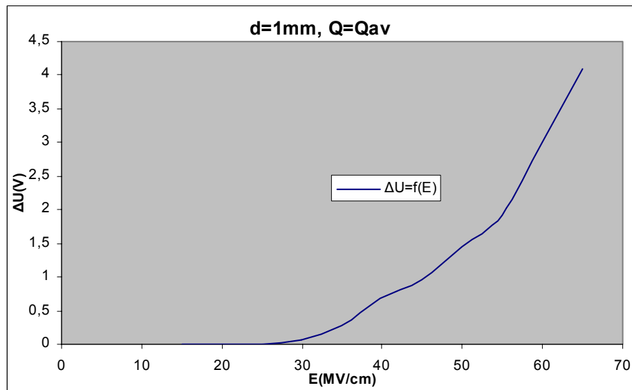
Σχήμα B 2.1.2 Μεταβολή Άλματος Δυναμικού σε συνάρτηση με την Ένταση του Ηλεκτρικού Πεδίου
