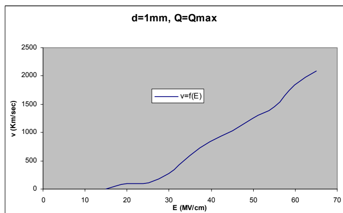
Σχήμα Β 2.5.6 Μεταβολή Ταχύτητας Ηλεκτρονίων σε συνάρτηση με την Ένταση του Ηλεκτρικού Πεδίου
