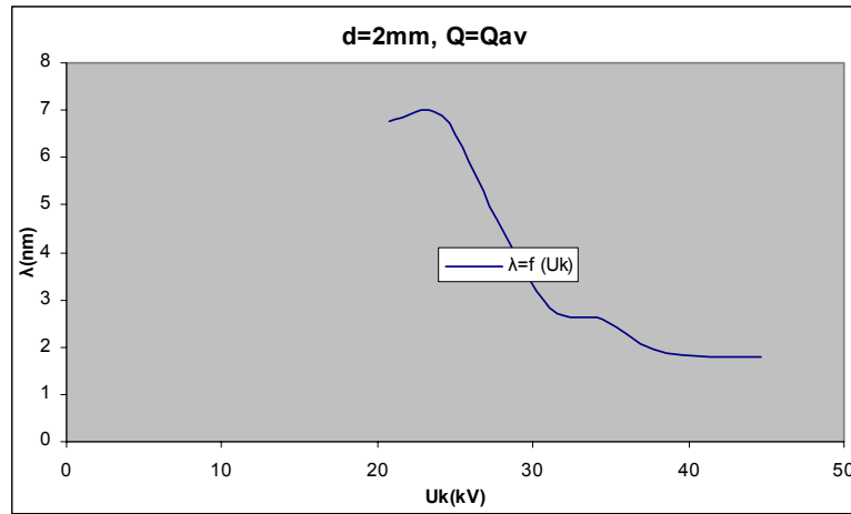
Σχήμα Β 2.3.9 Μεταβολή Μήκους Κύματος σε συνάρτηση με την Κρουστική Τάση
