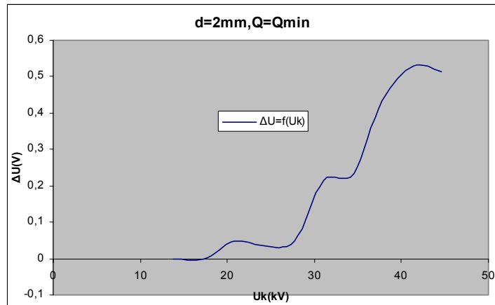
Σχήμα Β 2.10.1 Μεταβολή Άλματος Δυναμικού σε συνάρτηση με την Κρουστική Τάση
