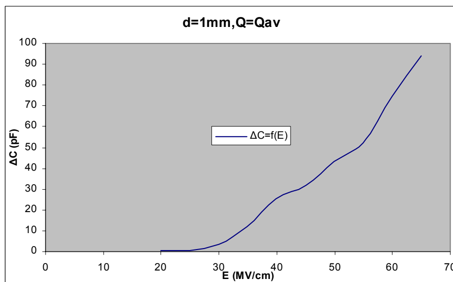
Σχήμα Β 2.1.8 Μεταβολή Χωρητικότητας σε συνάρτηση με την Ένταση του Ηλεκτρικού Πεδίου
