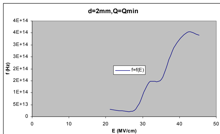
Σχήμα Β 2.10.12 Μεταβολή Συχνότητας σε συνάρτηση με την Ένταση του Ηλεκτρικού Πεδίου
