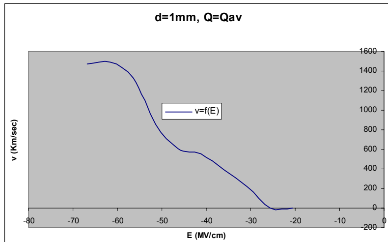
Σχήμα B 2.2.6 Μεταβολή Ταχύτητας Ηλεκτρονίων σε συνάρτηση με την Ένταση του Ηλεκτρικού Πεδίου
