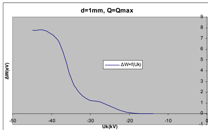
Σχήμα Β 2.7.3 Μεταβολή Ενέργειας Η/Μ Ακτινοβολίας σε συνάρτηση με την Κρουστική Τάση
