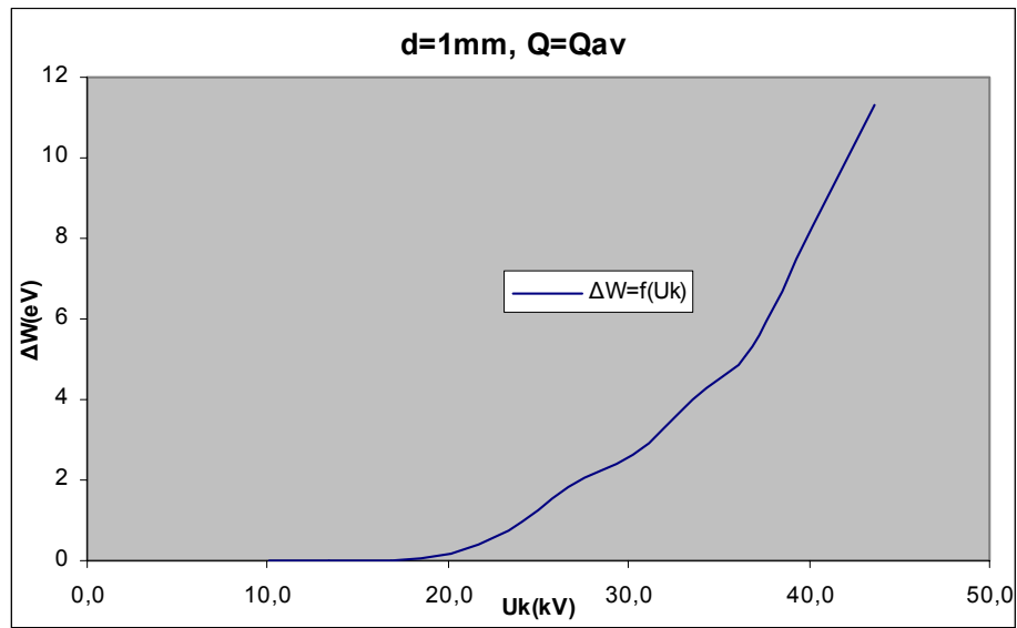
Σχήμα Β 2.1.3 Μεταβολή Ενέργειας Η/Μ Ακτινοβολίας σε συνάρτηση με την Κρουστική Τάση
