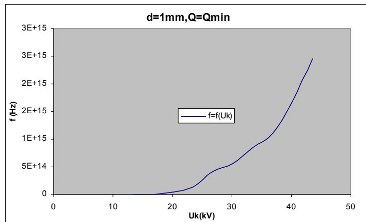
Σχήμα Β 2.6.11 Μεταβολή Συχνότητας σε συνάρτηση με την Κρουστική Τάση
