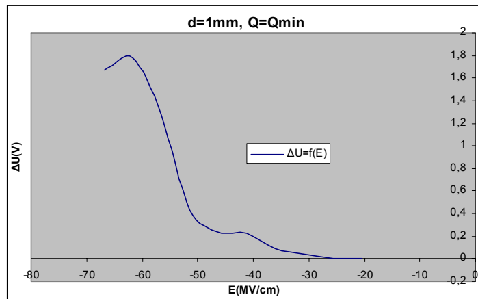
Σχήμα Β 2.8.2 Μεταβολή Άλματος Δυναμικού σε συνάρτηση με την Ένταση του Ηλεκτρικού Πεδίου
