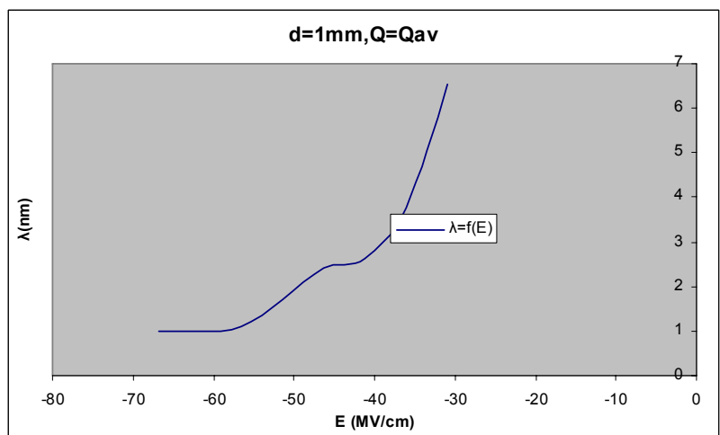
Σχήμα Β 2.2.10 Μεταβολή Μήκους Κύματος σε συνάρτηση με την Ένταση του Ηλεκτρικού Πεδίου
