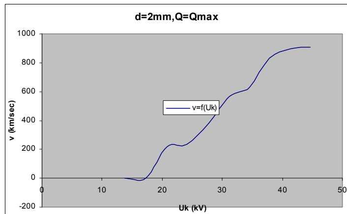
Σχήμα Β 2.9.5 Μεταβολή Ταχύτητας Ηλεκτρονίων σε συνάρτηση με την Κρουστική Τάση
