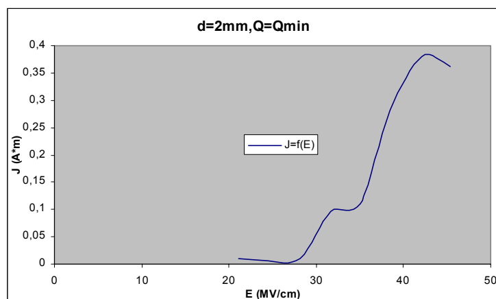
Σχήμα Β 2.10.16 Μεταβολή Πυκνότητας Ρεύματος σε συνάρτηση με την Ένταση του Ηλεκτρικού Πεδίου
