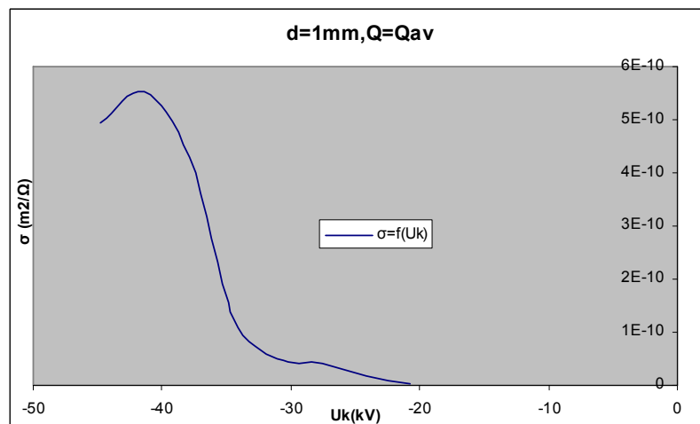
Σχήμα Β 2.2.13 Μεταβολή Ειδικής Αγωγιμότητας σε συνάρτηση με την Κρουστική Τάση
