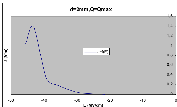
Σχήμα Β 2.11.16 Μεταβολή Πυκνότητας Ρεύματος σε συνάρτηση με την Ένταση του Ηλεκτρικού Πεδίου
