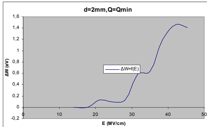
Σχήμα Β 2.10.4 Μεταβολή Ενέργειας Η/Μ Ακτινοβολίας σε συνάρτηση με την Ένταση του Ηλεκτρικού Πεδίου
