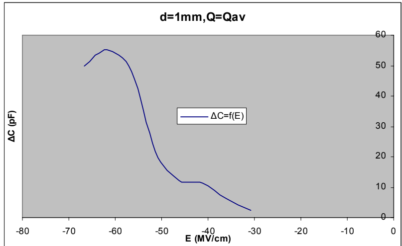
Σχήμα Β 2.2.8 Μεταβολή Χωρητικότητας σε συνάρτηση με την Ένταση του Ηλεκτρικού Πεδίου
