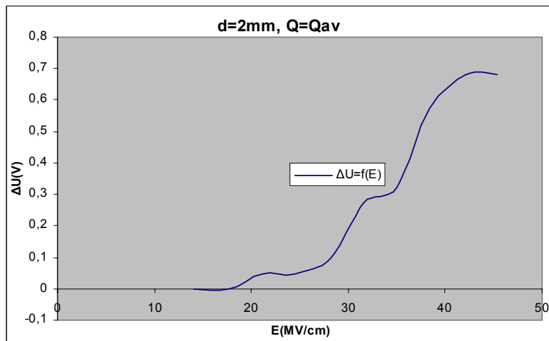
Σχήμα Β 2.3.2 Μεταβολή Άλματος Δυναμικού σε συνάρτηση με την Ένταση του Ηλεκτρικού Πεδίου
