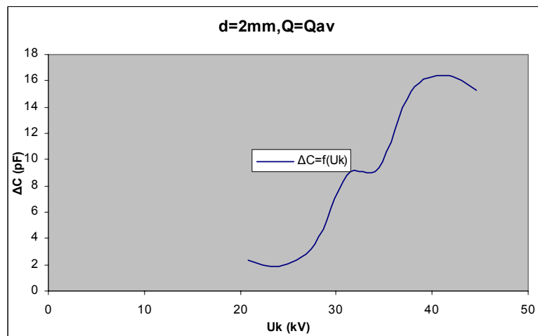
Σχήμα Β 2.3.7 Μεταβολή Χωρητικότητας σε συνάρτηση με την Κρουστική Τάση
