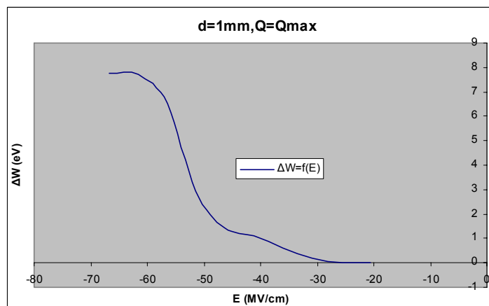
Σχήμα Β 2.7.4 Μεταβολή Ενέργειας Η/Μ Ακτινοβολίας σε συνάρτηση με την Ένταση του Ηλεκτρικού Πεδίου
