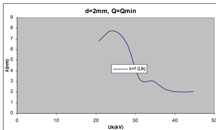
Σχήμα Β 2.10.9 Μεταβολή Μήκους Κύματος σε συνάρτηση με την Κρουστική Τάση
