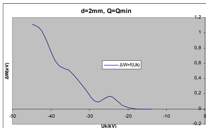
Σχήμα Β 2.12.3 Μεταβολή Ενέργειας Η/Μ Ακτινοβολίας σε συνάρτηση με την Κρουστική Τάση
