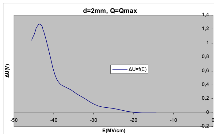
Σχήμα Β 2.11.2 Μεταβολή Άλματος Δυναμικού σε συνάρτηση με την Ένταση του Ηλεκτρικού Πεδίου
