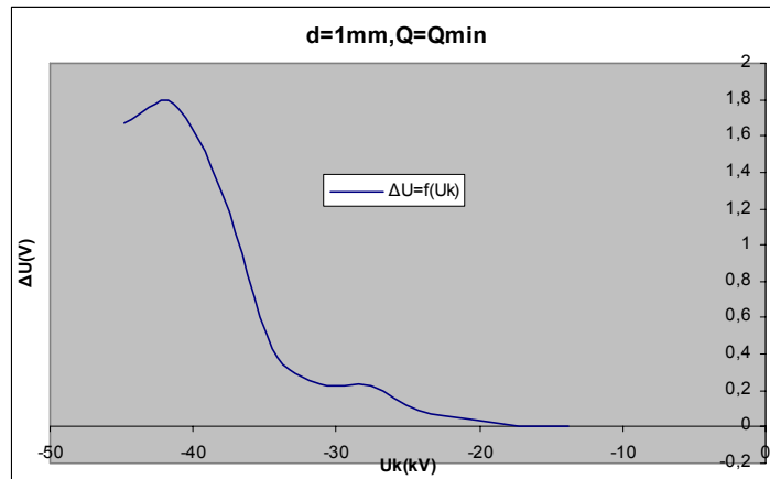
Σχήμα Β 2.8.1 Μεταβολή Άλματος Δυναμικού σε συνάρτηση με την Κρουστική Τάση
