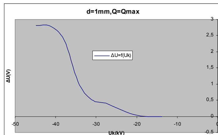
Σχήμα Β 2.7.1 Μεταβολή Άλλματος Δυναμικού σε συνάρτηση με την Κρουστική Τάση
