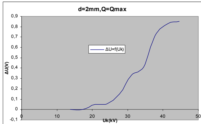
Σχήμα Β 2.9.1 Μεταβολή Άλματος Δυναμικού σε συνάρτηση με την Κρουστική Τάση
