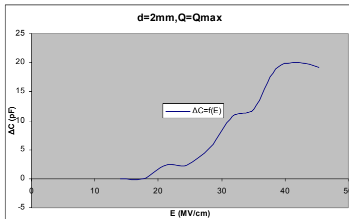
Σχήμα Β 2.9.8 Μεταβολή Χωρητικότητας σε συνάρτηση με την Ένταση του Ηλεκτρικού Πεδίου
