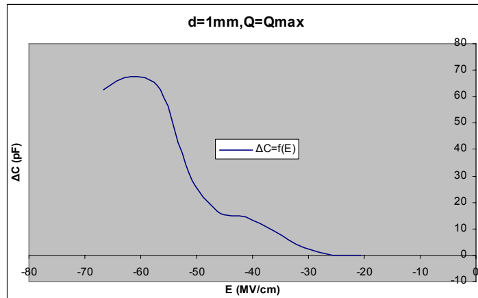
Σχήμα Β 2.7.8 Μεταβολή Χωρητικότητας σε συνάρτηση με την Ένταση του Ηλεκτρικού Πεδίου
