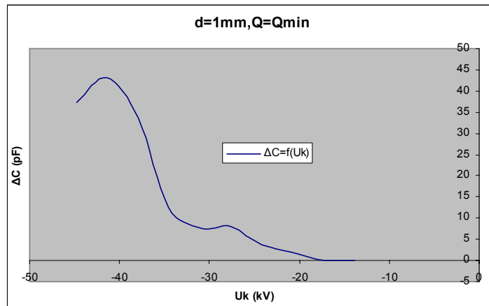
Σχήμα Β 2.8.7 Μεταβολή Χωρητικότητας σε συνάρτηση με την Κρουστική Τάση
