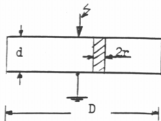
Σχήμα A2.3.2.1-1: Απλοποιημένη παράσταση του σχετού διάτρησης λόγω των απωλειών Joule του στερεού μονωτικού .
