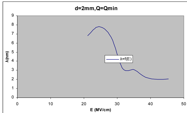
Σχήμα Β 2.10.10 Μεταβολή Μήκους Κύματος σε συνάρτηση με την Ένταση του Ηλεκτρικού Πεδίου
