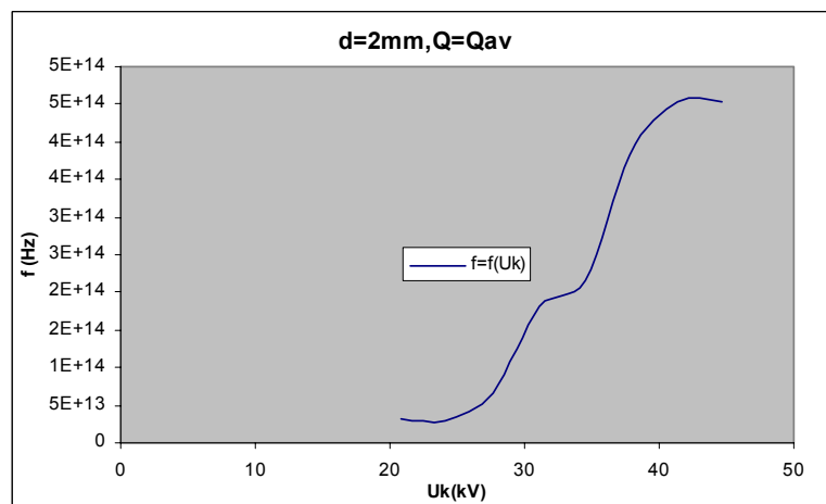
Σχήμα Β 2.3.11 Μεταβολή Συχνότητας σε συνάρτηση με την Κρουστική Τάση
