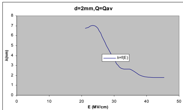
Σχήμα Β 2.3.10 Μεταβολή Μήκους Κύματος σε συνάρτηση με την Ένταση του Ηλεκτρικού Πεδίου
