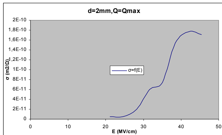
Σχήμα Β 2.9.14 Μεταβολή Ειδικής Αγωγιμότητας σε συνάρτηση με την Ένταση του Ηλεκτρικού Πεδίου
