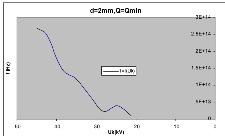
Σχήμα Β 2.12.11 Μεταβολή Συχνότητας σε συνάρτηση με την Κρουστική Τάση
