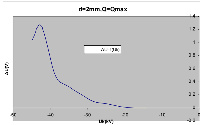
Σχήμα Β 2.11.1 Μεταβολή Άλματος Δυναμικού σε συνάρτηση με την Κρουστική Τάση
