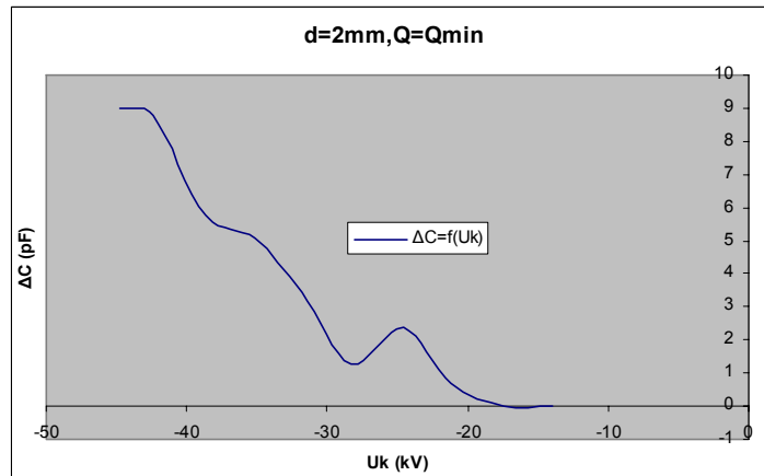
Σχήμα Β 2.12.7 Μεταβολή Χωρητικότητας σε συνάρτηση με την Κρουστική Τάση
