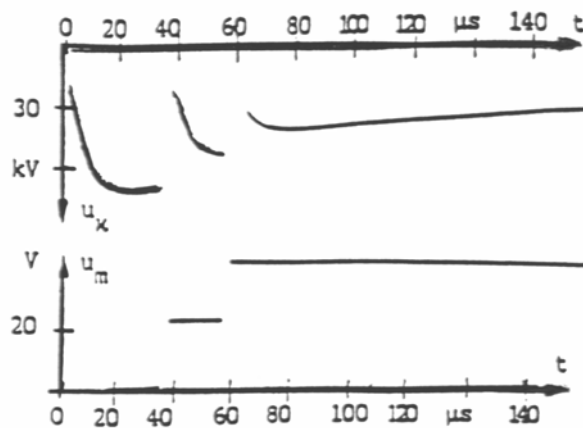
Σχήμα A2.3.5-1 : Παλμογράφημα αλμάτων δυναμικού κατά την επιφανειακή διάσπαση του pertinax (πάχους 2mm και με διάμετρο της επιφάνειάς του 150mm), υπό κρουστικές τάσεις 10/200 \mu\text{s} σε περιβάλλον μονωτικού ελαίου. Ηλεκτρόδια εφαρμογής της τάσης : «ακίδα-πλάκα».
