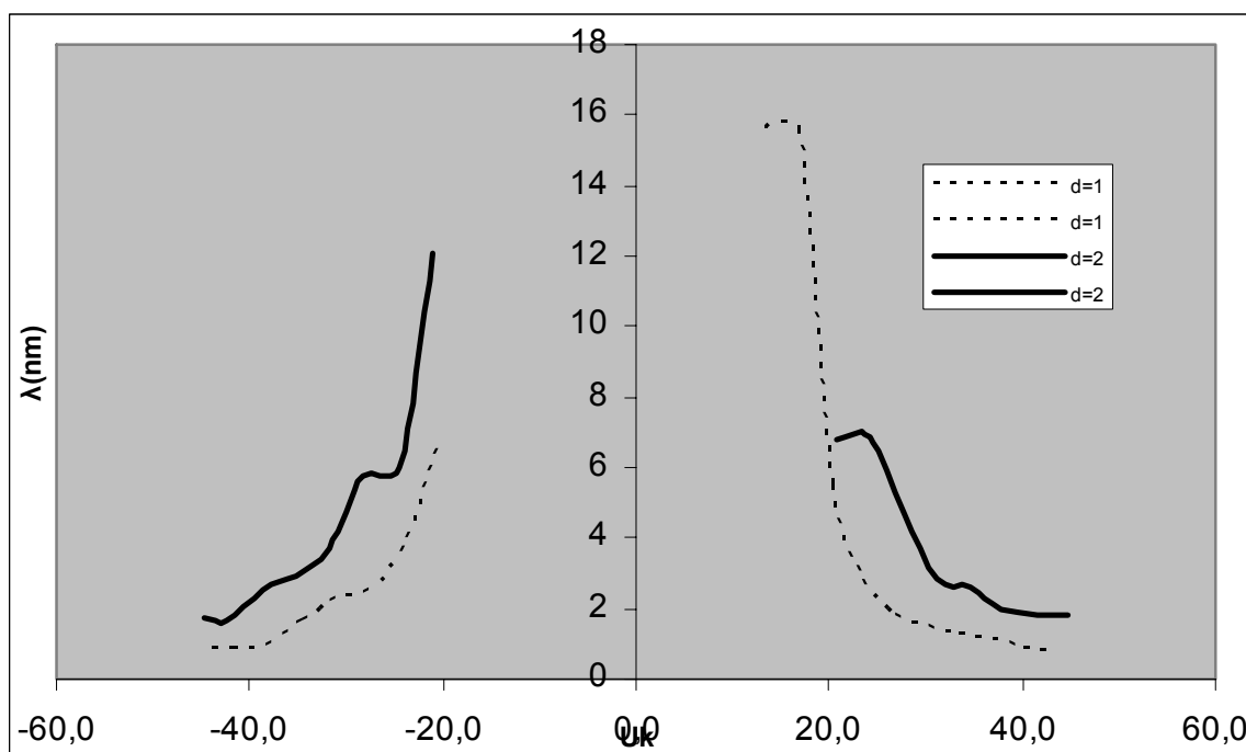
Σχήμα Δ.3 Επίδραση πάχους δοκιμίου και πολικότητας κρουστικής τάσης στο μήκος κύματος της εκπεμπόμενης ακτινοβολίας
