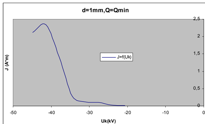
Σχήμα Β 2.8.15 Μεταβολή Πυκνότητας Ρεύματος σε συνάρτηση με την Κρουστική Τάση
