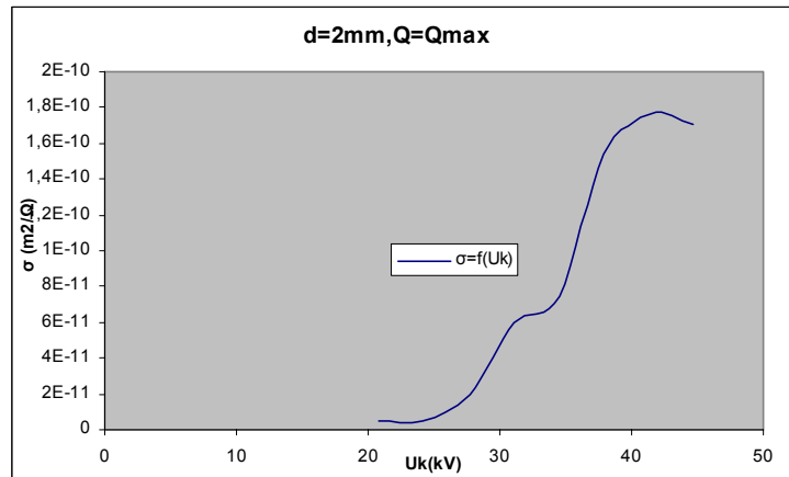
Σχήμα Β 2.9.13 Μεταβολή Ειδικής Αγωγιμότητας σε συνάρτηση με την Κρουστική Τάση
