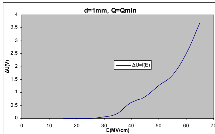
Σχήμα B 2.6.2 Μεταβολή Άλματος Δυναμικού σε συνάρτηση με την Ένταση του Ηλεκτρικού Πεδίου
