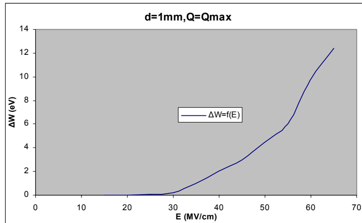
Σχήμα Β 2.5.4 Μεταβολή Ενέργειας Η/Μ Ακτινοβολίας σε συνάρτηση με την Ένταση του Ηλεκτρικού Πεδίου
