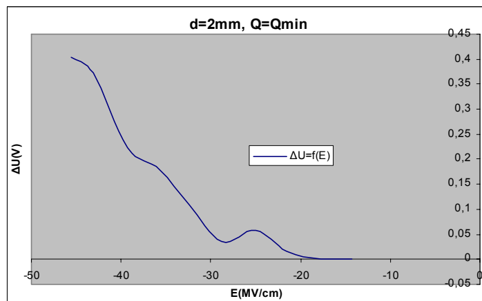
Σχήμα Β 2.12.2 Μεταβολή Άλματος Δυναμικού σε συνάρτηση με την Ένταση του Ηλεκτρικού Πεδίου
