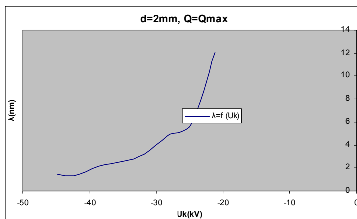
Σχήμα Β 2.11.9 Μεταβολή Μήκους Κύματος σε συνάρτηση με την Κρουστική Τάση
