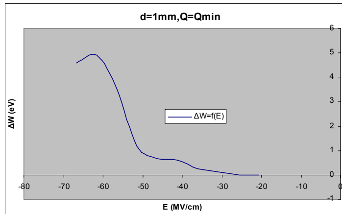
Σχήμα Β 2.8.4 Μεταβολή Ενέργειας Η/Μ Ακτινοβολίας σε συνάρτηση με την Ένταση του Ηλεκτρικού Πεδίου
