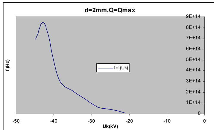
Σχήμα Β 2.11.11 Μεταβολή Συχνότητας σε συνάρτηση με την Κρουστική Τάση
