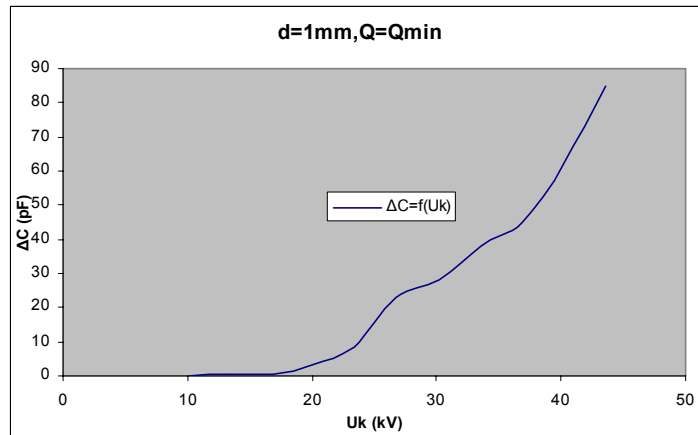
Σχήμα Β 2.6.7 Μεταβολή Χωρητικότητας σε συνάρτηση με την Κρουστική Τάση
