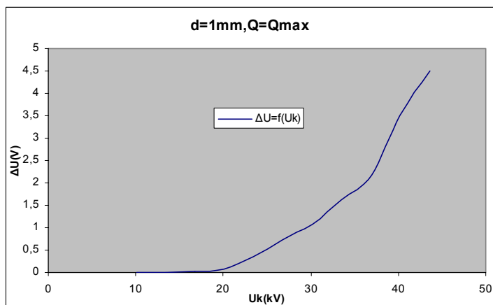
Σχήμα B 2.5.1 Μεταβολή Άλματος Δυναμικού σε συνάρτηση με την Κρουστική Τάση
