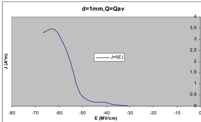
Σχήμα Β 2.2.16 Μεταβολή Πυκνότητας Ρεύματος σε συνάρτηση με την Ένταση του Ηλεκτρικού Πεδίου
