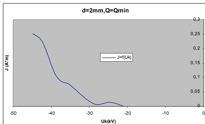
Σχήμα Β 2.12.15 Μεταβολή Πυκνότητας Ρεύματος σε συνάρτηση με την Κρουστική Τάση
