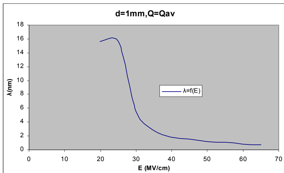
Σχήμα Β 2.1.10 Μεταβολή Μήκους Κύματος Ακτινοβολίας σε συνάρτηση με την Ένταση του Ηλεκτρικού Πεδίου
