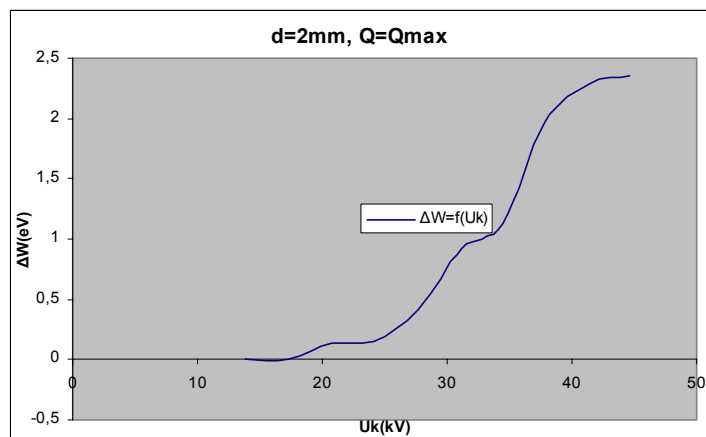
Σχήμα Β 2.9.3 Μεταβολή Ενέργειας Η/Μ Ακτινοβολίας σε συνάρτηση με την Κρουστική Τάση
