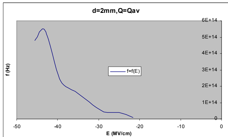
Σχήμα Β 2.4.12 Μεταβολή Συχνότητας σε συνάρτηση με την Ένταση του Ηλεκτρικού Πεδίου
