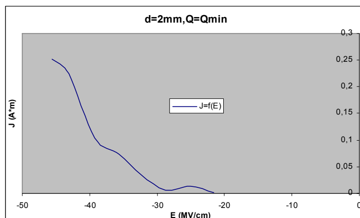
Σχήμα Β 2.12.16 Μεταβολή Πυκνότητας Ρεύματος σε συνάρτηση με την Ένταση του Ηλεκτρικού Πεδίου
