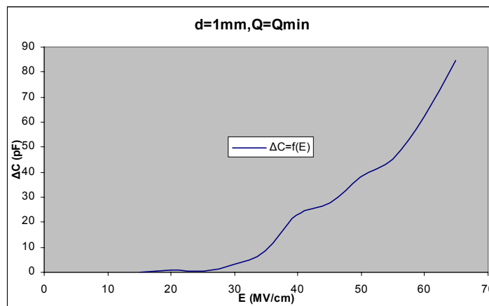
Σχήμα Β 2.6.8 Μεταβολή Χωρητικότητας σε συνάρτηση με την Ένταση του Ηλεκτρικού Πεδίου
