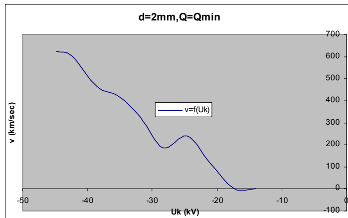
Σχήμα Β 2.12.5 Μεταβολή Ταχύτητας Ηλεκτρονίων σε συνάρτηση με την Κρουστική Τάση
