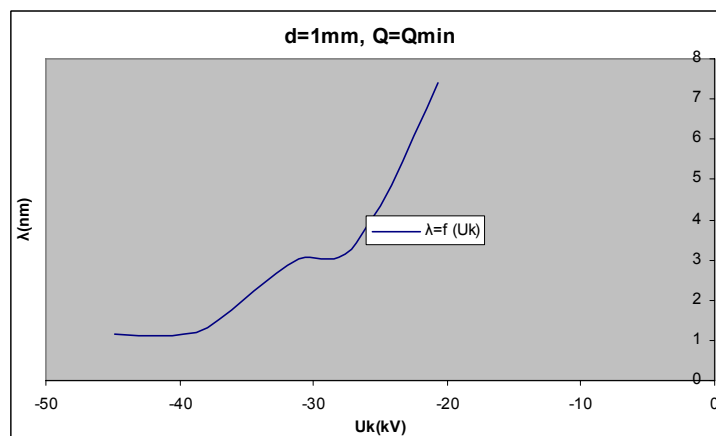
Σχήμα Β 2.8.9 Μεταβολή Μήκους Κύματος σε συνάρτηση με την Κρουστική Τάση
