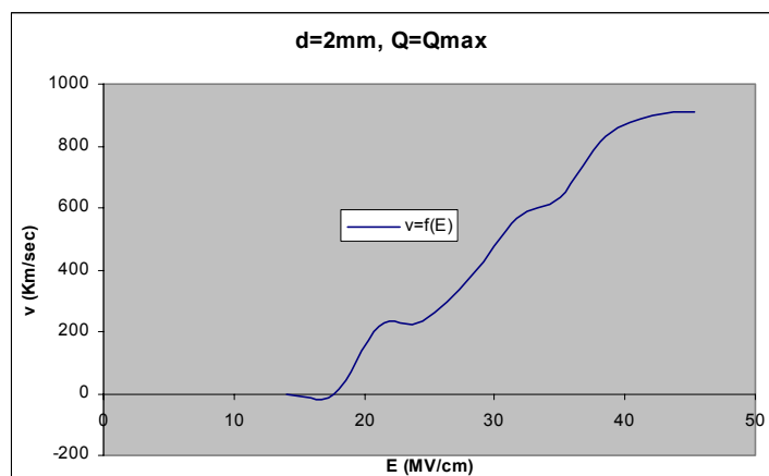
Σχήμα Β 2.9.6 Μεταβολή Ταχύτητας Ηλεκτρονίων σε συνάρτηση με την Ένταση του Ηλεκτρικού Πεδίου
