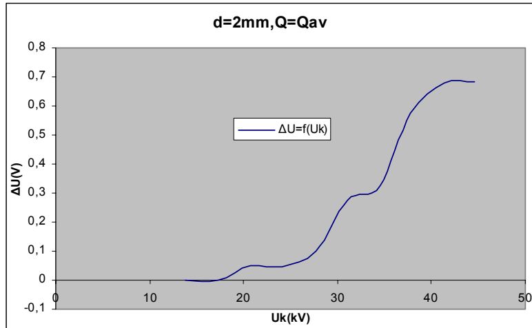
Σχήμα Β 2.3.1 Μεταβολή Άλματος Δυναμικού σε συνάρτηση με την Κρουστική Τάση
