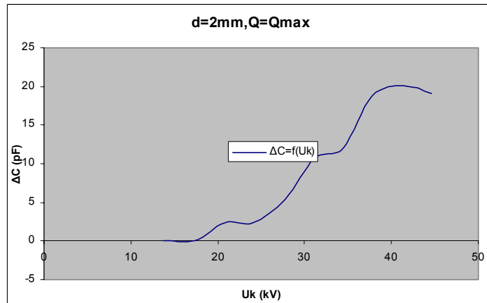
Σχήμα Β 2.9.7 Μεταβολή Χωρητικότητας σε συνάρτηση με την Κρουστική Τάση
