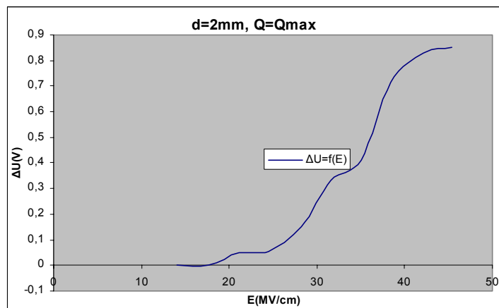
Σχήμα Β 2.9.2 Μεταβολή Άλματος Δυναμικού σε συνάρτηση με την Ένταση του Ηλεκτρικού Πεδίου
