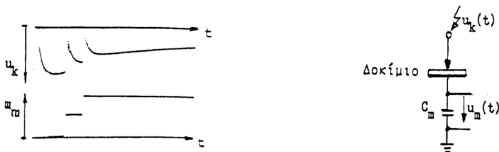
Σχήμα A2.3.2.5 : Τυπικό παλμογράφημα της επιφανειακής διάσπασης πολυμερών στερεών μονωτικών (πάχους 2mm) εντός μονωτικού ελαίου, υπό κρουστική τάση 10/200 \mu\text{s} και διάταξη ηλεκτροδίων ακίδα –πλάκα.
