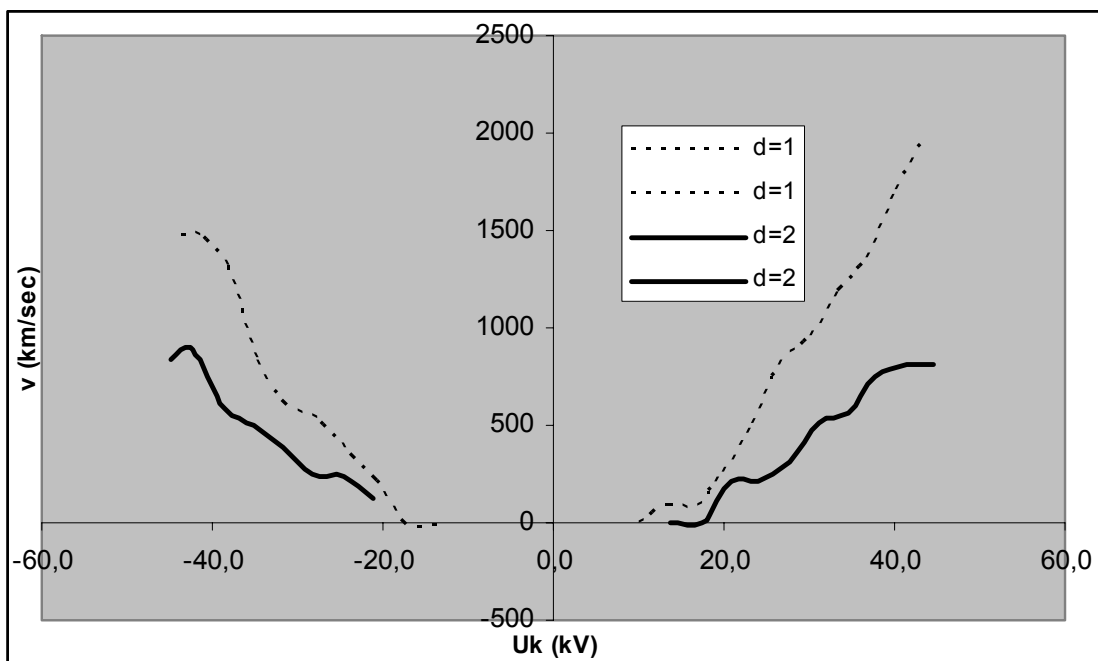
Σχήμα Δ.5 Επίδραση πάχους δοκιμίου και πολικότητας κρουστικής τάσης στην ταχύτητα των ηλεκτρονίων
