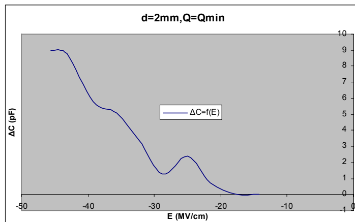
Σχήμα Β 2.12.8 Μεταβολή Χωρητικότητας σε συνάρτηση με την Ένταση του Ηλεκτρικού Πεδίου
