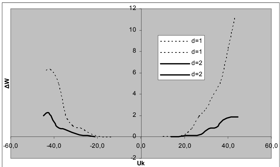
Σχήμα Δ.2 Επίδραση πάχους δοκιμίου και πολικότητας κρουστικής τάσης στην ενέργεια της ακτινοβολίας
