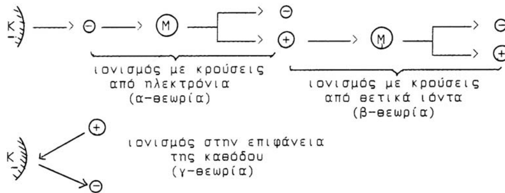
Σχήμα Α2.1.1-1: Ένα μακροσκοπικό μοντέλο για τις περιπτώσεις ιονισμού με κρούσεις κατά τη θεωρία Thowsend.
