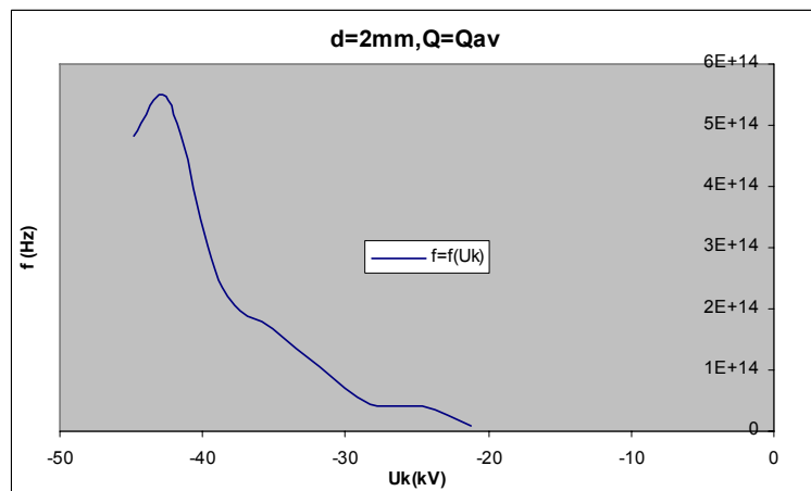
Σχήμα Β 2.4.11 Μεταβολή Συχνότητας σε συνάρτηση με την Κρουστική Τάση
