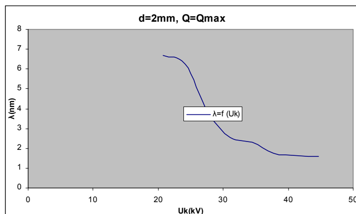
Σχήμα Β 2.9.9 Μεταβολή Μήκους Κύματος σε συνάρτηση με την Κρουστική Τάση
