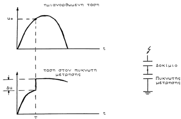
Σχήμα A2.3.2.6-3 : Παράδειγμα καθορισμού ορισμένων εννοιών για την στατιστική μελέτη των μερικών εκκενώσεων σε στερεά μονωτικά, των πρακτικών εφαρμογών, υπό ημιανορθωμένες τάσεις καταπόνησης. T_1 : Χρόνος έναρξης των μερικών εκκενώσεων. u_0 : Τάση έναρξης των μερικών εκκενώσεων (στιγμιαία τιμή). \Delta u : άλμα δυναμικού.
