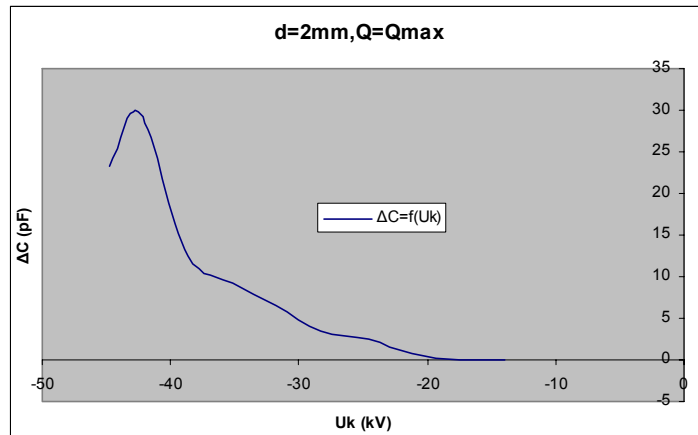
Σχήμα Β 2.11.7 Μεταβολή Χωρητικότητας σε συνάρτηση με την Κρουστική Τάση
