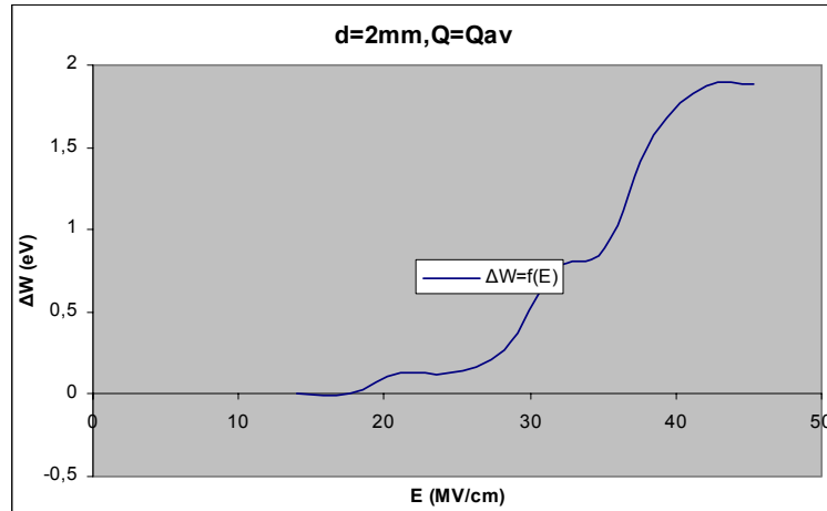
Σχήμα Β 2.3.4 Μεταβολή Ενέργειας Η/Μ Ακτινοβολίας σε συνάρτηση με την Ένταση του Ηλεκτρικού Πεδίου
