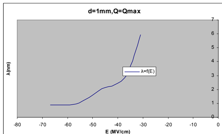
Σχήμα Β 2.7.10 Μεταβολή Μήκους Κύματος σε συνάρτηση με την Ένταση του Ηλεκτρικού Πεδίου
