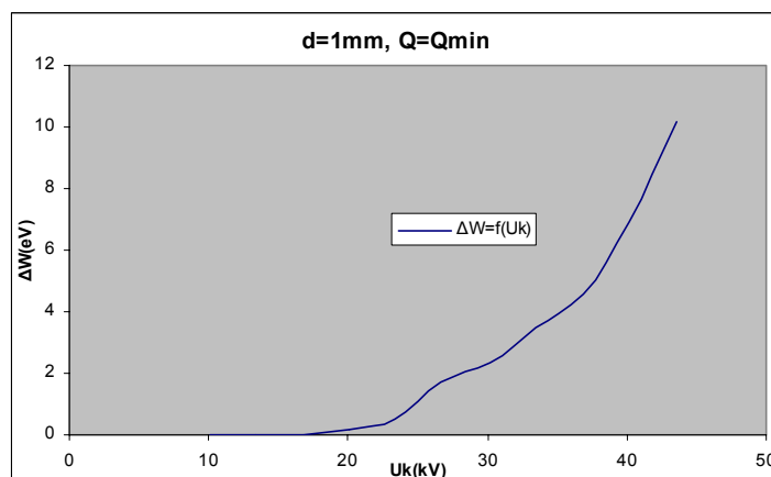
Σχήμα B 2.6.3 Μεταβολή Ενέργειας Η/Μ Ακτινοβολίας σε συνάρτηση με την Κρουστική Τάση
