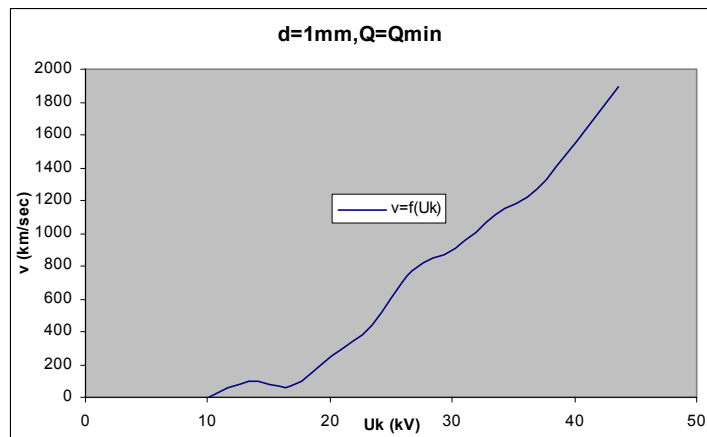
Σχήμα Β 2.6.5 Μεταβολή Ταχύτητας Ηλεκτρονίων σε συνάρτηση με την Κρουστική Τάση
