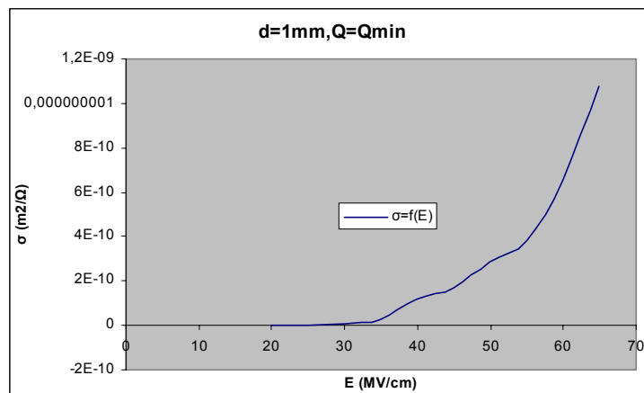
Σχήμα B 2.6.14 Μεταβολή Ειδικής Αγωγιμότητας σε συνάρτηση με την Ένταση του Ηλεκτρικού Πεδίου
