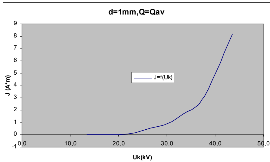
Σχήμα B 2.1.15 Μεταβολή Πυκνότητας Ρεύματος σε συνάρτηση με την Κρουστική Τάση
