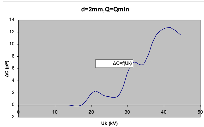
Σχήμα Β 2.10.7 Μεταβολή Χωρητικότητας σε συνάρτηση με την Κρουστική Τάση
