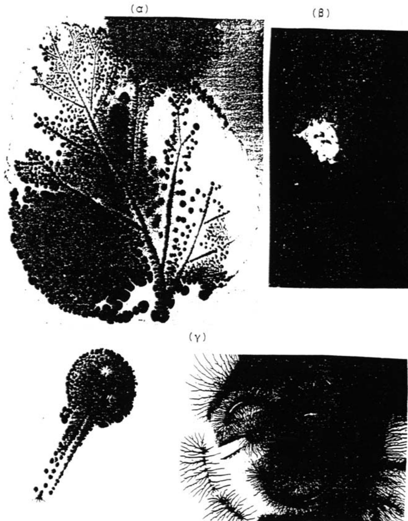
Σχήμα Α2.3.5-2 : Προσβολή του φωτογραφικού φιλμ κατά την επιφανειακή διάσπαση στον αέρα πολυμερούς στερεού μονωτικού, υπό κρουστική τάση 1,2/50μs. Διάταξη ηλεκτροδίων : ακίδα-πλάκα. α) Φωτογράφιση φύλλου δένδρου β) Φωτογραφία βιολογικού οργανισμού (σκαθάρι). γ) Φωτογραφία μεταλλικών αντικειμένων.
