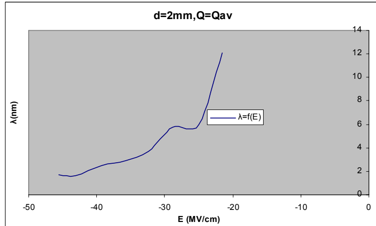
Σχήμα Β 2.4.10 Μεταβολή Μήκους Κύματος σε συνάρτηση με την Ένταση του Ηλεκτρικού Πεδίου
