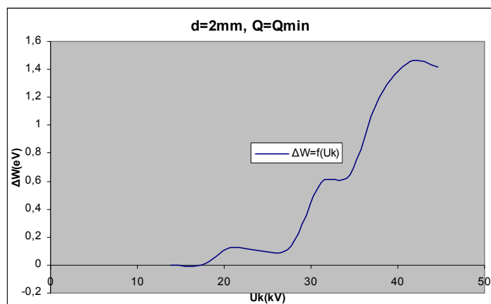
Σχήμα Β 2.10.3 Μεταβολή Ενέργειας Η/Μ Ακτινοβολίας σε συνάρτηση με την Κρουστική Τάση
