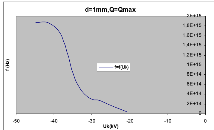
Σχήμα B 2.7.11 Μεταβολή Συχνότητας σε συνάρτηση με την Κρουστική Τάση
