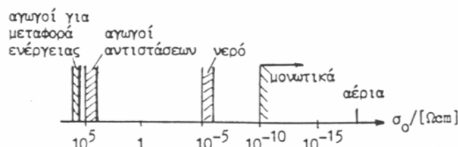
Σχήμα Α1.3-1 : Τάξη μεγέθους της ειδικής ηλεκτρικής αγωγιμότητας διαφόρων κατηγοριών υλικών.
