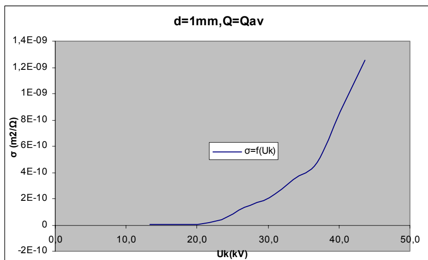
Σχήμα Β 2.1.13 Μεταβολή Ειδικής Αγωγιμότητας σε συνάρτηση με την Κρουστική Τάση
