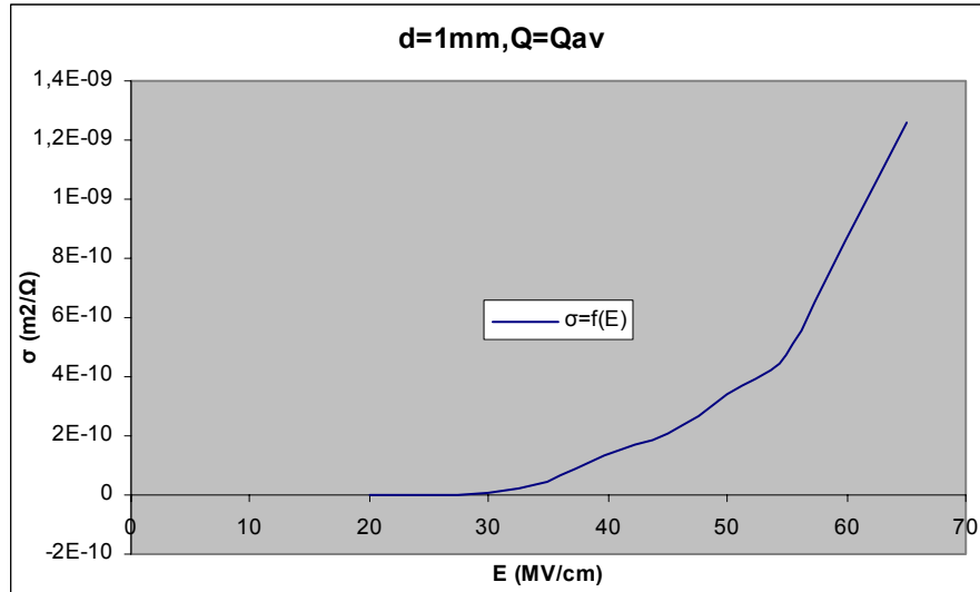
Σχήμα B 2.1.14 Μεταβολή Ειδικής Αγωγιμότητας σε συνάρτηση με την Ένταση του Ηλεκτρικού Πεδίου
