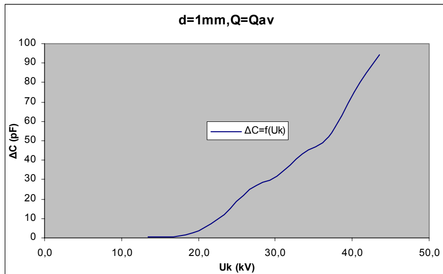
Σχήμα Β 2.1.7 Μεταβολή Χωρητικότητας σε συνάρτηση με την Κρουστική Τάση
