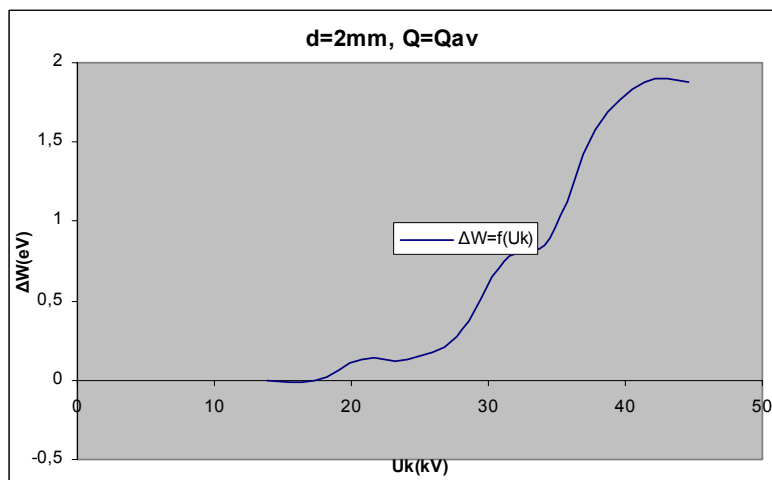
Σχήμα Β 2.3.3 Μεταβολή Ενέργειας Η/Μ Ακτινοβολίας σε συνάρτηση με την Κρουστική Τάση
