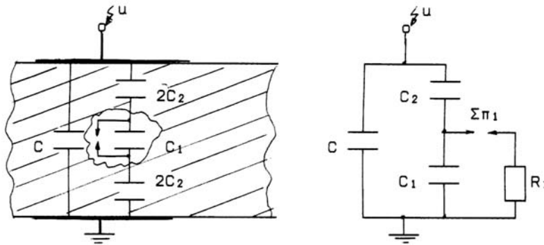
Σχήμα A2.3.2.3-3: Σχηματική παράσταση και ισοδύναμο κύκλωμα ενός στερεού μονωτικού με φυσαλίδα αερίου στον όγκο του (κατά Gemant και Philipoff).
