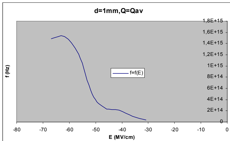
Σχήμα Β 2.2.11 Μεταβολή Συχνότητας σε συνάρτηση με την Κρουστική Τάση
