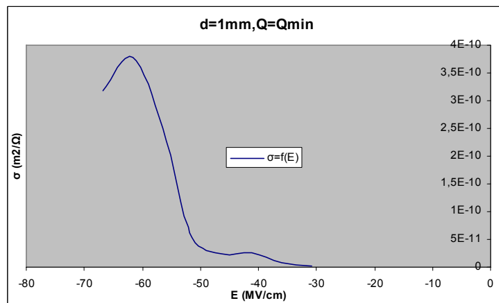
Σχήμα Β 2.8.14 Μεταβολή Ειδικής Αγωγιμότητας σε συνάρτηση με την Ένταση του Ηλεκτρικού Πεδίου
