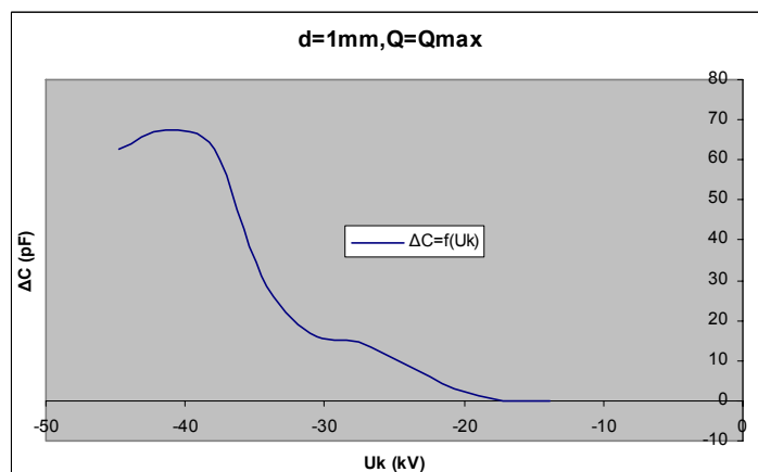
Σχήμα B 2.7.7 Μεταβολή Χωρητικότητας σε συνάρτηση με την Κρουστική Τάση
