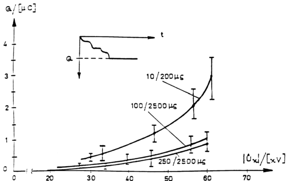
Σχήμα 2.3.2.6-4 : Χαρακτηριστική Q_2=f(\hat{U}_\kappa) για τον βακελίτη (πάχους 2mm), υπό κρουστικές τάσεις 10/200μs, 100/2500μs και 250/2500μs. Περιβάλλον μέσο : μονωτικό λάδι. Διάταξη ηλεκτροδίων : ακίδα-πλάκα. C_m : 1000nF.
