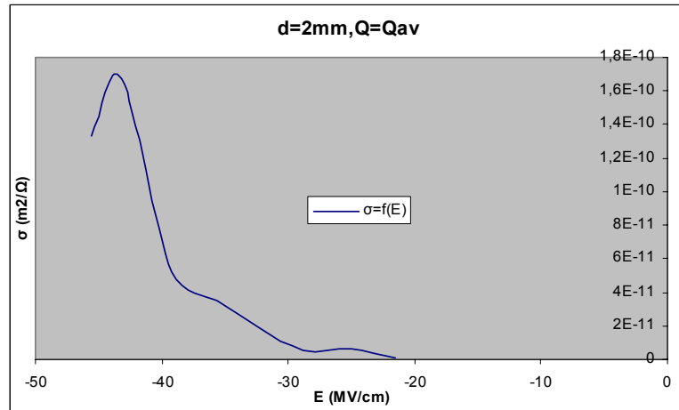
Σχήμα Β 2.4.14 Μεταβολή Ειδικής Αγωγιμότητας σε συνάρτηση με την Ένταση του Ηλεκτρικού Πεδίου
