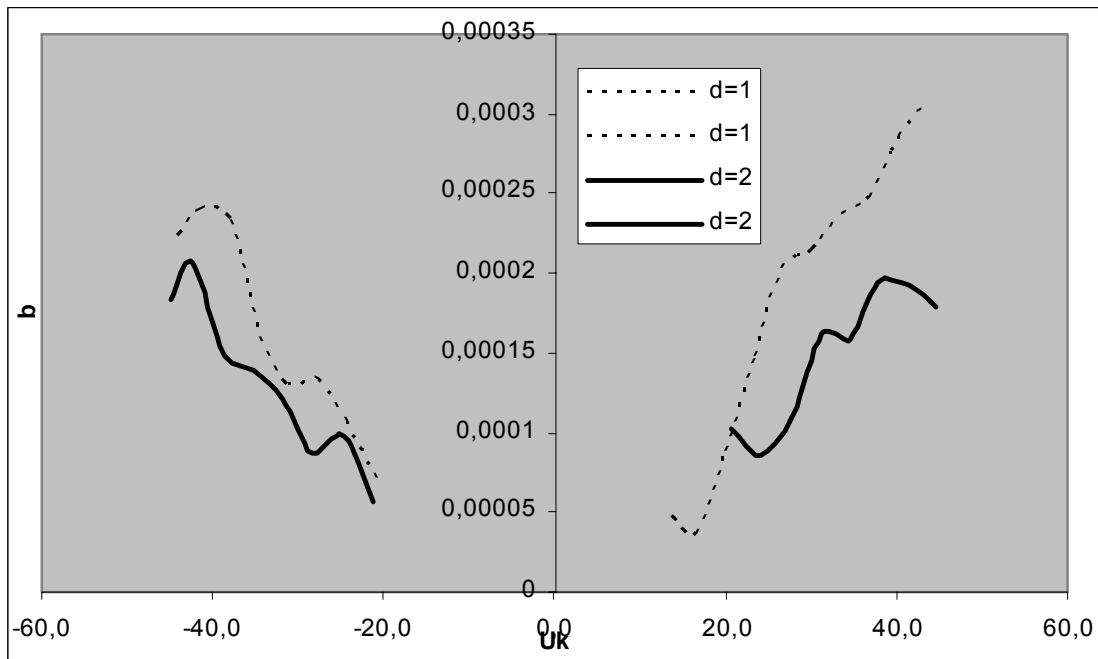
Σχήμα Δ.4 Επίδραση πάχους δοκιμίου και πολικότητας κρουστικής τάσης στην κινητικότητα των ηλεκτρονίων
