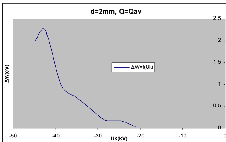
Σχήμα B 2.4.2 Μεταβολή Άλματος Δυναμικού σε συνάρτηση με την Ένταση του Ηλεκτρικού Πεδίου
