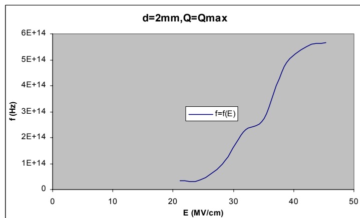
Σχήμα Β 2.9.12 Μεταβολή Συχνότητας σε συνάρτηση με την Ένταση του Ηλεκτρικού Πεδίου
