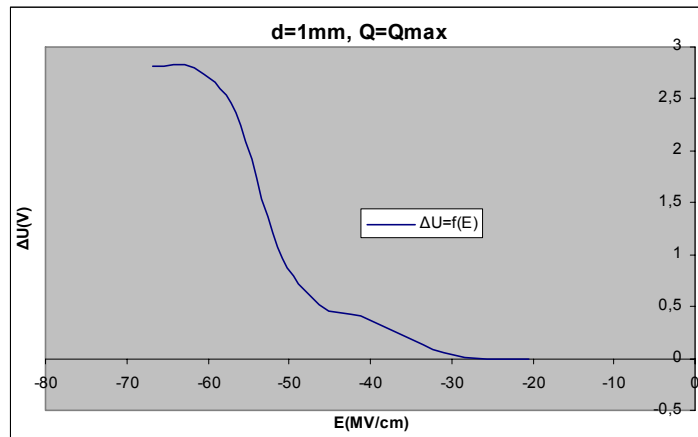
Σχήμα Β 2.7.2 Μεταβολή Άλματος Δυναμικού σε συνάρτηση με την Ένταση του Ηλεκτρικού Πεδίου
