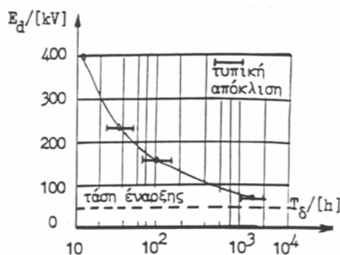
Σχήμα A2.3.2.3-2 : Μείωση της διηλεκτρικής αντοχής στο νάιλον πάχους 0,125mm, λόγω μερικών εκκενώσεων.
