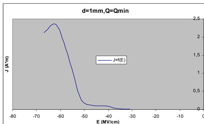
Σχήμα Β 2.8.16 Μεταβολή Πυκνότητας Ρεύματος σε συνάρτηση με την Ένταση του Ηλεκτρικού Πεδίου
