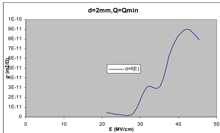
Σχήμα Β 2.10.14 Μεταβολή Ειδικής Αγωγιμότητας σε συνάρτηση με την Ένταση του Ηλεκτρικού Πεδίου
