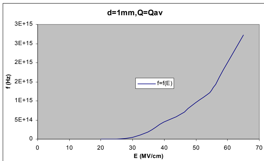
Σχήμα Β 2.1.11 Μεταβολή Συχνότητας Ακτινοβολίας σε συνάρτηση με την Κρουστική Τάση
