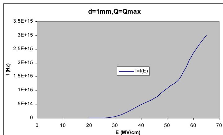
Σχήμα Β 2.5.12 Μεταβολή Συχνότητας σε συνάρτηση με την Ένταση του Ηλεκτρικού Πεδίου
