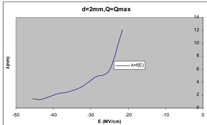
Σχήμα Β 2.11.10 Μεταβολή Μήκους Κύματος σε συνάρτηση με την Ένταση του Ηλεκτρικού Πεδίου
