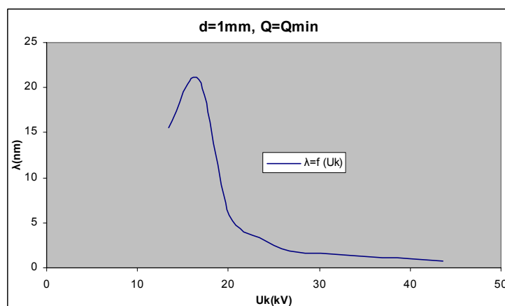
Σχήμα Β 2.6.9 Μεταβολή Μήκους Κύματος σε συνάρτηση με την Κρουστική Τάση
