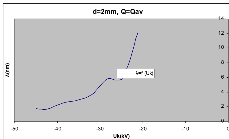
Σχήμα Β 2.4.9 Μεταβολή Μήκους Κύματος σε συνάρτηση με την Κρουστική Τάση
