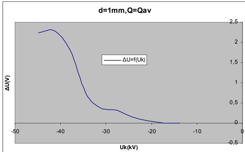
Σχήμα Β 2.2.1 Μεταβολή Άλματος Δυναμικού σε συνάρτηση με την Κρουστική Τάση
