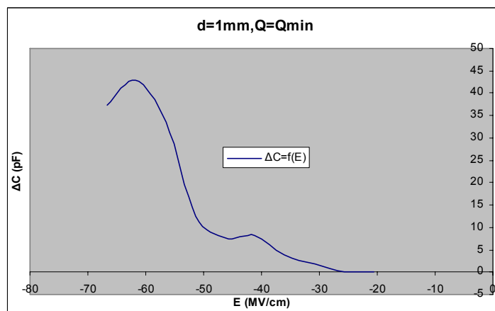
Σχήμα Β 2.8.8 Μεταβολή Χωρητικότητας σε συνάρτηση με την Ένταση του Ηλεκτρικού Πεδίου
