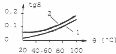
Σχήμα A1.3-3 : \text{tg}\delta ορισμένων διηλεκτρικών 1 : σκληρό χαρτί, 2 : πορσελάνη.
