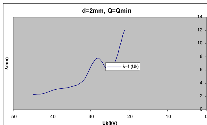
Σχήμα Β 2.12.9 Μεταβολή Μήκους Κύματος σε συνάρτηση με την Κρουστική Τάση
