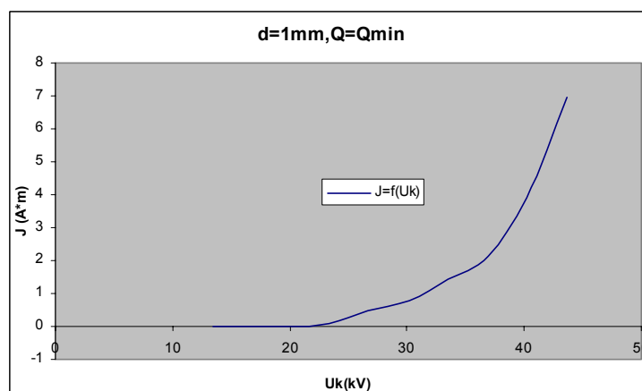
Σχήμα B 2.6.15 Μεταβολή Πυκνότητας Ρεύματος σε συνάρτηση με την Κρουστική Τάση
