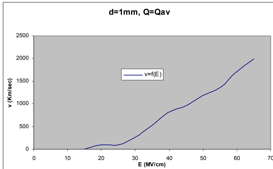
Σχήμα Β 2.1.6 Μεταβολή Ταχύτητας Ηλεκτρονίων σε συνάρτηση με την Ένταση του Ηλεκτρικού Πεδίου
