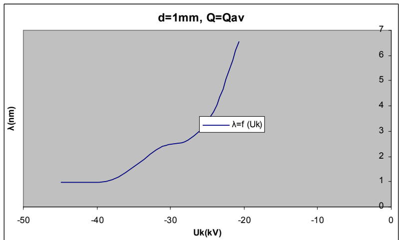
Σχήμα Β 2.2.9 Μεταβολή Μήκους Κύματος σε συνάρτηση με την Κρουστική Τάση
