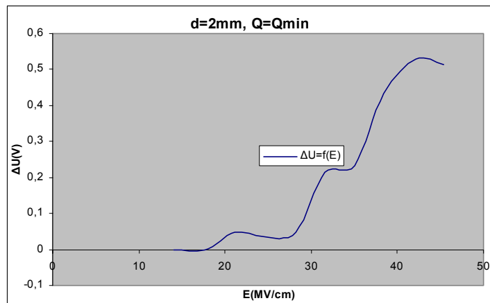
Σχήμα Β 2.10.2 Μεταβολή Άλματος Δυναμικού σε συνάρτηση με την Ένταση του Ηλεκτρικού Πεδίου
