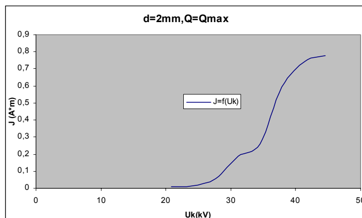
Σχήμα Β 2.9.15 Μεταβολή Πυκνότητας Ρεύματος σε συνάρτηση με την Κρουστική Τάση
