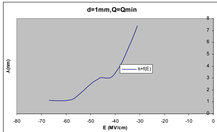
Σχήμα Β 2.8.10 Μεταβολή Μήκους Κύματος σε συνάρτηση με την Ένταση του Ηλεκτρικού Πεδίου
