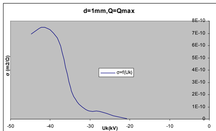
Σχήμα B 2.7.13 Μεταβολή Ειδικής Αγωγιμότητας σε συνάρτηση με την Κρουστική Τάση
