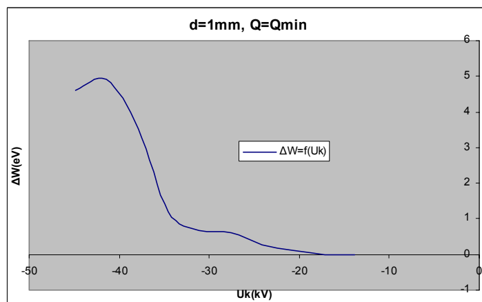
Σχήμα Β 2.8.3 Μεταβολή Ενέργειας Η/Μ Ακτινοβολίας σε συνάρτηση με την Κρουστική Τάση
