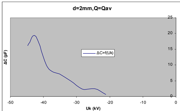
Σχήμα Β 2.4.7 Μεταβολή Χωρητικότητας σε συνάρτηση με την Κρουστική Τάση
