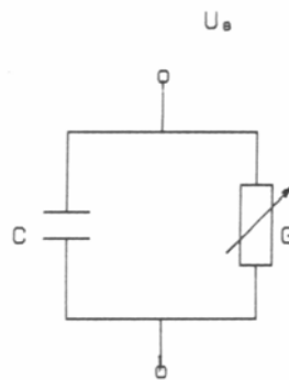
Σχήμα A2.3.2.1-2 : Ισοδύναμο κύκλωμα του στερεού μονωτικού λόγω αύξησης των απωλειών Joule.
