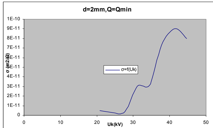
Σχήμα Β 2.10.13 Μεταβολή Ειδικής Αγωγιμότητας σε συνάρτηση με την Κρουστική Τάση
