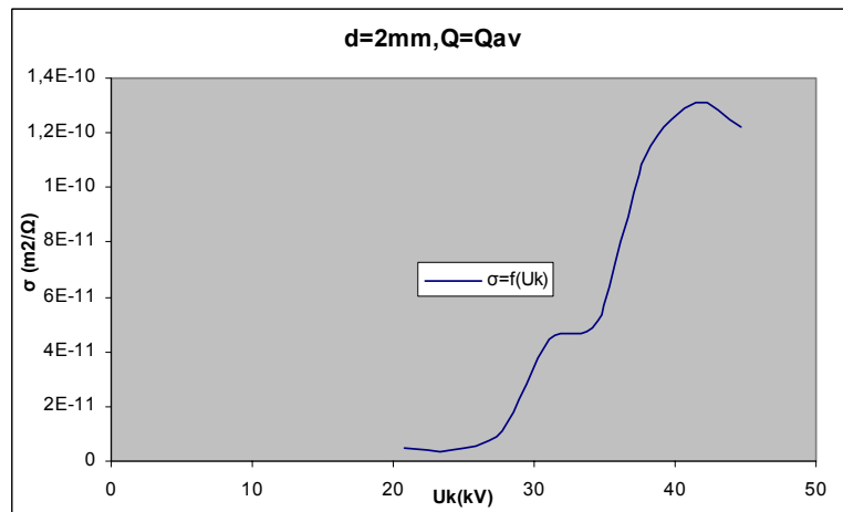
Σχήμα B 2.3.13 Μεταβολή Ειδικής Αγωγιμότητας σε συνάρτηση με την Κρουστική Τάση
