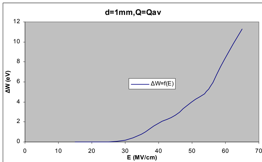
Σχήμα Β 2.1.4 Μεταβολή Ενέργειας Η/Μ Ακτινοβολίας σε συνάρτηση με την Ένταση του Ηλεκτρικού Πεδίου
