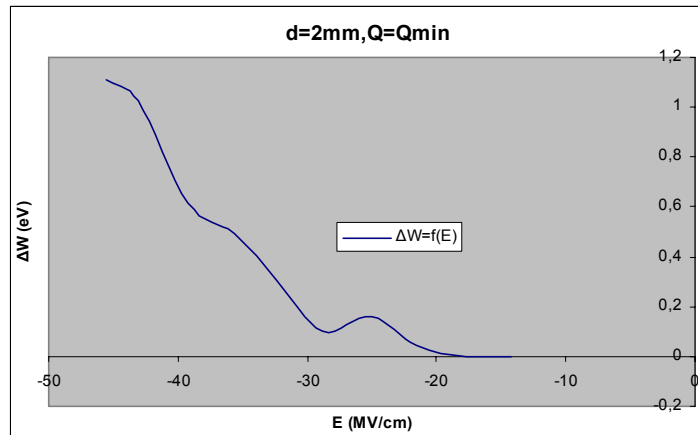
Σχήμα Β 2.12.4 Μεταβολή Ενέργειας Η/Μ Ακτινοβολίας σε συνάρτηση με την Ένταση του Ηλεκτρικού Πεδίου
