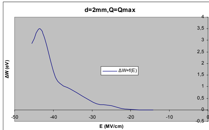
Σχήμα Β 2.11.4 Μεταβολή Ενέργειας Η/Μ Ακτινοβολίας σε συνάρτηση με την Ένταση του Ηλεκτρικού Πεδίου
