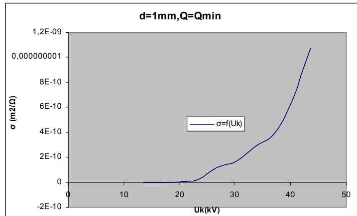
Σχήμα B 2.6.13 Μεταβολή Ειδικής Αγωγιμότητας σε συνάρτηση με την Κρουστική Τάση
