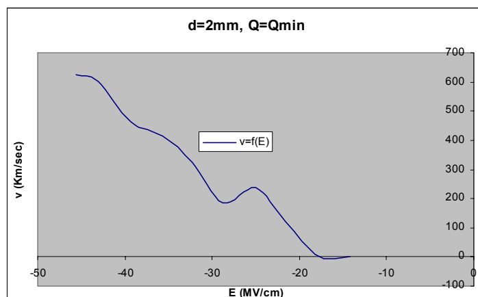
Σχήμα Β 2.12.6 Μεταβολή Ταχύτητας Ηλεκτρονίων σε συνάρτηση με την Ένταση του Ηλεκτρικού Πεδίου
