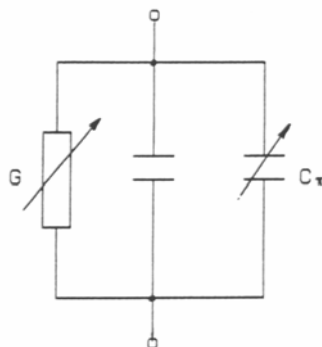
Σχήμα A2.3.2.2-2: Ισοδύναμο κύκλωμα του στερεού μονωτικού κατά την ηλεκτρική διάτρηση.
