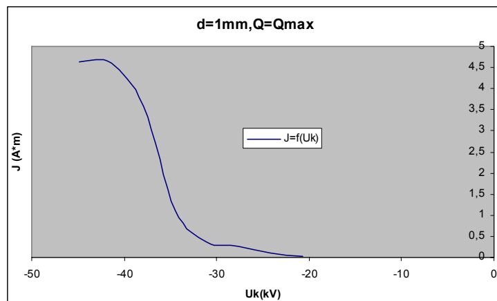
Σχήμα Β 2.7.15 Μεταβολή Πυκνότητας Ρεύματος σε συνάρτηση με την Κρουστική Τάση
