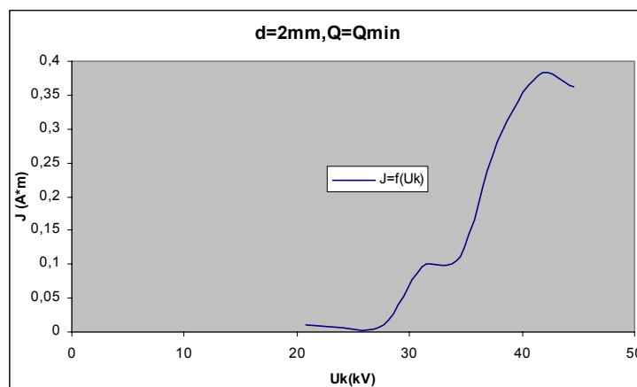
Σχήμα Β 2.10.15 Μεταβολή Πυκνότητας Ρεύματος σε συνάρτηση με την Κρουστική Τάση
