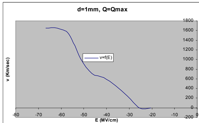
Σχήμα B 2.7.6 Μεταβολή Ταχύτητας Ηλεκτρονίων σε συνάρτηση με την Ένταση του Ηλεκτρικού Πεδίου
