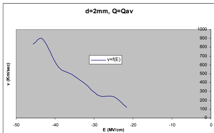
Σχήμα B 2.4.6 Μεταβολή Ταχύτητας Ηλεκτρονίων σε συνάρτηση με την Ένταση του Ηλεκτρικού Πεδίου
