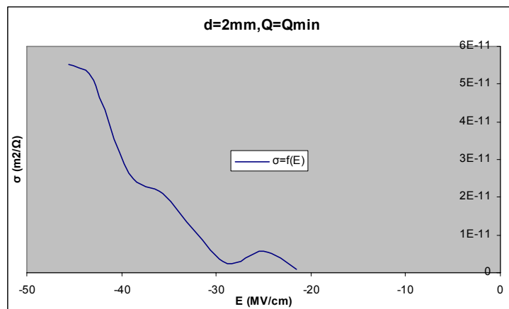
Σχήμα Β 2.12.14 Μεταβολή Ειδικής Αγωγιμότητας σε συνάρτηση με την Ένταση του Ηλεκτρικού Πεδίου
