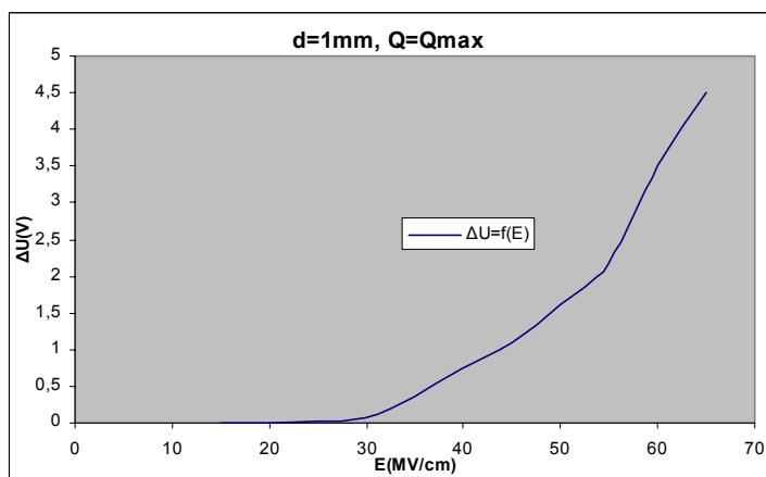
Σχήμα B 2.5.2 Μεταβολή Άλματος Δυναμικού σε συνάρτηση με την Ένταση του Ηλεκτρικού Πεδίου
