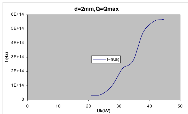
Σχήμα Β 2.9.11 Μεταβολή Συχνότητας σε συνάρτηση με την Κρουστική Τάση
