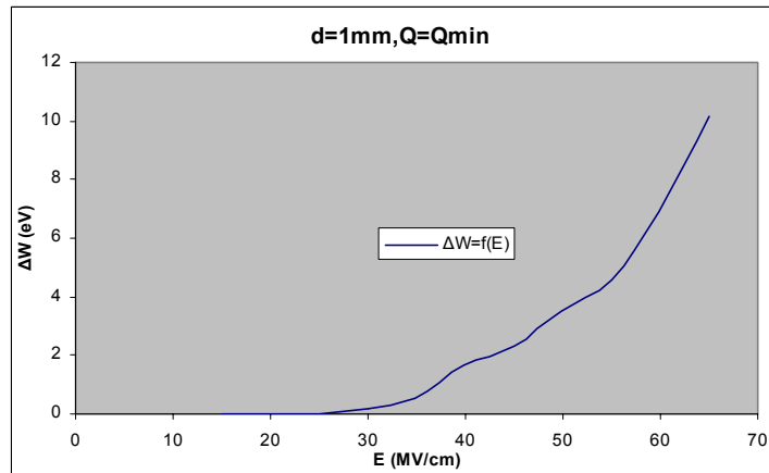
Σχήμα Β 2.6.4 Μεταβολή Ενέργειας Η/Μ Ακτινοβολίας σε συνάρτηση με την Ένταση του Ηλεκτρικού Πεδίου
