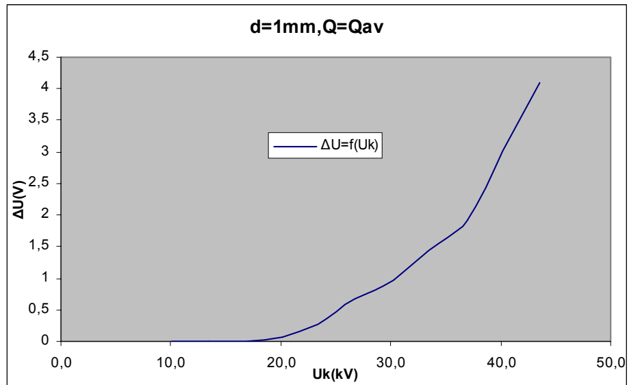
Σχήμα B 2.1.1 Μεταβολή Άλματος Δυναμικού σε συνάρτηση με την Κρουστική Τάση
