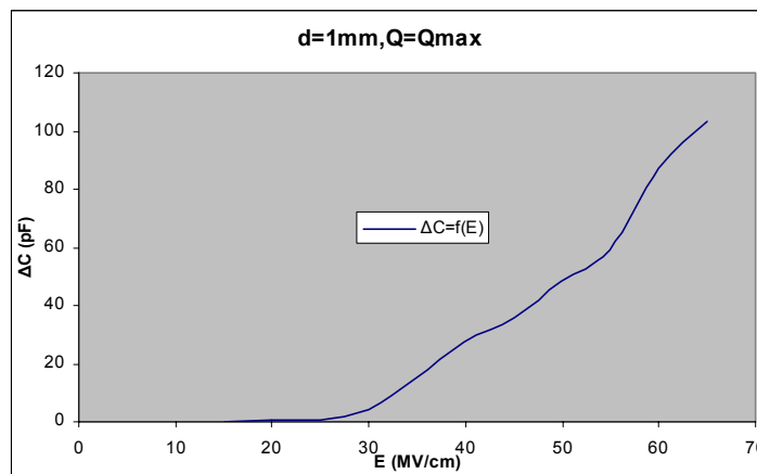
Σχήμα B 2.5.8 Μεταβολή Χωρητικότητας σε συνάρτηση με την Ένταση του Ηλεκτρικού Πεδίου
