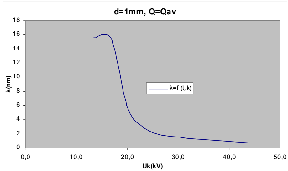
Σχήμα Β 2.1.9 Μεταβολή Μήκους Κύματος Ακτινοβολίας σε συνάρτηση με την Κρουστική Τάση
