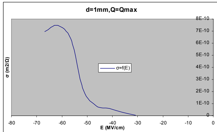
Σχήμα Β 2.7.14 Μεταβολή Ειδικής Αγωγιμότητας σε συνάρτηση με την Ένταση του Ηλεκτρικού Πεδίου
