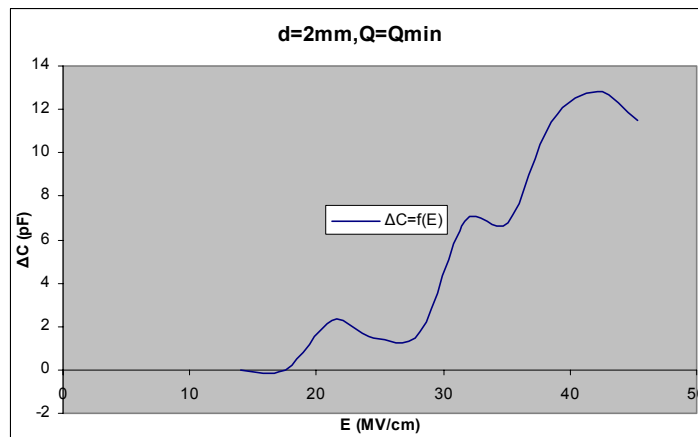
Σχήμα Β 2.10.8 Μεταβολή Χωρητικότητας σε συνάρτηση με την Ένταση του Ηλεκτρικού Πεδίου
