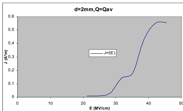
Σχήμα Β 2.3.15 Μεταβολή Πυκνότητας Ρεύματος σε συνάρτηση με την Κρουστική Τάση
