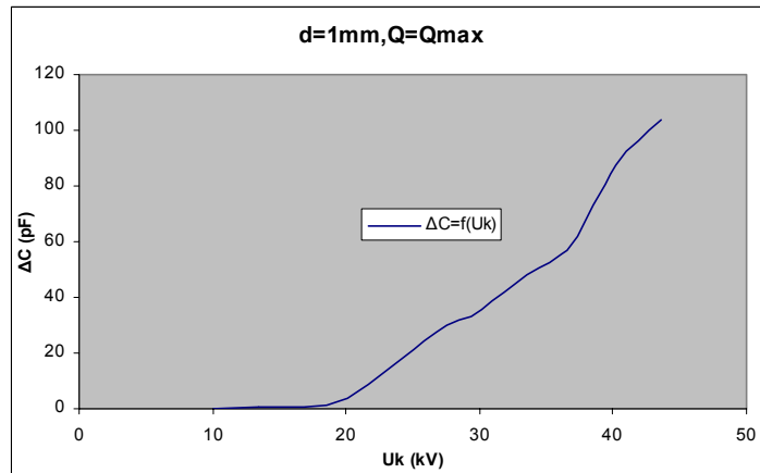
Σχήμα B 2.5.7 Μεταβολή Χωρητικότητας σε συνάρτηση με την Κρουστική Τάση
