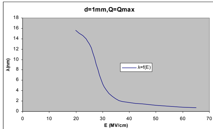
Σχήμα Β 2.5.10 Μεταβολή Μήκους Κύματος σε συνάρτηση με την Ένταση του Ηλεκτρικού Πεδίου
