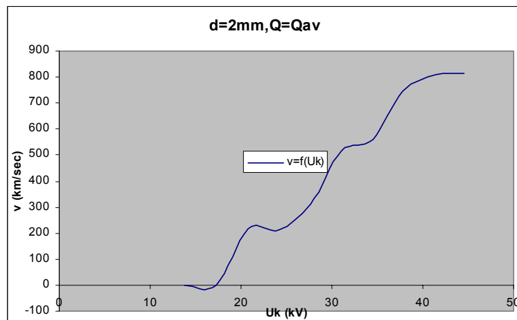
Σχήμα Β 2.3.5 Μεταβολή Ταχύτητας Ηλεκτρονίων σε συνάρτηση με την Κρουστική Τάση
