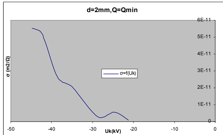
Σχήμα Β 2.12.13 Μεταβολή Ειδικής Αγωγιμότητας σε συνάρτηση με την Κρουστική Τάση
