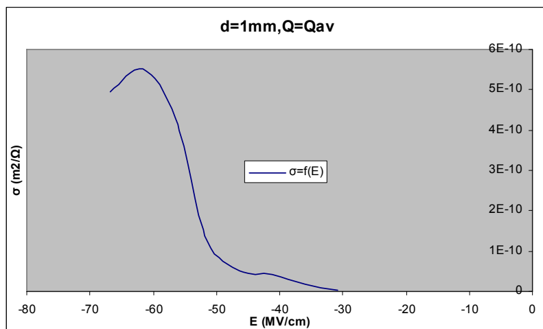
Σχήμα Β 2.2.14 Μεταβολή Ειδικής Αγωγιμότητας σε συνάρτηση με την Ένταση του Ηλεκτρικού Πεδίου
