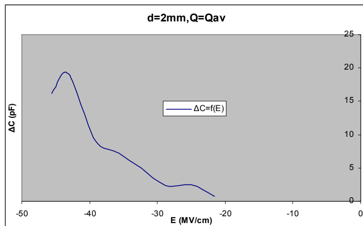
Σχήμα Β 2.4.8 Μεταβολή Χωρητικότητας σε συνάρτηση με την Ένταση του Ηλεκτρικού Πεδίου
