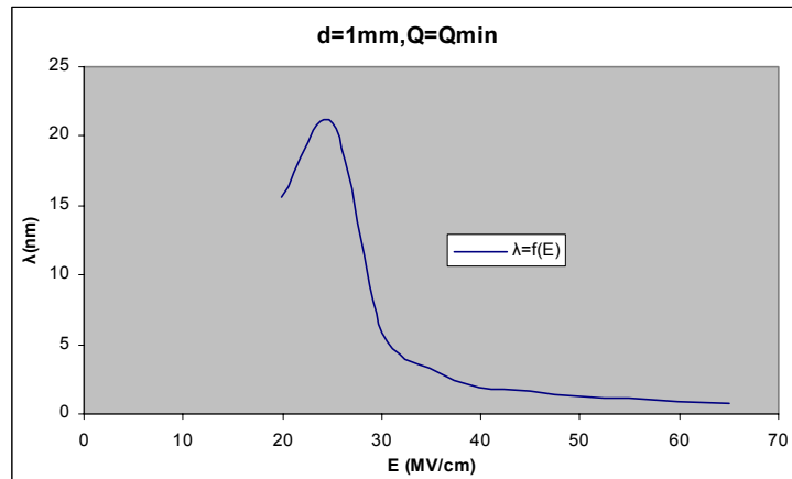
Σχήμα Β 2.6.10 Μεταβολή Μήκους Κύματος σε συνάρτηση με την Ένταση του Ηλεκτρικού Πεδίου
