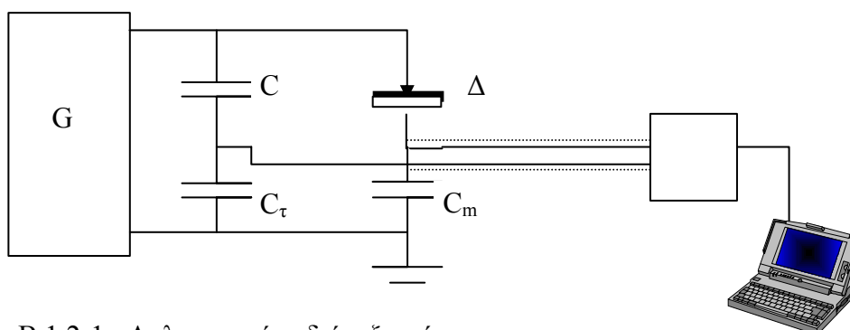
Σχήμα Β 1.2-1 : Απλοποιημένη διάταξη μέτρησης
