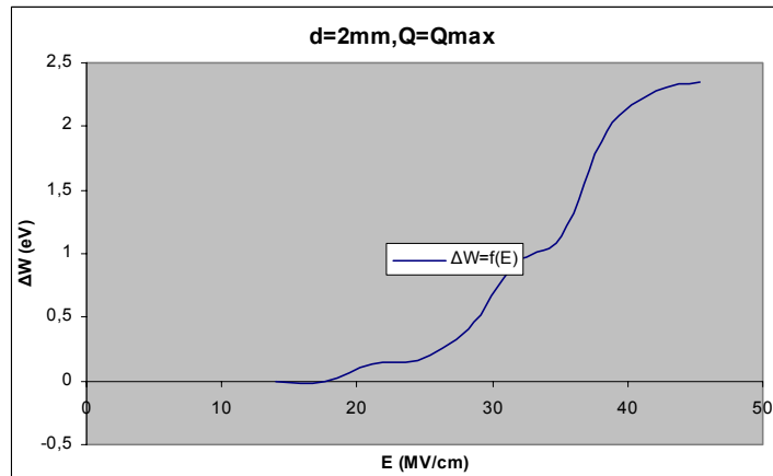
Σχήμα Β 2.9.4 Μεταβολή Ενέργειας Η/Μ Ακτινοβολίας σε συνάρτηση με την Ένταση του Ηλεκτρικού Πεδίου
