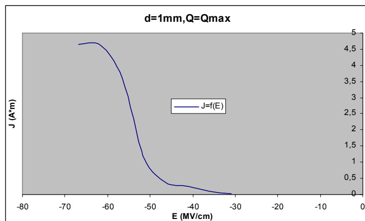
Σχήμα Β 2.7.16 Μεταβολή Πυκνότητας Ρεύματος σε συνάρτηση με την Ένταση του Ηλεκτρικού Πεδίου
