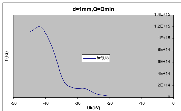
Σχήμα Β 2.8.11 Μεταβολή Συχνότητας σε συνάρτηση με την Κρουστική Τάση
