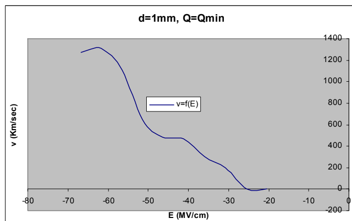
Σχήμα Β 2.8.6 Μεταβολή Ταχύτητας Ηλεκτρονίων σε συνάρτηση με την Ένταση του Ηλεκτρικού Πεδίου
