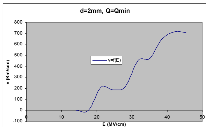
Σχήμα Β 2.10.6 Μεταβολή Ταχύτητας Ηλεκτρονίων σε συνάρτηση με την Ένταση του Ηλεκτρικού Πεδίου
