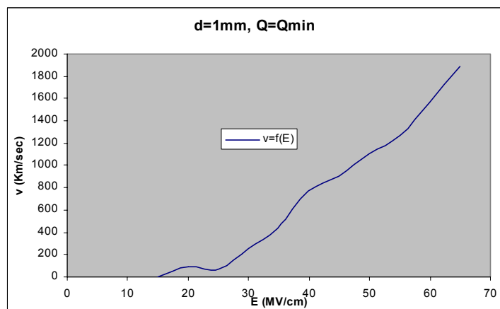
Σχήμα Β 2.6.6 Μεταβολή Ταχύτητας Ηλεκτρονίων σε συνάρτηση με την Ένταση του Ηλεκτρικού Πεδίου
