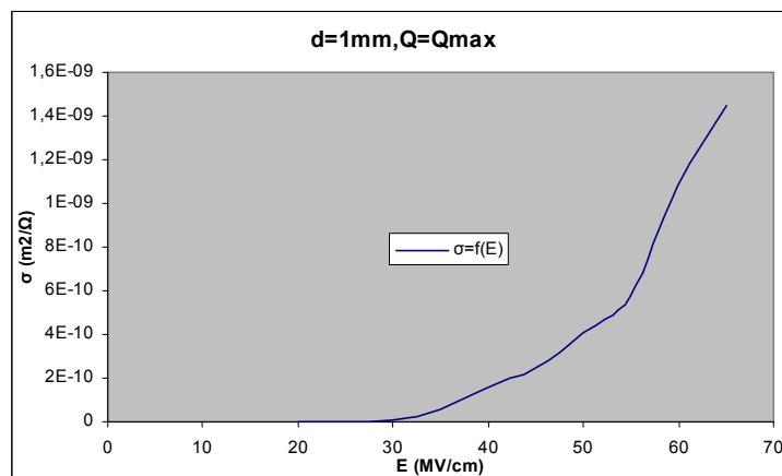
Σχήμα Β 2.5.14 Μεταβολή Ειδικής Αγωγιμότητας σε συνάρτηση με την Ένταση του Ηλεκτρικού Πεδίου
