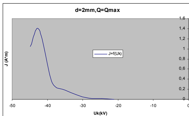
Σχήμα B 2.11.15 Μεταβολή Πυκνότητας Ρεύματος σε συνάρτηση με την Κρουστική Τάση
