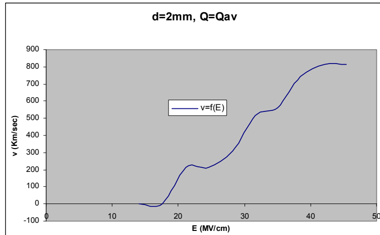
Σχήμα Β 2.3.6 Μεταβολή Ταχύτητας Ηλεκτρονίων σε συνάρτηση με την Ένταση του Ηλεκτρικού Πεδίου
