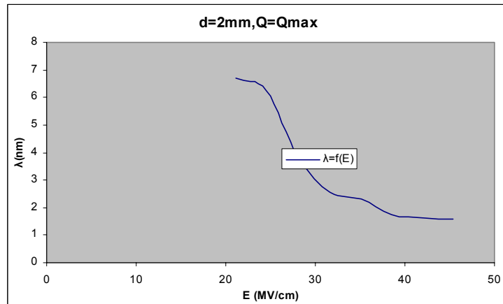
Σχήμα Β 2.9.10 Μεταβολή Μήκους Κύματος σε συνάρτηση με την Ένταση του Ηλεκτρικού Πεδίου
