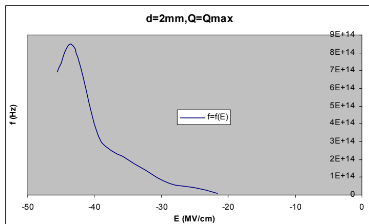
Σχήμα Β 2.11.12 Μεταβολή Συχνότητας σε συνάρτηση με την Ένταση του Ηλεκτρικού Πεδίου
