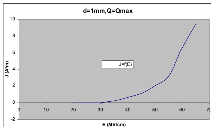
Σχήμα Β 2.5.16 Μεταβολή Πυκνότητας Ρεύματος σε συνάρτηση με την Ένταση του Ηλεκτρικού Πεδίου
