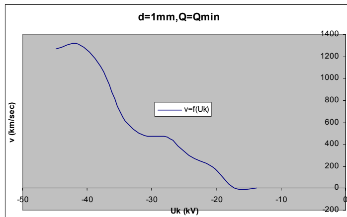
Σχήμα Β 2.8.5 Μεταβολή Ταχύτητας Ηλεκτρονίων σε συνάρτηση με την Κρουστική Τάση
