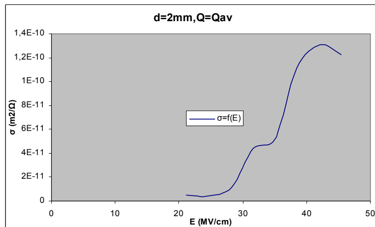
Σχήμα B 2.3.14 Μεταβολή Ειδικής Αγωγιμότητας σε συνάρτηση με την Ένταση του Ηλεκτρικού Πεδίου
