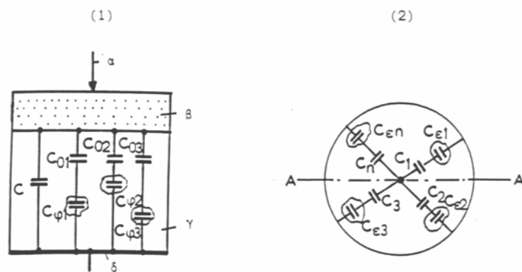
Σχήμα A2.3.2.3-1: Μία μακροσκοπική παράσταση των θέσεων διαταραχής σε στερεό μονωτικό εντός μονωτικού ελαίου
