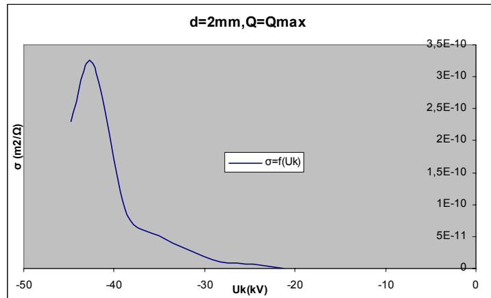
Σχήμα B 2.11.13 Μεταβολή Ειδικής Αγωγιμότητας σε συνάρτηση με την Κρουστική Τάση
