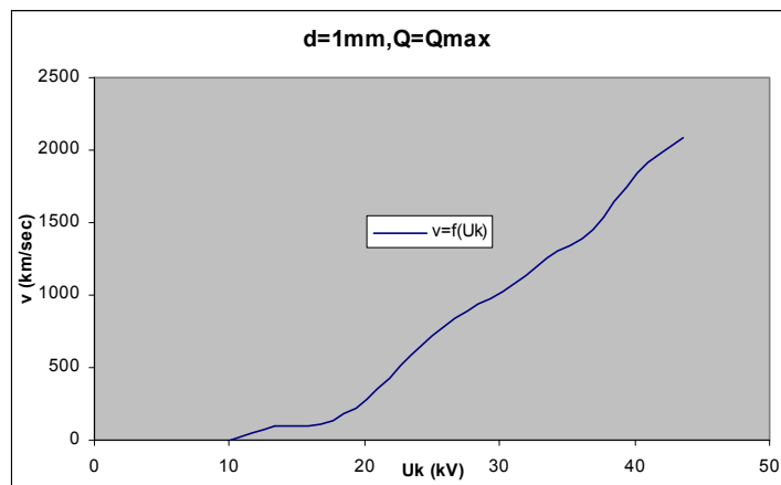
Σχήμα Β 2.5.5 Μεταβολή Ταχύτητας Ηλεκτρονίων σε συνάρτηση με την Κρουστική Τάση
