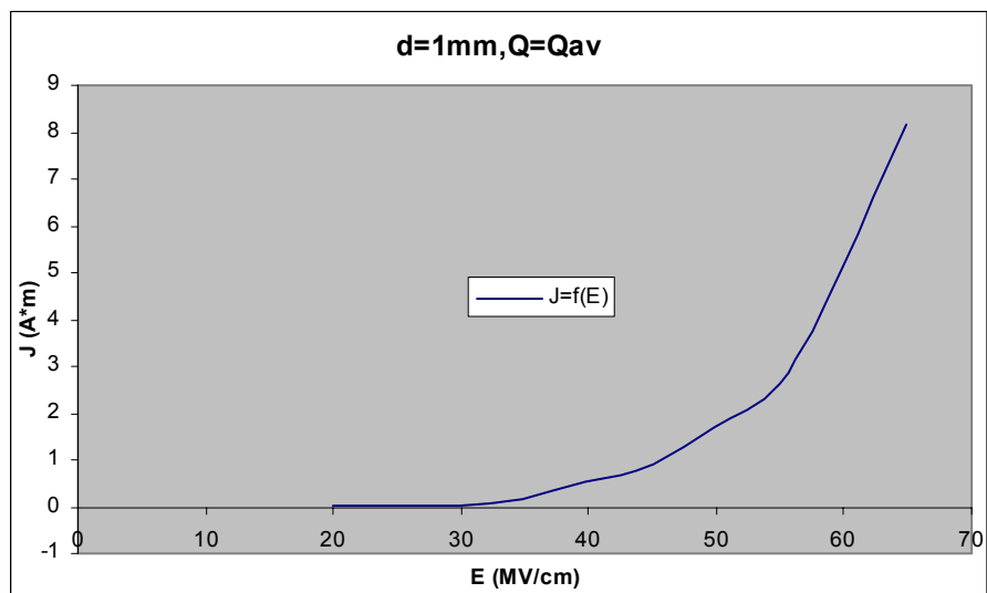
Σχήμα B 2.1.16 Μεταβολή Πυκνότητας Ρεύματος σε συνάρτηση με την Ένταση του Ηλεκτρικού Πεδίου
