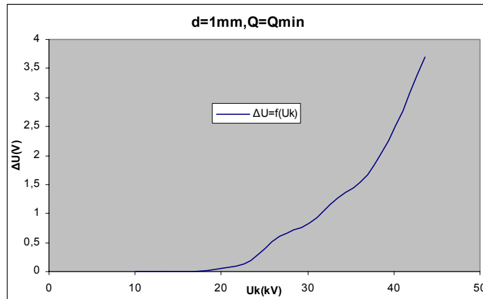
Σχήμα B 2.6.1 Μεταβολή Άλματος Δυναμικού σε συνάρτηση με την Κρουστική Τάση
