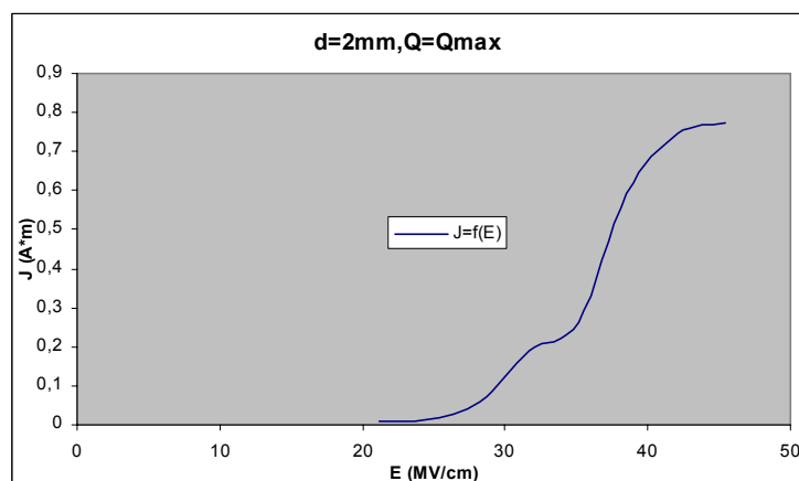
Σχήμα Β 2.9.16 Μεταβολή Πυκνότητας Ρεύματος σε συνάρτηση με την Ένταση του Ηλεκτρικού Πεδίου
