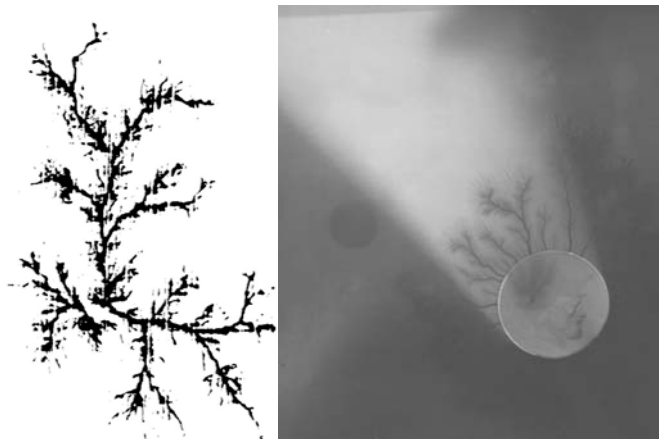
Σχήμα 2.3.5-3 : Φωτογράφιση ενός εικοσάδραχμου κατά την επιφανειακή διάσπαση στον αέρα πολυμερών στερεών μονωτικών υπό κρουστική τάση 1,2/50μs (διάταξη ηλεκτροδίων ακίδα-πλάκα).
