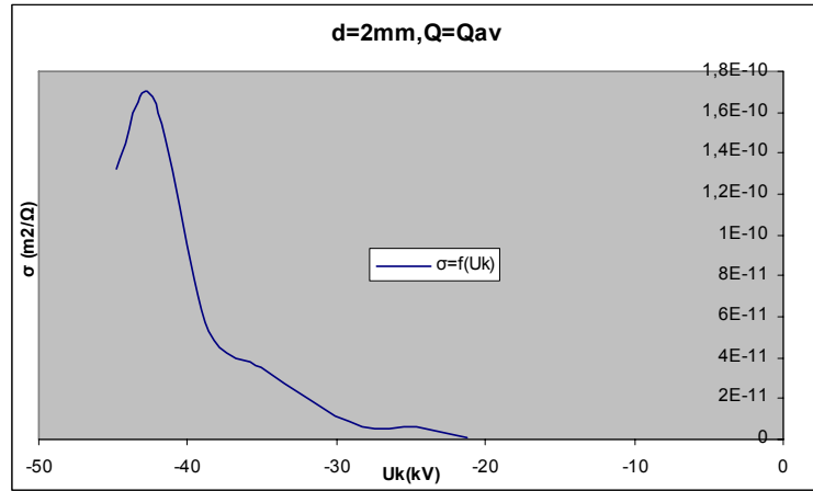
Σχήμα Β 2.4.13 Μεταβολή Ειδικής Αγωγιμότητας σε συνάρτηση με την Κρουστική Τάση
