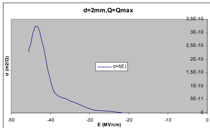
Σχήμα B 2.11.14 Μεταβολή Ειδικής Αγωγιμότητας σε συνάρτηση με την Ένταση του Ηλεκτρικού Πεδίου
