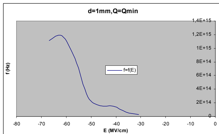
Σχήμα Β 2.8.12 Μεταβολή Συχνότητας σε συνάρτηση με την Ένταση του Ηλεκτρικού Πεδίου
