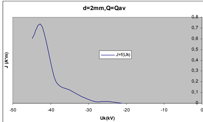
Σχήμα Β 2.4.15 Μεταβολή Πυκνότητας Ρεύματος σε συνάρτηση με την Κρουστική Τάση
