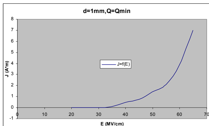
Σχήμα Β 2.6.16 Μεταβολή Πυκνότητας Ρεύματος σε συνάρτηση με την Ένταση του Ηλεκτρικού Πεδίου
