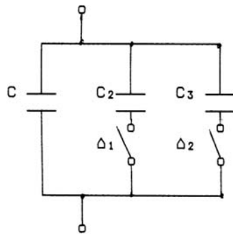
Σχήμα A2.3.2.3-5: Ισοδύναμο κύκλωμα των μερικών εκκενώσεων (παραλλαγή του ισοδύναμου κυκλώματος των Gemant και Philipoff).
