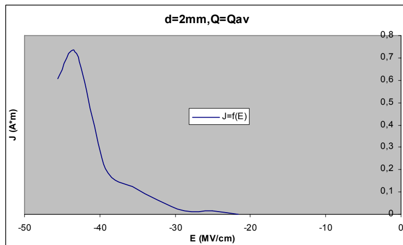
Σχήμα Β 2.4.16 Μεταβολή Πυκνότητας Ρεύματος σε συνάρτηση με την Ένταση του Ηλεκτρικού Πεδίου
