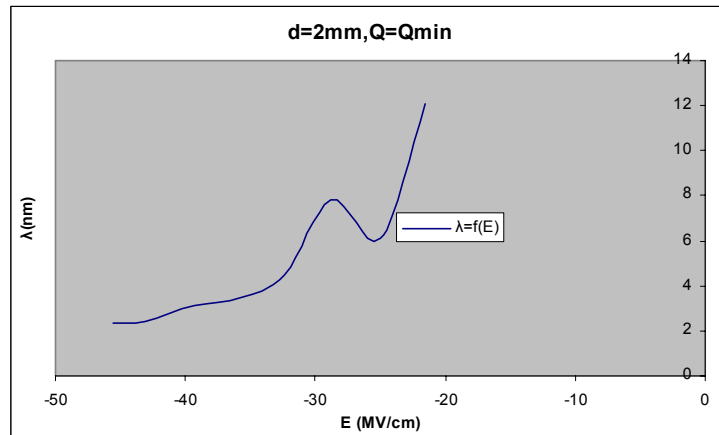
Σχήμα Β 2.12.10 Μεταβολή Μήκους Κύματος σε συνάρτηση με την Ένταση του Ηλεκτρικού Πεδίου
