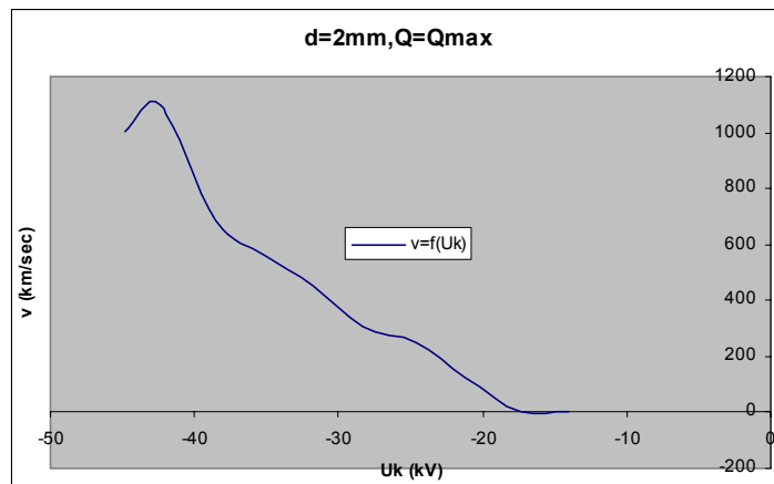
Σχήμα Β 2.11.5 Μεταβολή Ταχύτητας Ηλεκτρονίων σε συνάρτηση με την Κρουστική Τάση
