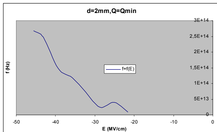
Σχήμα Β 2.12.12 Μεταβολή Συχνότητας σε συνάρτηση με την Ένταση του Ηλεκτρικού Πεδίου
