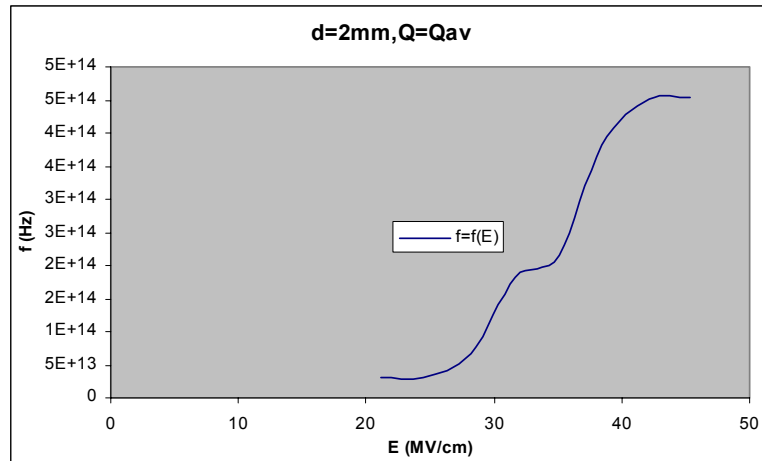
Σχήμα B 2.3.12 Μεταβολή Συχνότητας σε συνάρτηση με την Ένταση του Ηλεκτρικού Πεδίου
