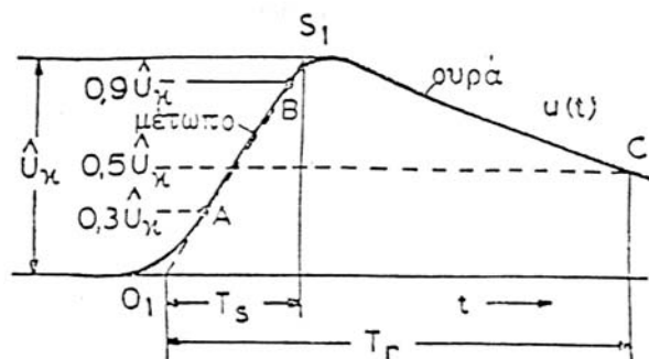
Σχήμα Α3-1: Χαρακτηρισμός των μεγεθών μίας κρουστικής τάσης.
