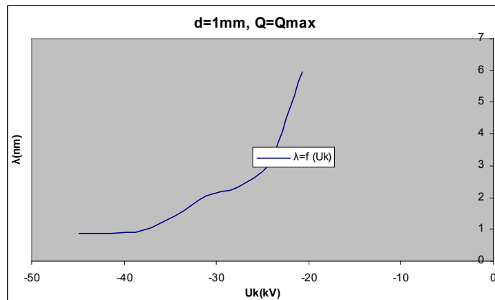
Σχήμα Β 2.7.9 Μεταβολή Μήκους Κύματος σε συνάρτηση με την Κρουστική Τάση
