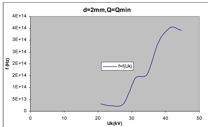
Σχήμα Β 2.10.11 Μεταβολή Συχνότητας σε συνάρτηση με την Κρουστική Τάση
