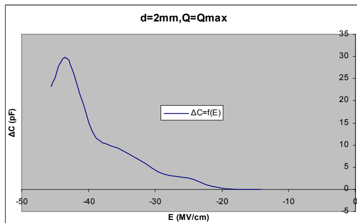
Σχήμα Β 2.11.8 Μεταβολή Χωρητικότητας σε συνάρτηση με την Ένταση του Ηλεκτρικού Πεδίου
