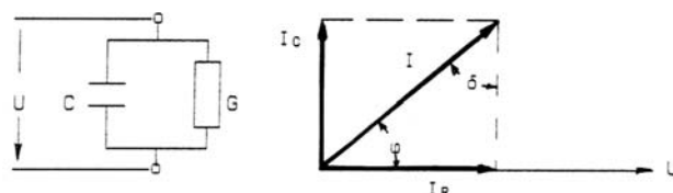
Σχήμα Α1.3-2 : Ισοδύναμο κύκλωμα ενός πυκνωτή C με απώλειες λόγω της αγωγιμότητας G του διηλεκτρικού του.
