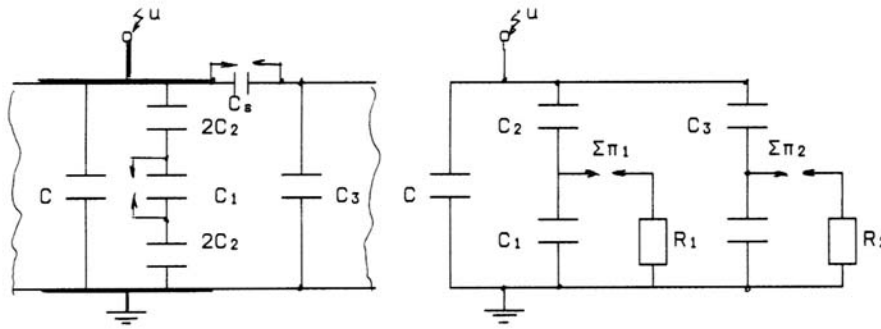
Σχήμα A2.3.2.3-4: Σχηματική παράσταση και ισοδύναμο κύκλωμα ενός στερεού μονωτικού με φυσαλίδα αερίου στον όγκο του και με επιφανειακή θέση διαταραχής.
