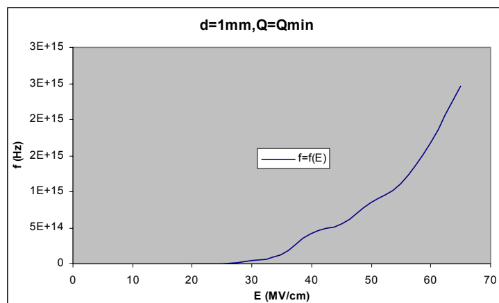
Σχήμα Β 2.6.12 Μεταβολή Συχνότητας σε συνάρτηση με την Ένταση του Ηλεκτρικού Πεδίου
