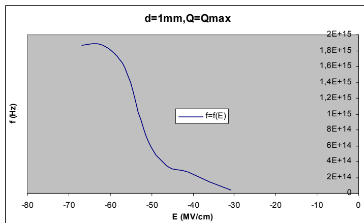
Σχήμα B 2.7.12 Μεταβολή Συχνότητας σε συνάρτηση με την Ένταση του Ηλεκτρικού Πεδίου
