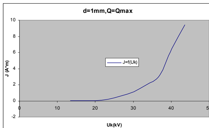
Σχήμα Β 2.5.15 Μεταβολή Πυκνότητας Ρεύματος σε συνάρτηση με την Κρουστική Τάση
