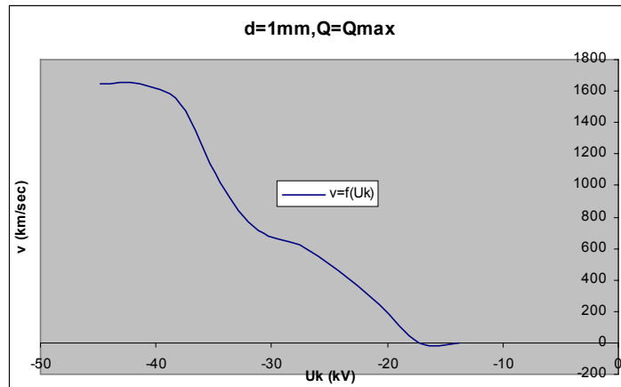
Σχήμα B 2.7.5 Μεταβολή Ταχύτητας Ηλεκτρονίων σε συνάρτηση με την Κρουστική Τάση
