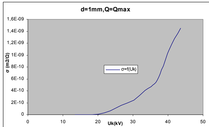
Σχήμα Β 2.5.13 Μεταβολή Ειδικής Αγωγιμότητας σε συνάρτηση με την Κρουστική Τάση
