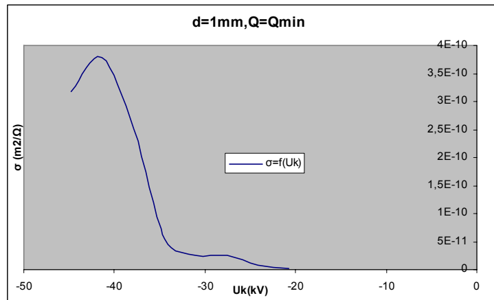
Σχήμα Β 2.8.13 Μεταβολή Ειδικής Αγωγιμότητας σε συνάρτηση με την Κρουστική Τάση
