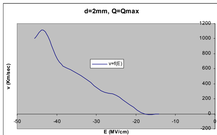
Σχήμα Β 2.11.6 Μεταβολή Ταχύτητας Ηλεκτρονίων σε συνάρτηση με την Ένταση του Ηλεκτρικού Πεδίου
