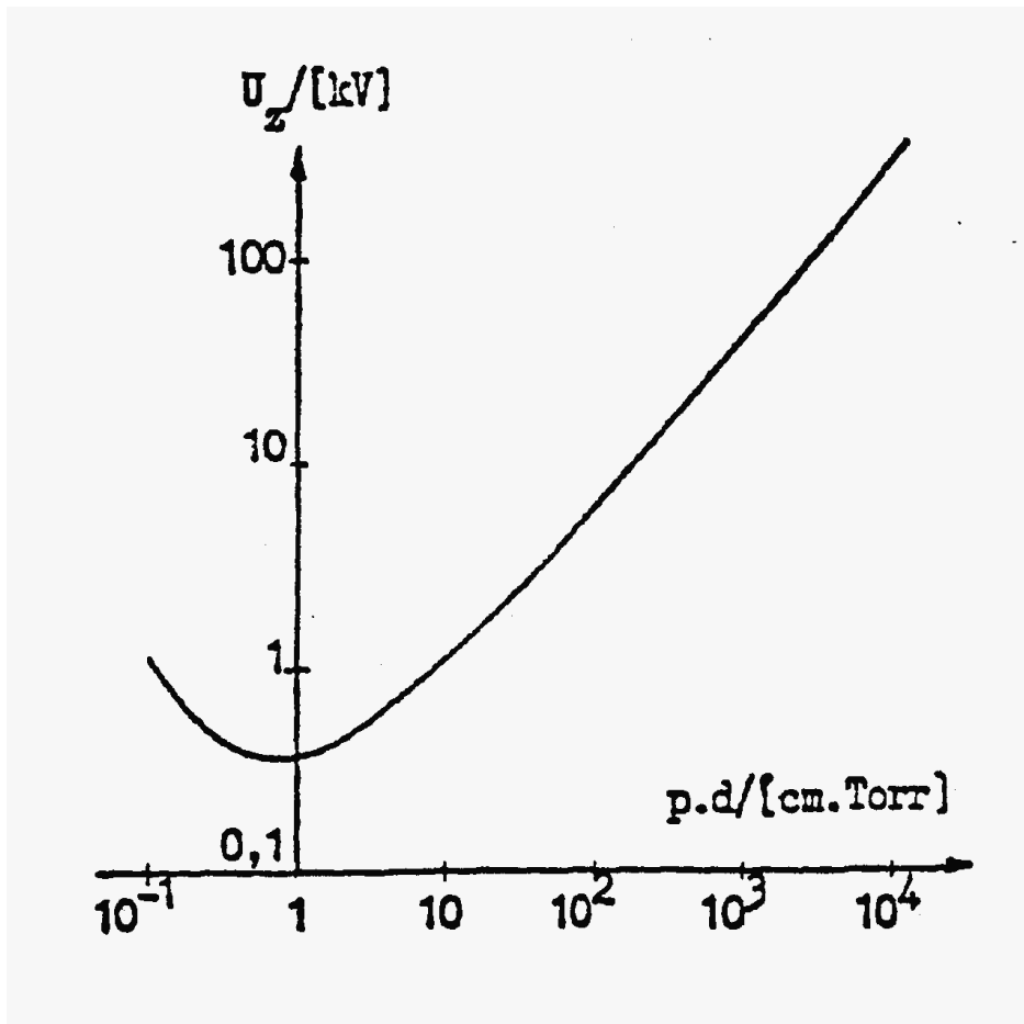
Σχήμα A2.1.1-2 : U_z = f(p \cdot d) για τον αέρα σε κανονική θερμοκρασία
