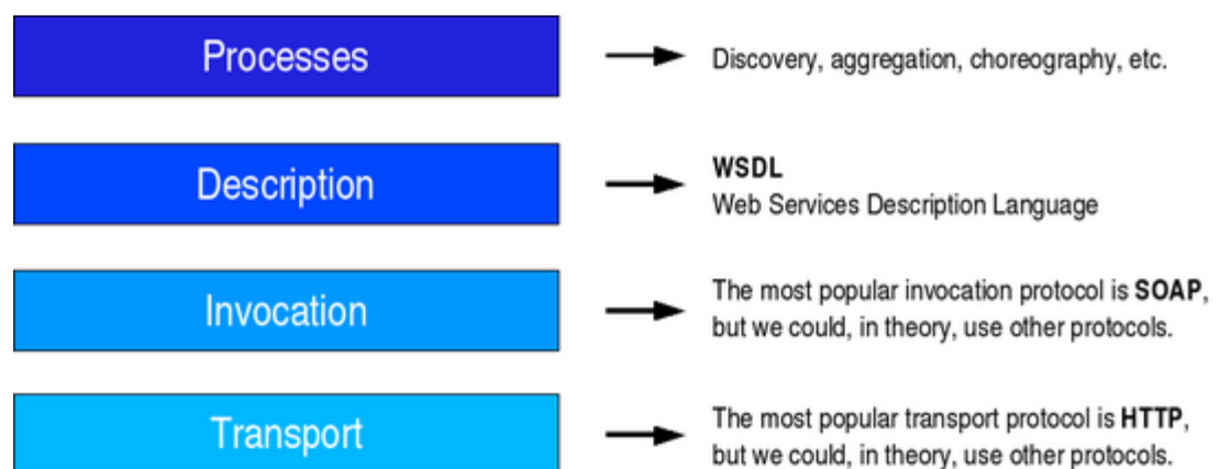
Εικόνα 3.2 Globus Toolkit 4
