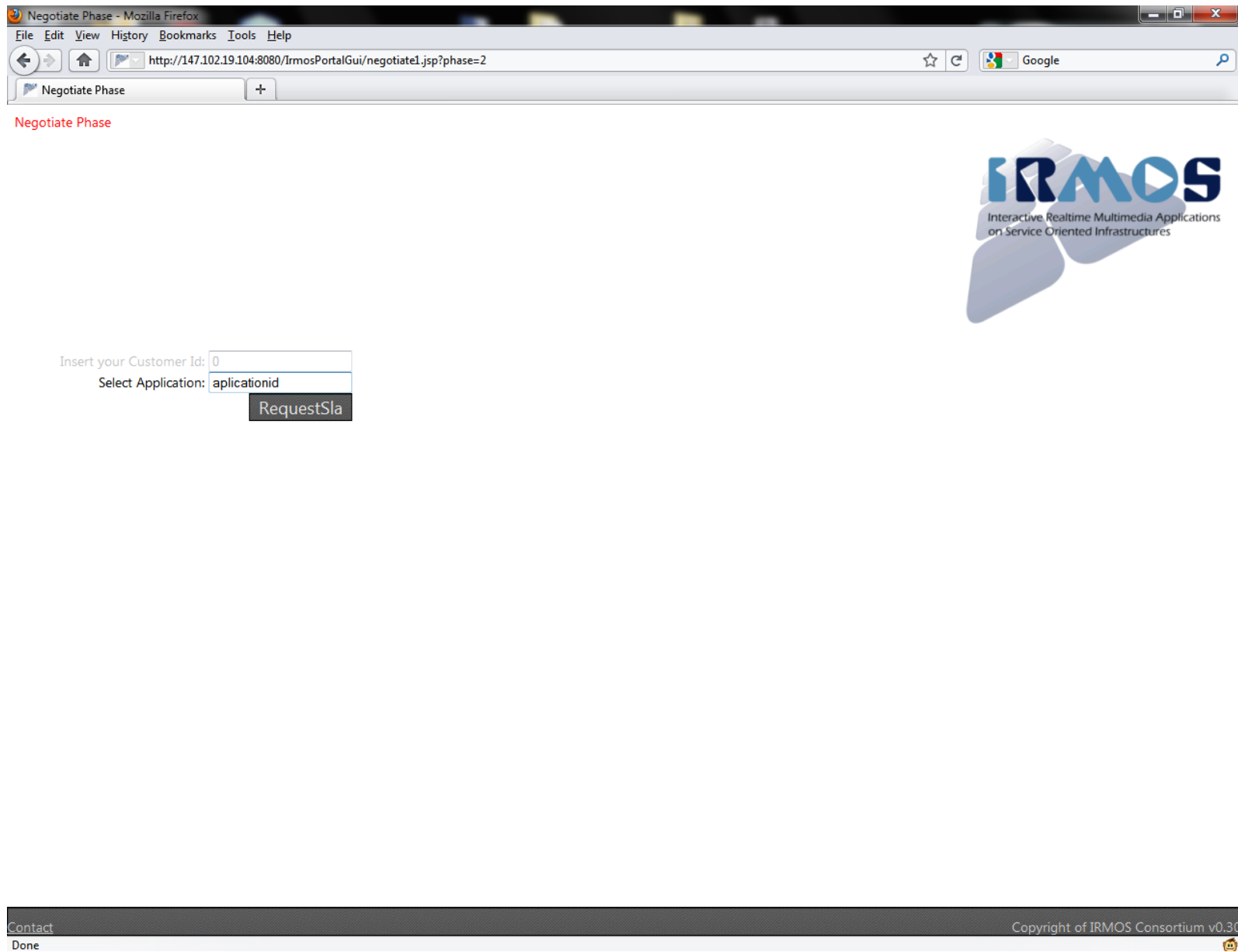
Εικόνα 8.6 Negotiation1 Phase 2
