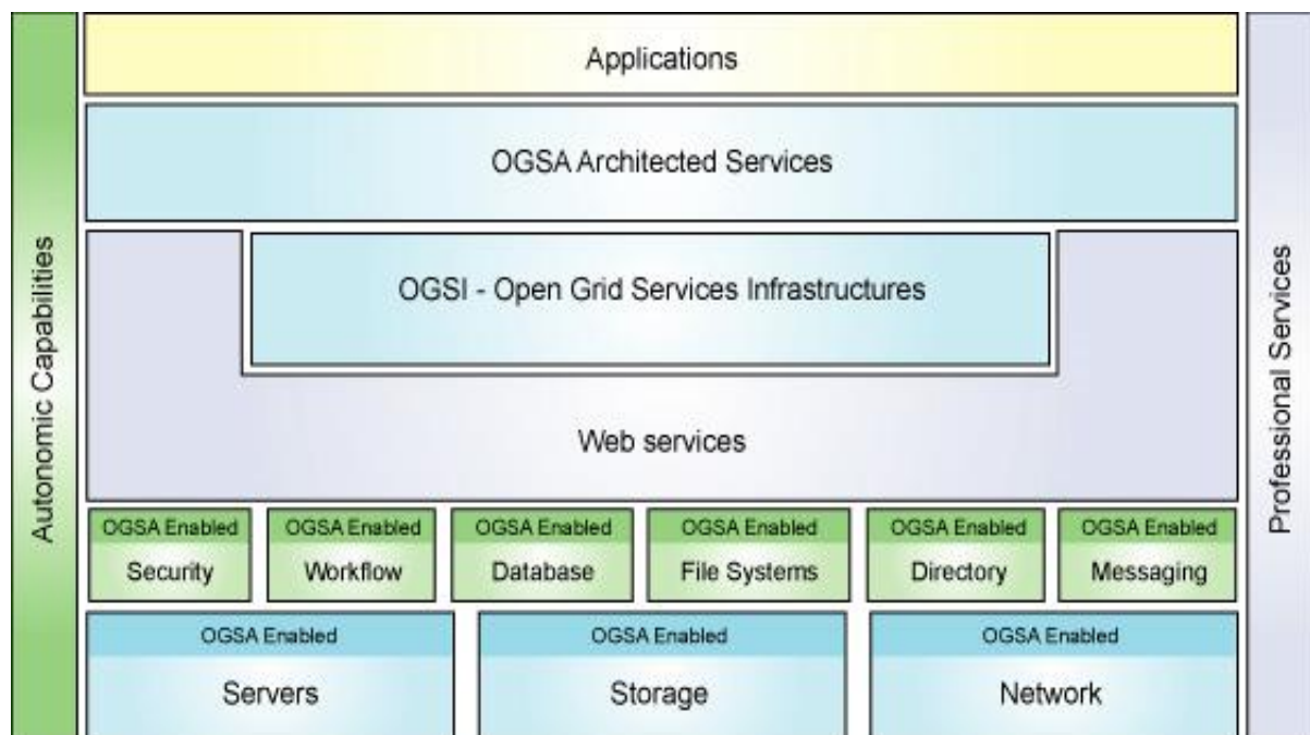
Εικόνα 2.6 : OGSA Αρχιτεκτονική
