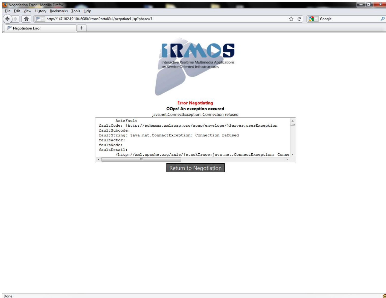
Εικόνα 8.11 Σφάλμα Negotiation
