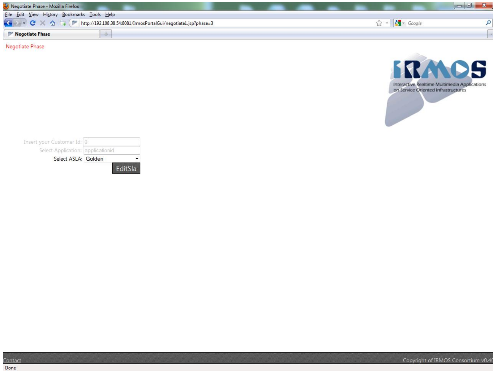
Εικόνα 8.7 Negotiate1 Phase 3
