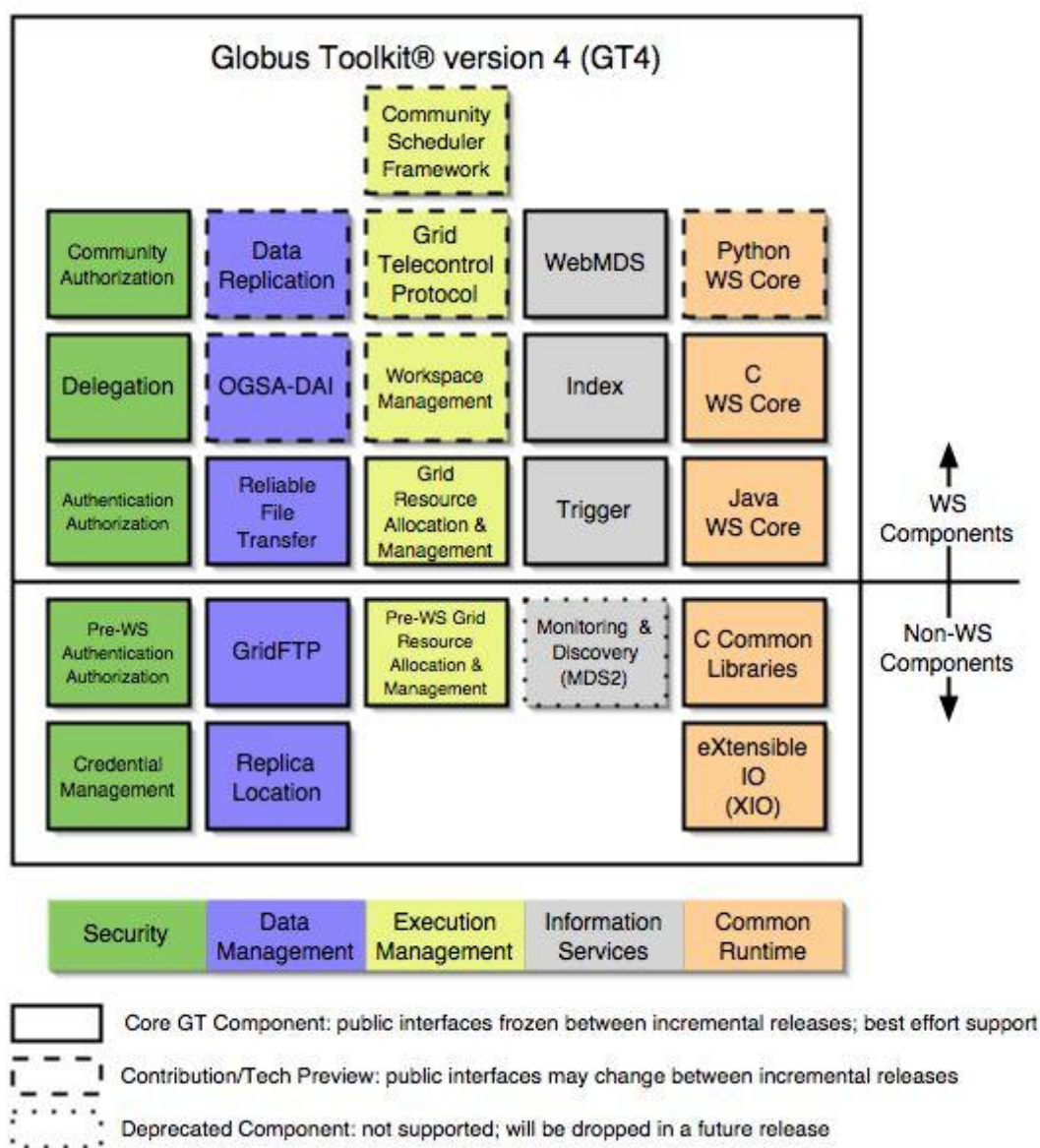
Εικόνα 4.1.7 Globus Toolkit
