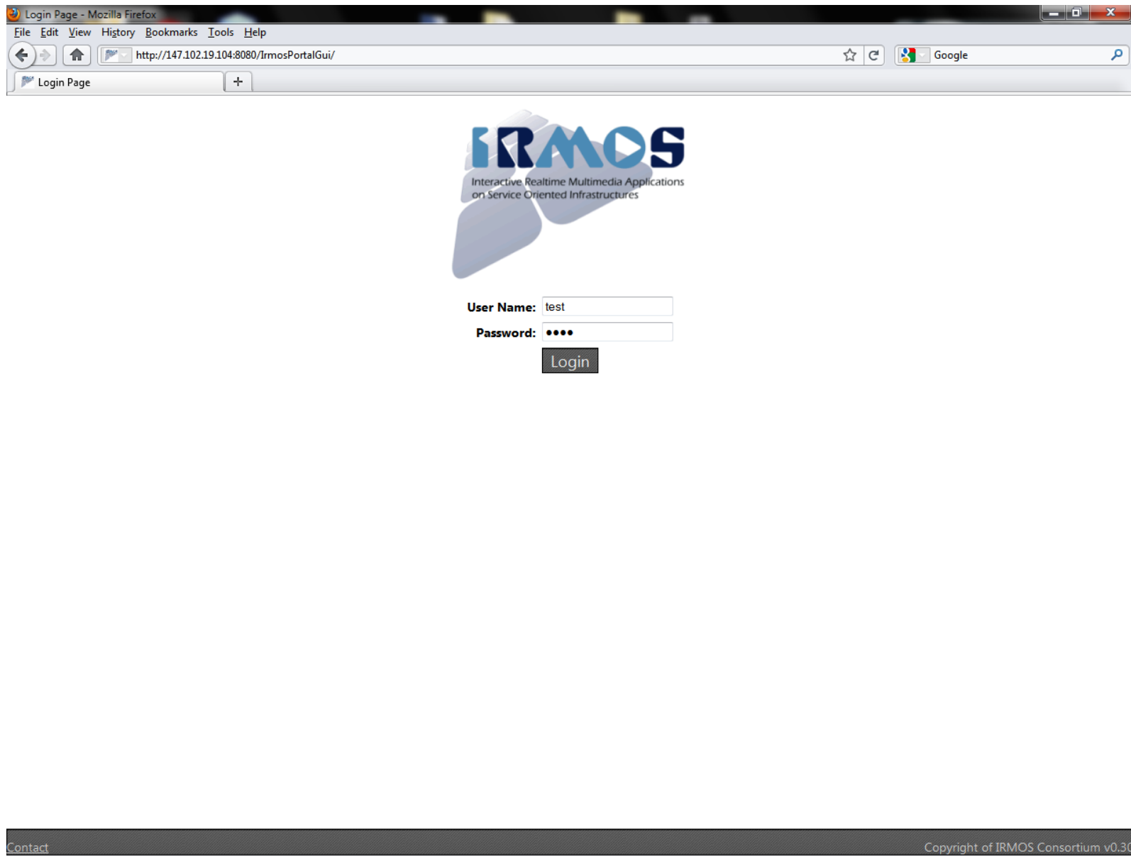
Εικόνα 8.2 Login.jsp
