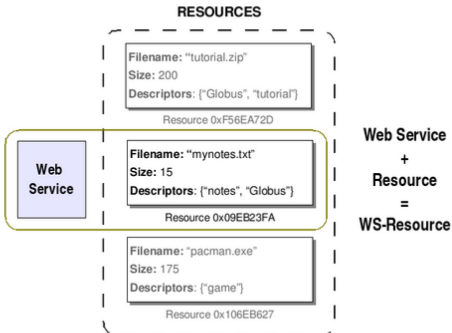
Εικόνα 4.5 WS-Resource
