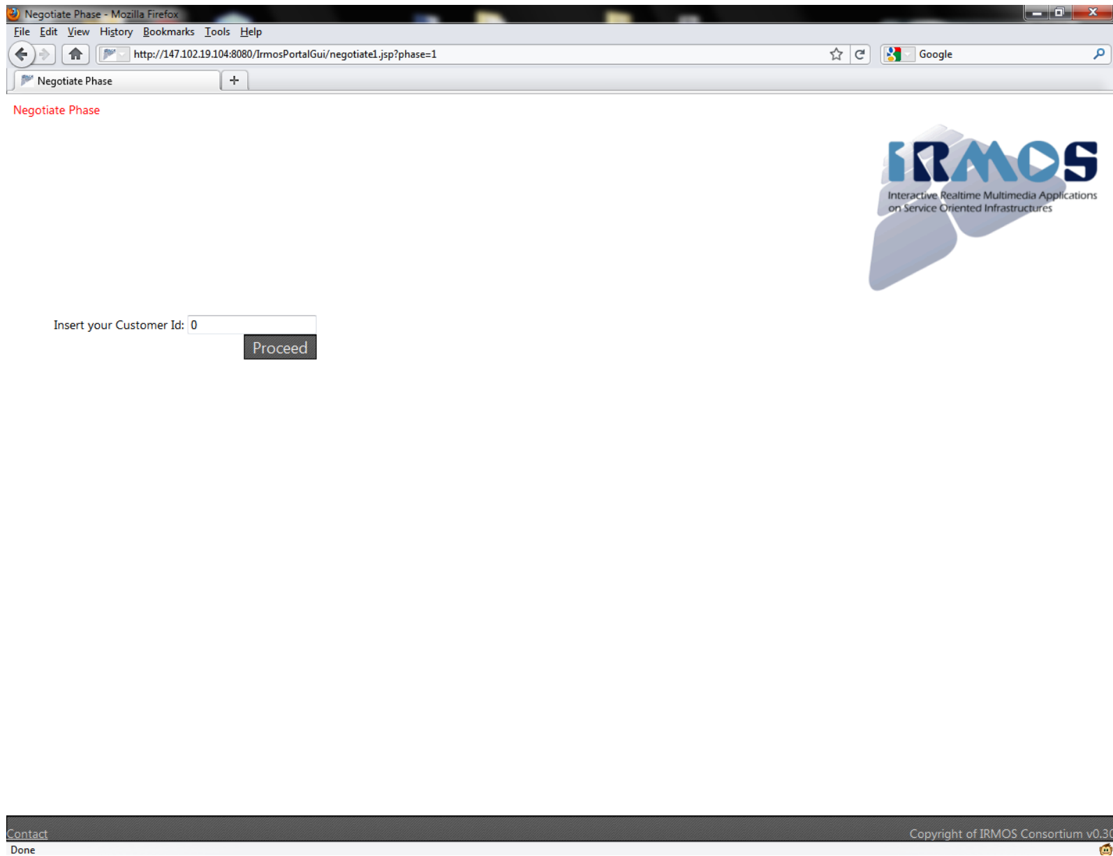
Εικόνα 8.5 Negotiate1.jsp Phase 1
