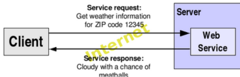
Εικόνα 3.1: Web Services
