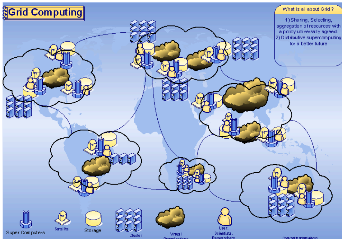
Εικόνα 1.1 Υπολογιστικό Πλέγμα
