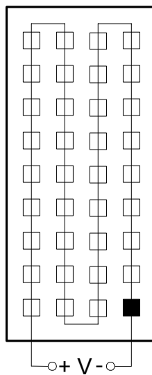
Σχήμα 21: Διάταξη φωτοβολταϊκών στοιχείων σε σειρά
