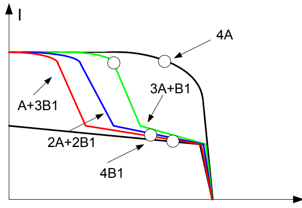
Χαρακτηριστική I-V 18 : Φωτοβολταϊκού πλαισίου συναρτήσει ενός σκιασμένου φωτοβολταϊκού στοιχείου σε μία ή περισσότερες στήλες [ 17 ]
