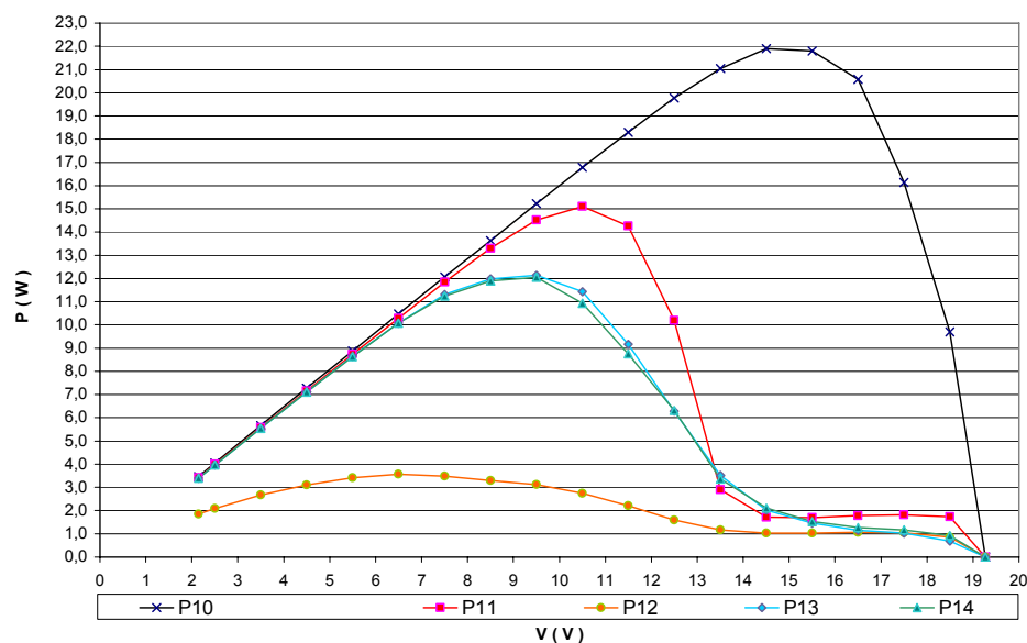
Χαρακτηριστική P-V 5 : Φωτοβολταϊκού πλαισίου με παρακαμπτήρια δίοδο στην 1 η στήλη συναρτήσεως ενός πλήρους σκιασμένου στοιχείου
