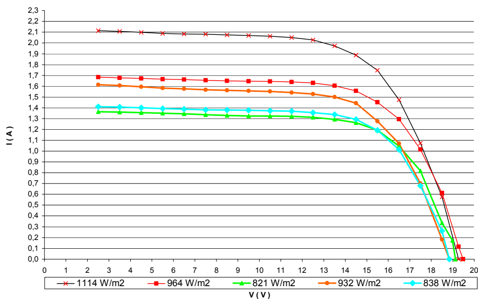
Χαρακτηριστική I-V 19 : Φωτοβολταϊκού πλαισίου συναρτήσεως της έντασης ακτινοβολίας
