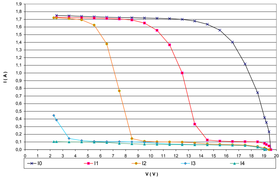
Χαρακτηριστική I-V 30 : Φωτοβολταϊκού πλαισίου με όλες τις παρακαμπτήριες διόδους συναρτηθεί ενός πλήρους σκιασμένου στοιχείου σε μία ή περισσότερες στήλες
