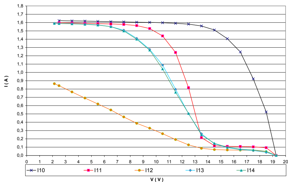
Χαρακτηριστική I-V 22 : Φωτοβολταϊκού πλαισίου με παρακαμπτήρια δίοδο στην 1 η στήλη συναρτήσεως ενός πλήρους σκιασμένου στοιχείου
