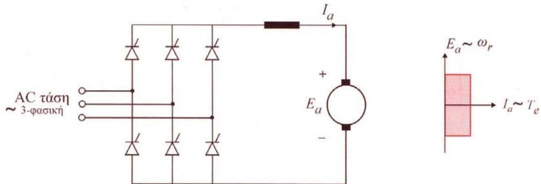
Σχήμα 1.5 Τριφασική πλήρως ελεγχόμενη ανορθωτική γέφυρα (ac-dc μετατροπέας ισχύος) για οδήγηση κινητήρα συνεχούς ρεύματος με δυνατότητα στα δυο τεταρτημόρια
