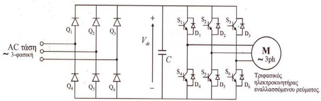
Σχήμα 1.9 Κύκλωμα ισχύος στατικού μετατροπέα συχνότητας πηγής τάσης
