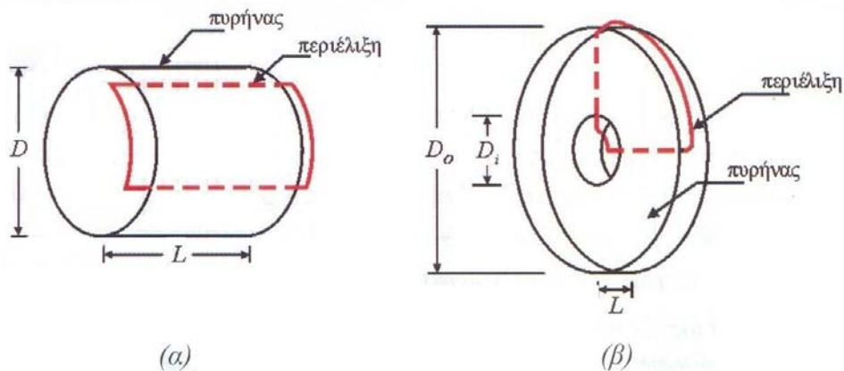
Σχήμα 2.12 Βασικός σχεδιασμός μηχανών: (α) ακτινικής, (β) αξονικής ροής
