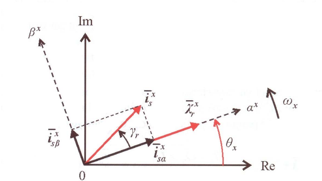
Σχήμα 3.12 Διάγραμμα των διανυσμάτων χώρου ηλεκτρικής μηχανής στο αυθαίρετο σύστημα αξόνων αναφοράς, όταν το διάνυσμα της ροής του δρομέα είναι προσανατολισμένο κατά τον οριζόντιο άξονα ( \alpha^x -άξονα)
