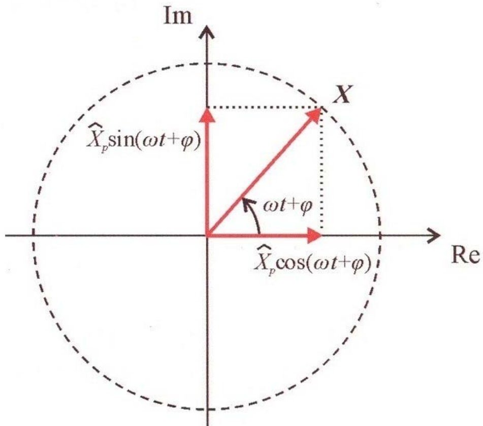
Σχήμα 3.2 Στρεφόμενα διανύσματα (α) στο πεδίο του χρόνου (β) στο πεδίο της συχνότητας
