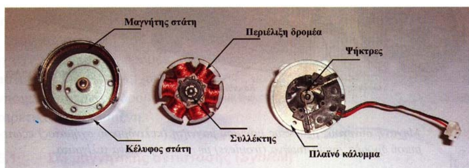
Σχήμα 2.30 Μηχανή συνεχούς ρεύματος μόνιμου μαγνήτη (δακτυλιοειδούς σχήματος) εσωτερικού δρομέα με συγκεντρωμένα τυλίγματα
