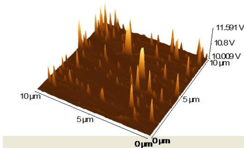
Σχήμα 6.12 : Εικόνα c-AFM δείγματος EK22
