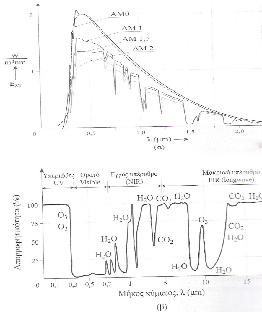
Σχήμα 3.1 (α) Φάσματα και (β) Φάσμα απορρόφησης των διαφόρων αερίων
