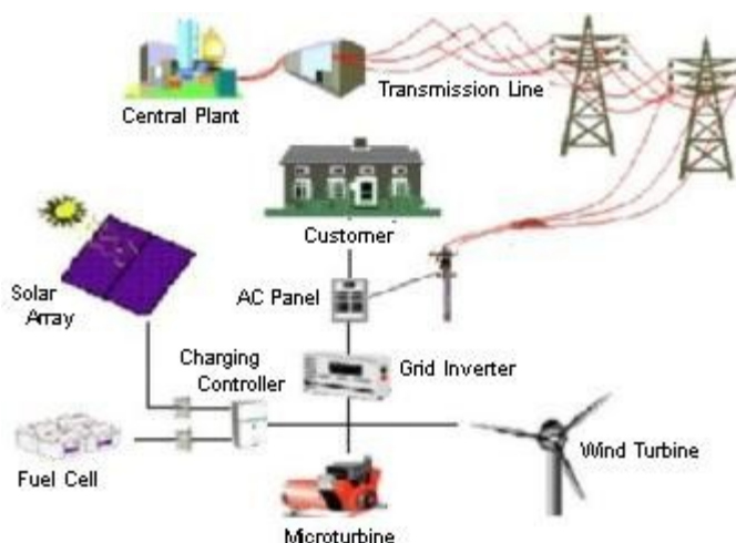
Σχήμα 2.1 Διεσπαρμένη παραγωγή
