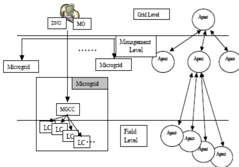
Σχήμα 6.7 Αντιστοίχιση επιπέδων ελέγχου για το μικροδίκτυο και προσέγγισης με σύστημα MAS
