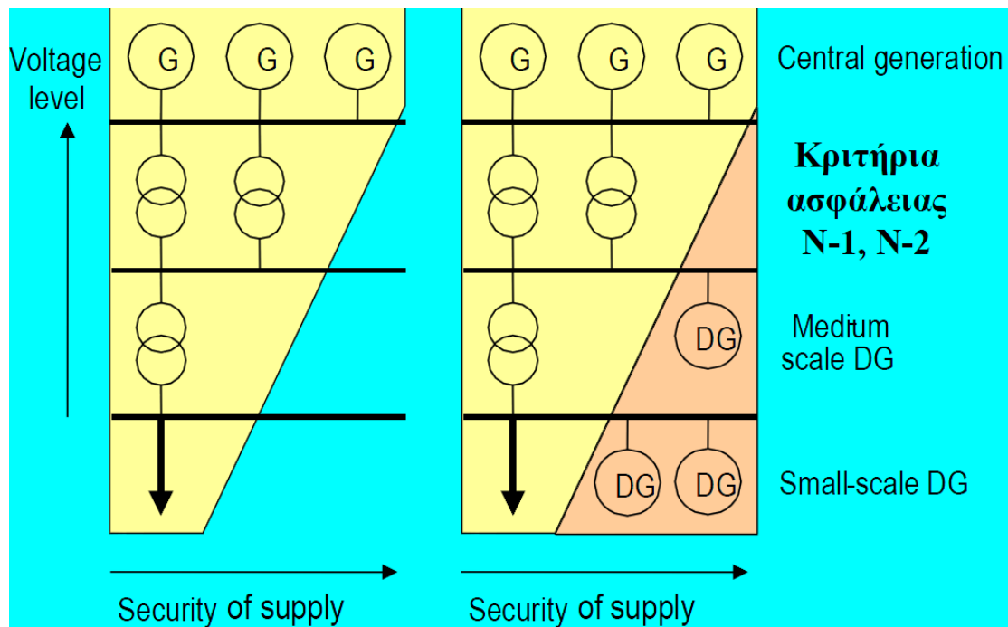
Σχήμα 2.3 Αύξηση της αξιοπιστίας παροχής από τη διεσπαρμένη παραγωγή
