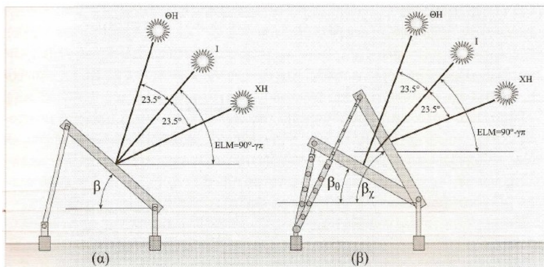
Σχήμα 3.21 (α) σταθερή στήριξη σε ετήσια βάση, με γωνία κλίσης \beta = \varphi ( 10^\circ έως 15^\circ ), (β) εποχική ρύθμιση της κλίσης του συλλέκτη δύο φορές μέσα στο έτος. ΘΗ: Θερινό Ηλιοστάσιο. ΧΗ: Χειμερινό Ηλιοστάσιο. Ι: Ισημερίες
