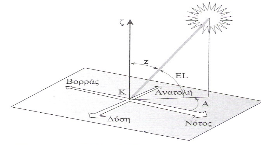
Σχήμα 3.5 Προσδιορισμός της θέσης του ήλιου στο σύστημα του τοπικού παρατηρητή
