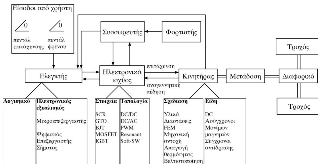
Σχήμα 5.7 Διάγραμμα συστατικών μερών κίνησης
