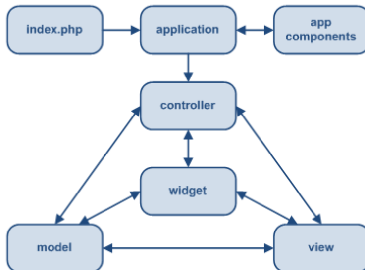
Εικόνα 13. Στατική δομή μίας εφαρμογής στο Yii
