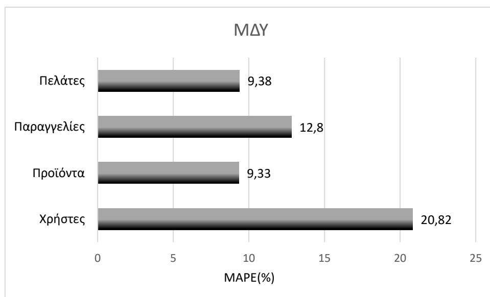
Εικόνα 5-2 Αξιολόγηση Μηχανών Διανυσμάτων Υποστήριξης
