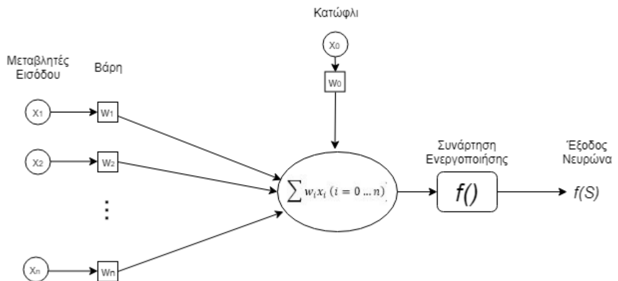
Εικόνα 2-9 Μοντέλο Τεχνητού Νευρώνα
