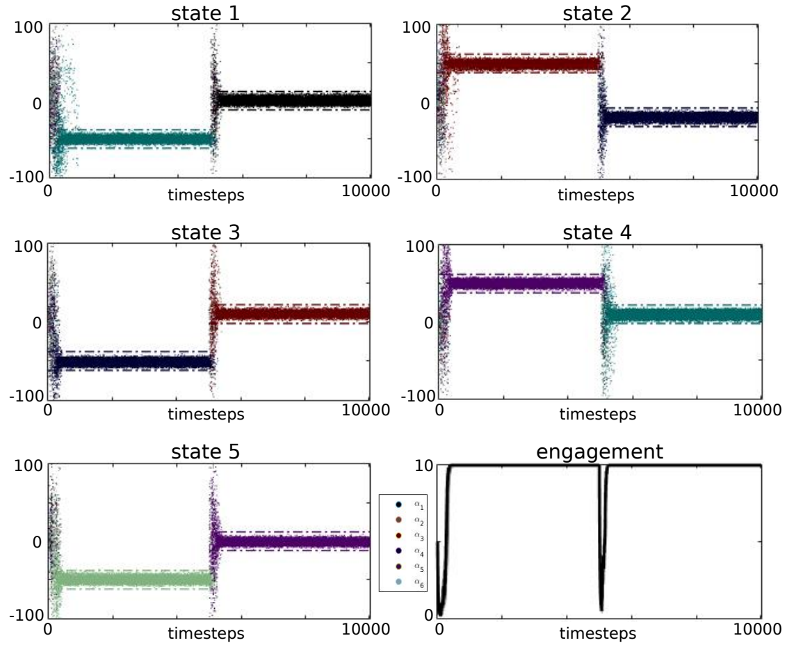
Σχήμα 6.7: Αποτελέσματα σε μη στατικό περιβάλλον με καθολικές αλλαγές διακοπτόμενου τύπου. Οι επιλεγμένες δράσεις για 50 υπερ-συνεδρίες φαίνονται ως χρωματιστές κουκκίδες σε κάθε κατάσταση και κάθε χρονική στιγμή, όπου το κάθε χρώμα αντιστοιχεί σε μία διαφορετική δράση. Η τιμή της επιλεγμένης παραμέτρου αντιστοιχεί στην κατακόρυφη θέση του κάθε σημείου. Το χρώμα των διακεκομμένων γραμμών αντιστοιχεί στη βέλτιστη διακριτή δράση, ενώ το κατακόρυφο εύρος μεταξύ των διακεκομμένων γραμμών αντιστοιχεί στο διάστημα ανοχής. Η μέση εικονική συμμετοχή/παρακολούθηση από 50 υπερ-συνεδρίες για κάθε χρονική στιγμή φαίνεται κάτω δεξιά.
