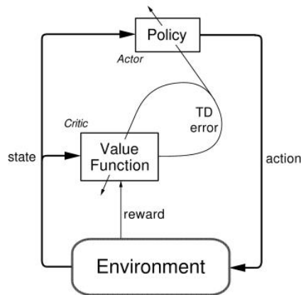
Σχήμα 5.1: Διάγραμμα ενισχυτικής μάθησης με δράστη-κριτή (Πηγή [56]).
