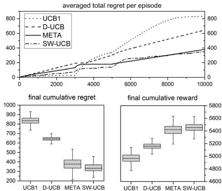
Σχήμα 4.4: Συγκριτικά αποτελέσματα αλγορίθμου MLB για το μη-στατικό διακοπτόμενο περιβάλλον του σχήματος 4.3, εκτελώντας 500 επαναλήψεις (ο MLB εδώ έχει το αχρώνυμο META). Πάνω: Μέση αθροιστική μεταμέλεια ανά χρονική στιγμή. Κάτω αριστερά: Τελική αθροιστική μεταμέλεια. Κάτω δεξιά: Μέση αθροιστική επιβράβευση.
