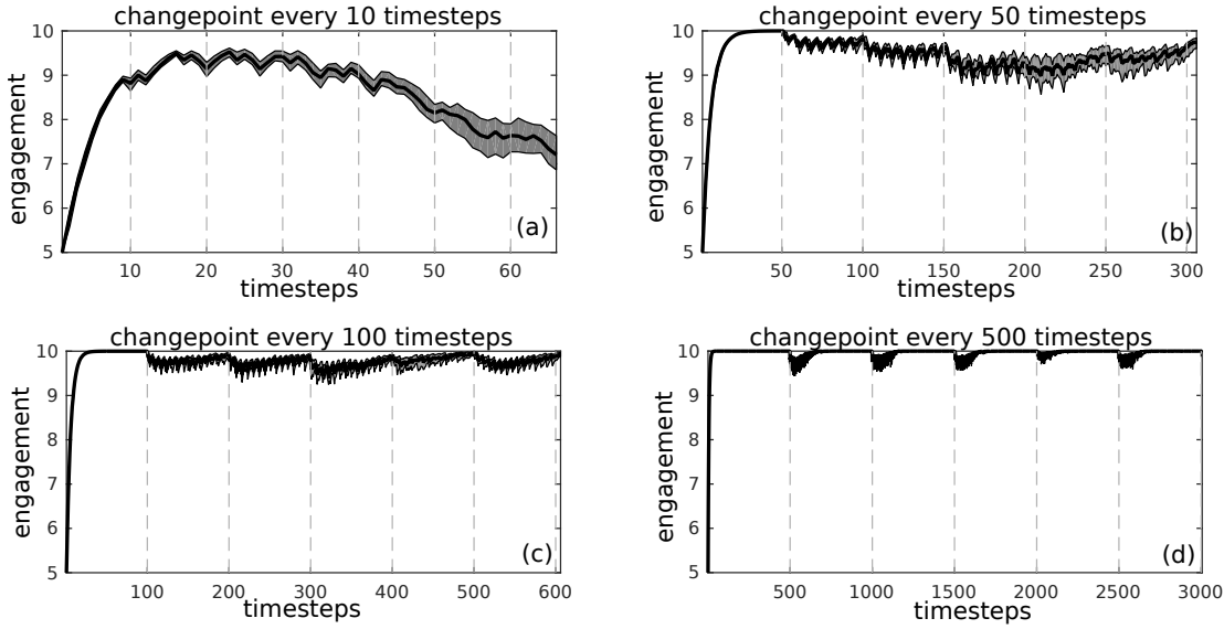
Σχήμα 6.13: Ευρωστία της αλληλεπίδρασης για διαφορετικά επίπεδα μεταβλητότητας με απεικόνιση της μέσης εικονικής συμμετοχής/παρακολούθησης μετά από 50 υπερσυνεδρίες. (a): Αλλαγή της βέλτιστης τιμής κάποιας παραμέτρου κάθε 10 κινήσεις. (b): Αλλαγή της βέλτιστης τιμής κάποιας παραμέτρου κάθε 50 κινήσεις. (c): Αλλαγή της βέλτιστης τιμής κάποιας παραμέτρου κάθε 100 κινήσεις. (d): Αλλαγή της βέλτιστης τιμής κάποιας παραμέτρου κάθε 500 κινήσεις.
