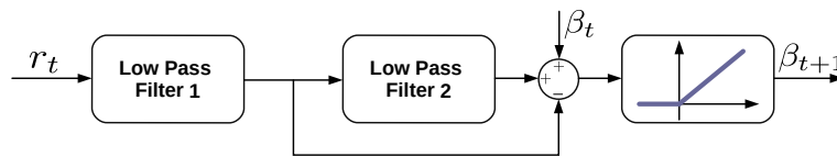
Σχήμα 4.2: Διάγραμμα μετα-μάθησης της εξερεύνησης στον αλγόριθμο MLB. Το σήμα \bar{r}_t - \bar{\bar{r}}_t καθώς και η προηγούμενη τιμή του \beta_t χρησιμοποιούνται για την ανανέωση της εξερεύνησης διαμέσου μίας τμηματικά γραμμικής μονάδας (RELU).
