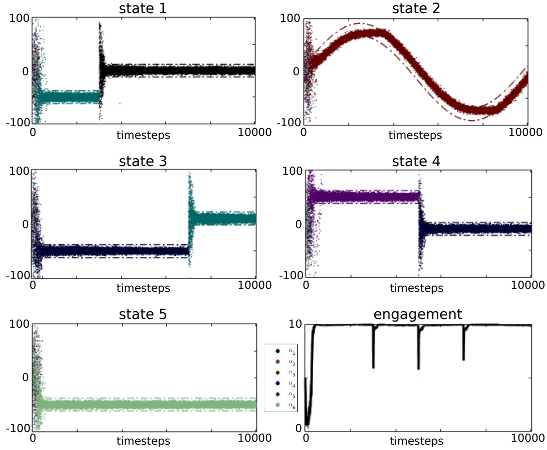
Σχήμα 6.8: Αποτελέσματα σε μη στατικό περιβάλλον με τοπικές και ομαλές αλλαγές. Σ' αυτή την περίπτωση κάθε κατάσταση μπορεί να αλλάζει σε χρονικές στιγμές ανεξάρτητα από τις υπόλοιπες, ενώ η βέλτιστη παράμετρος στην κατάσταση 2 αλλάζει με ημιτονοειδή τρόπο στην πάροδο του χρόνου. Η περιγραφή της διάταξης είναι παρόμοια με αυτή του σχήματος 6.7.
