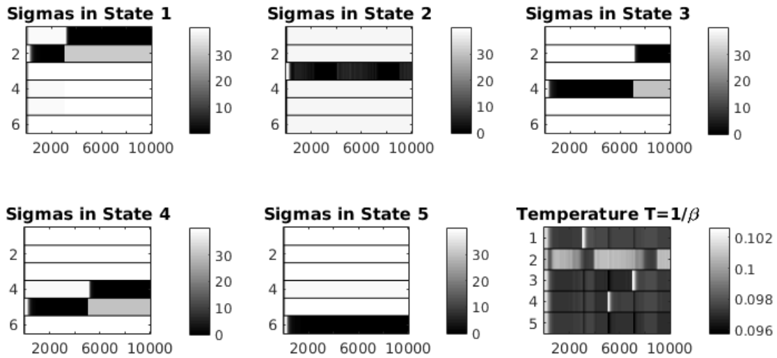
Σχήμα 6.9: Αβεβαιότητα σε μη στατικά περιβάλλοντα με τοπικές αλλαγές. Κάτω δεξιά: Απεικονίζεται η μέση θερμοκρασία T(s) = 1/\beta(s) για κάθε μία από τις 5 καταστάσεις (γραμμές), σε κάθε χρονική στιγμή. Υπόλοιπες απεικονίσεις: Εμφάνιση της μέσης αβεβαιότητας \sigma(s, a) για κάθε δράση (γραμμές) σε κάθε κατάσταση, για κάθε χρονική στιγμή.
