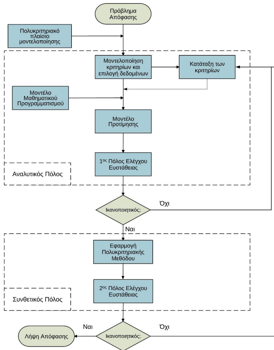
Σχήμα 7.1: Διάγραμμα ροής μεθοδολογίας ελέγχου ευστάθειας για τη μέθοδο Simos
