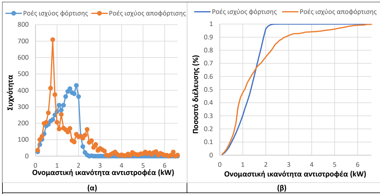
Σχήμα 5.4: Συχνότητα των ετήσιων ροών ισχύος στο διάστημα 0-6,6 kW (α) και ποσοστό διέλευσης ετήσιων ροών ισχύος (β) ανάλογα με την ονομαστική ικανότητα του αντιστροφέα για Φ/Β παραγωγή 1 MWh/MWh φορτίου και χρήσιμη χωρητικότητα μπαταρίας 1 kWh/MWh φορτίου.
