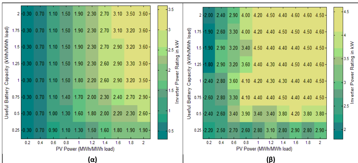
Σχήμα 5.5: Βέλτιστη ονομαστική ισχύς του αντιστροφέα σε kW που ικανοποιεί το 95% των ροών ισχύος φόρτισης (α) και το 95% των ροών ισχύος αποφόρτισης.
