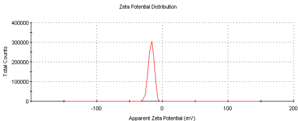
Σχήμα 7.54: Κατανομή δυναμικού Zeta για το δείγμα M8
