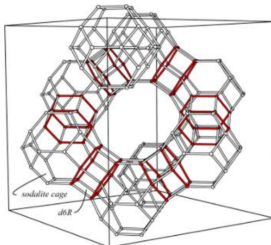
Σχήμα 5.16: Κλωβοί σοδαλίτη στον τύπο πλαισίου FAU
