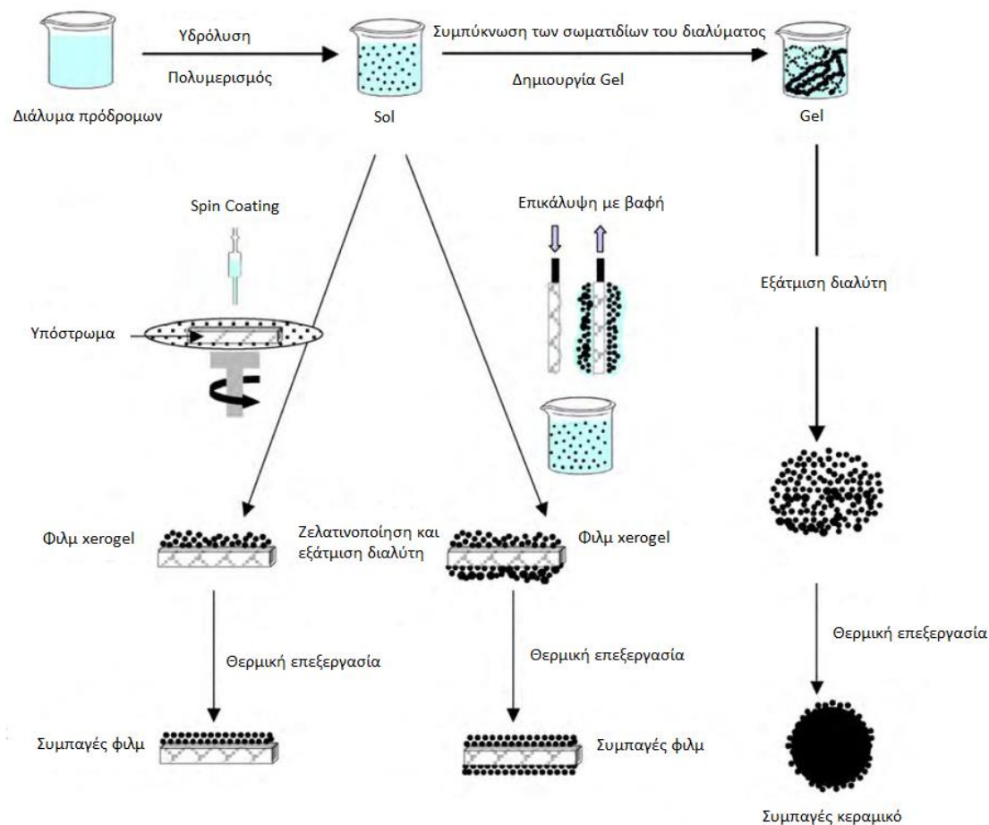
Σχήμα 4.2: Σύνθεση νανοσωματιδίων με τη μέθοδο sol-gel: υμένια από κολλοειδές sol και σκόνη από κολλοειδές sol μετασχηματισμένο σε gel [185]
