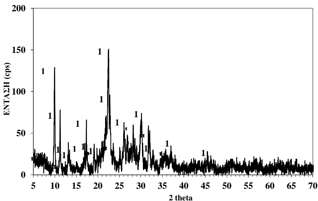
Σχήμα 7.19: Φάσμα περίθλασης ακτίνων X για τον Κλινοπτιλολίτη-Na
