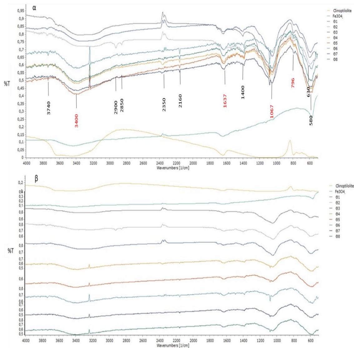
Σχήμα 7.24: Φάσματα απορρόφησης υπέρυθρων για τα δείγματα της σειράς Θ, καθαρό μαγνητίτη και κλινοπτιλολίτη-Na (με κόκκινο σημειώνονται οι κυματάρηθμοι που αφορούν αποκλειστικά στον κλινοπτιλολίτη) α) όπως εμφανίζονται στο FTIR και β) στοιχισμένα με βάση τη διαπερατότητα τους.
