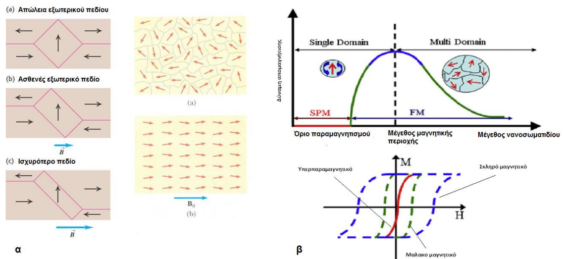
Σχήμα 3.7: α) Προσανατολισμός μαγνητικών ροπών και αυξομειώσεις μαγνητικών περιοχών με την επιβολή εξωτερικού μαγνητικού πεδίου, β) Διάγραμμα απομαγνήτισης – μεγέθους μαγνητικών σωματιδίων και M-H βρόχος για μαλακά φερρομαγνητικά, σκληρά φερρομαγνητικά και υπερπαραμαγνητικά υλικά
