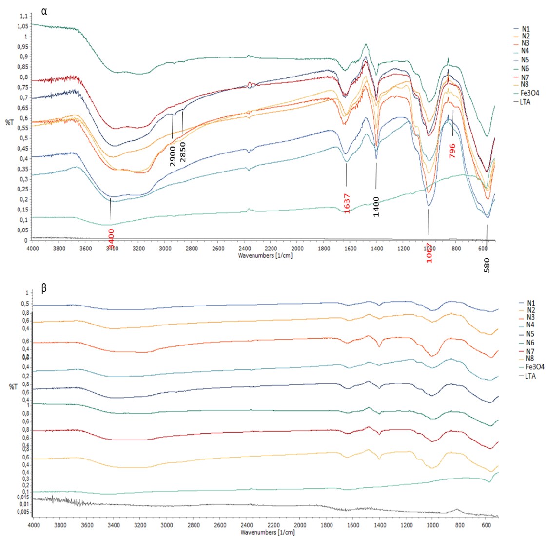
Σχήμα 7.50: Φάσματα απορρόφησης υπέρυθρων για τα δείγματα της σειράς N, καθαρό μαγνητίτη και ζεόλιθο A (με κόκκινο σημειώνονται οι κυματάρηθμοι που αφορούν αποκλειστικά στον LTA) α) όπως εμφανίζονται στο FTIR και β) στοιχισμένα με βάση τη διαπερατότητα τους.
