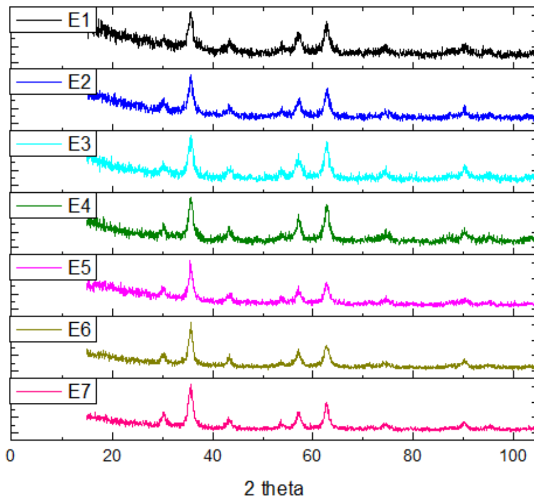
Σχήμα 7.9: Φάσματα περίθλασης ακτινών X για τη σειρά δειγμάτων E
