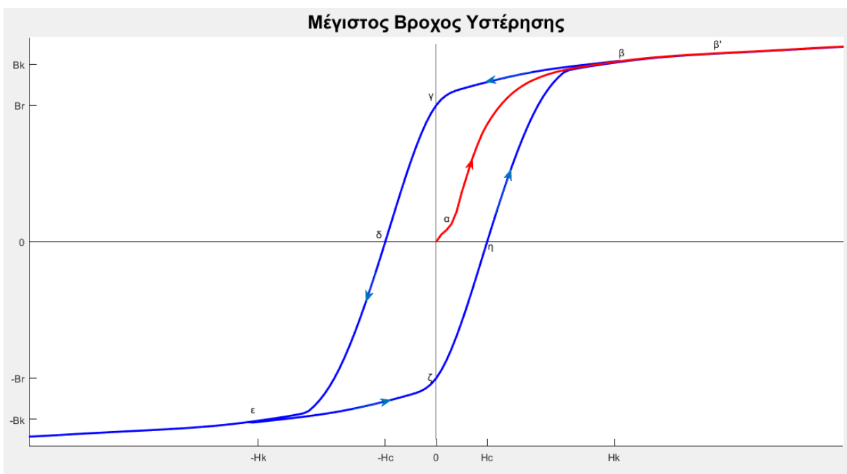
Διάγραμμα 2. 2 Μέγιστος βρόχος υστέρησης σιδηρομαγνητικού υλικού
