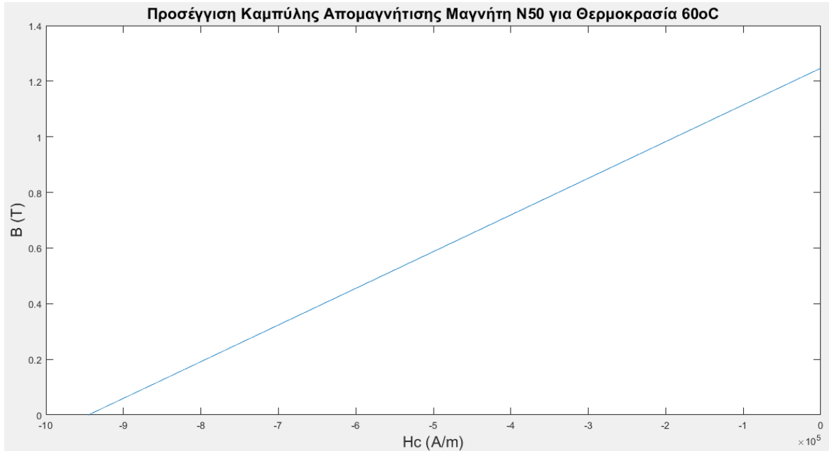
Διάγραμμα 4. 2 Προσέγγιση Καμπύλης Απομαγνήτισης Μαγνήτη N50 στους 60°C
