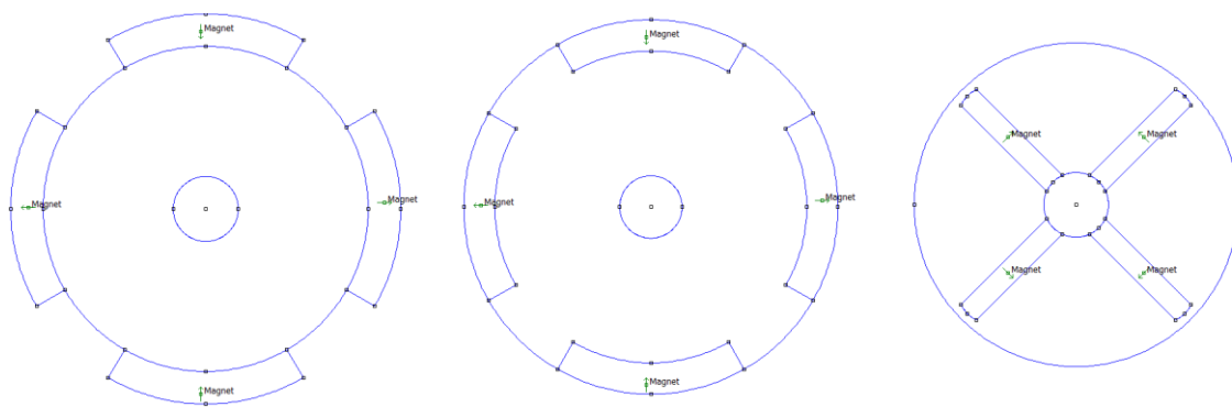
Σχήμα 2. 5 Αναπαραστάσεις τοπολογιών δρομέα ανάλογα με τη θέση του μαγνήτη
