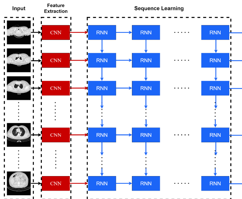
Σχήμα 4.1 Αρχιτεκτονική CNN-RNN
