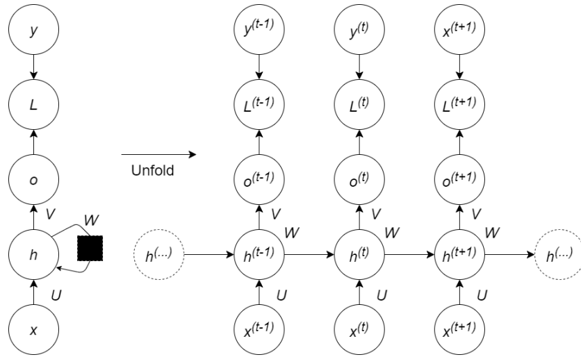
Σχήμα 2.12 Ακολουθιακό Δίκτυο
