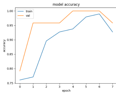
Σχήμα 5.3 Καμπύλη Ακρίβειας
