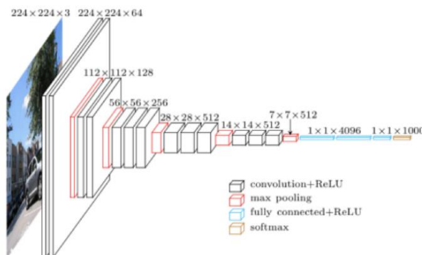
Σχήμα 2.10 Δομή VGG-16
