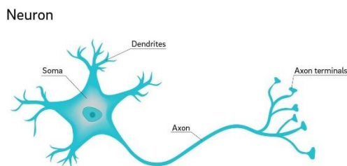
Σχήμα 2.3 Βιολογικός Νευρώνας
