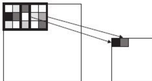
Εικόνα 3: 3 \times 3 max pooling με βήμα s = 2 (Πηγή: [4])
