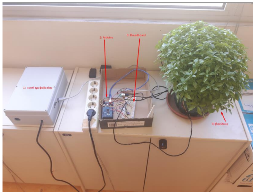
Εικόνα 19: IoT οικοσύστημα
