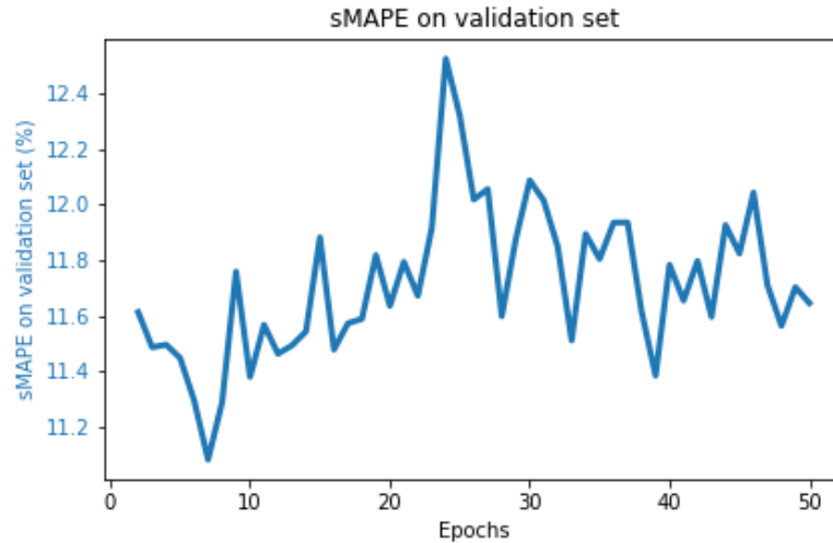
Σχήμα 6.2: Δείκτης sMAPE ανά Εποχή στο Σύνολο Επικύρωσης. Η εποχή 7 έχει το μικρότερο sMAPE στο σύνολο επικύρωσης και συνεπώς η ίδια εποχή επιλέγεται ως καλύτερη και για το σύνολο αξιολόγησης
