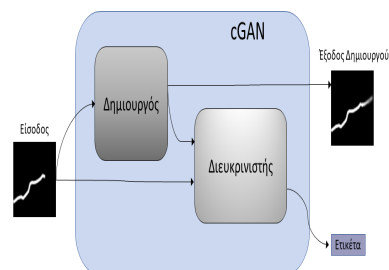
Υπό Συνθήκη Γεννητικό Ανταγωνιστικό Δίκτυο (Conditional Generative Adversarial Network - cGAN)
