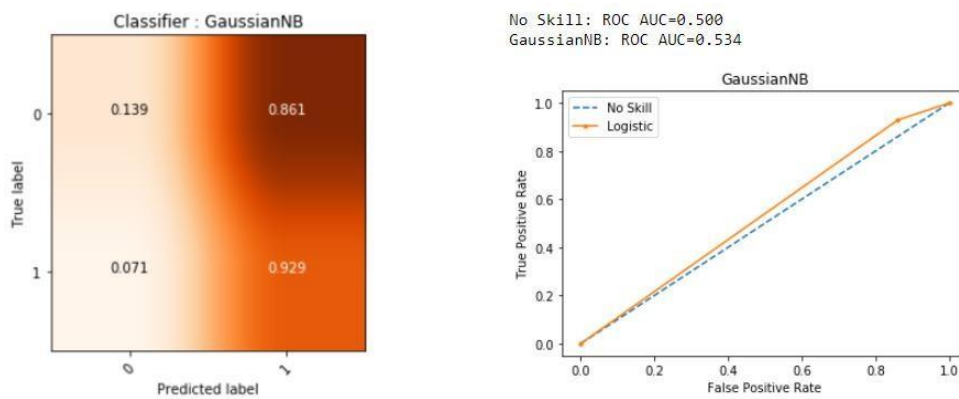
Εικόνα 7. Feature Extraction / GaussianNB
