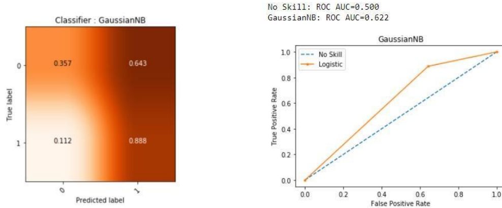
Εικόνα 1. BagOfWords / GaussianNB
