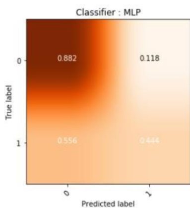
Εικόνα 10. FeatureExtraction / MLP
