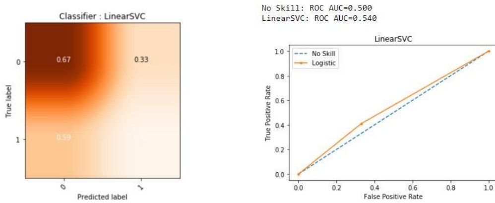
Εικόνα 5. Συγκρότητα Όρων / Linear SVC
