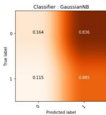
Εικόνα 4. Συχνότητα Όρων / GaussianNB
