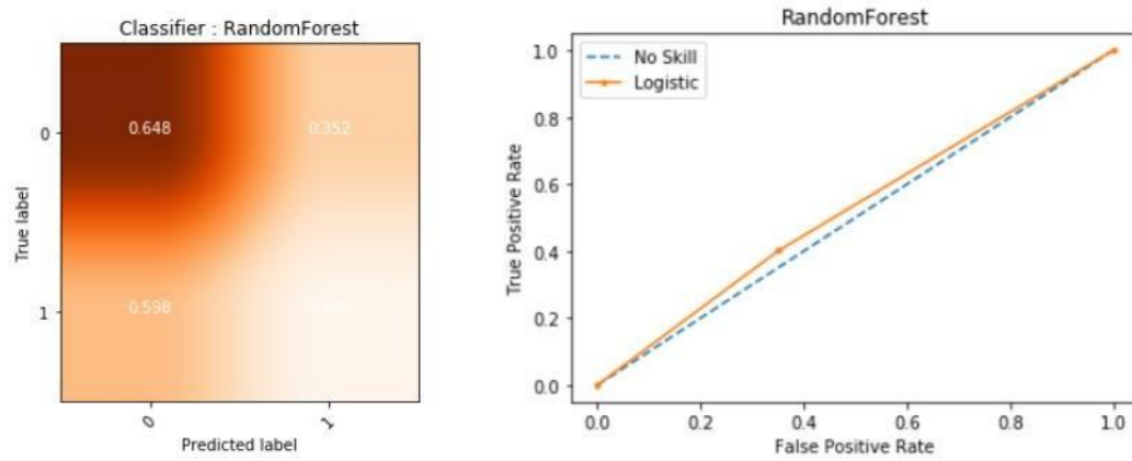
Εικόνα 6. Συγκρότητα Όρων / Random Forest
