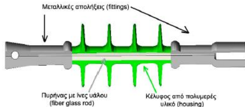
Εικόνα 1.10. Τομή σε μοντέλο συνθετικού μονωτήρα όπου διακρίνονται το πολυμερικό περίβλημα, ο πυρήνας και οι μεταλλικοί ακροδέκτες [29]
