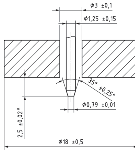
Εικόνα 2.17-Δεισδυτής για σκληρόμετρα τύπου A (διαστάσεις σε mm) [46]
