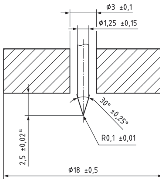
Εικόνα 2.18-Δεισδυτής για σκληρόμετρα τύπου D (διαστάσεις σε mm) [46]
