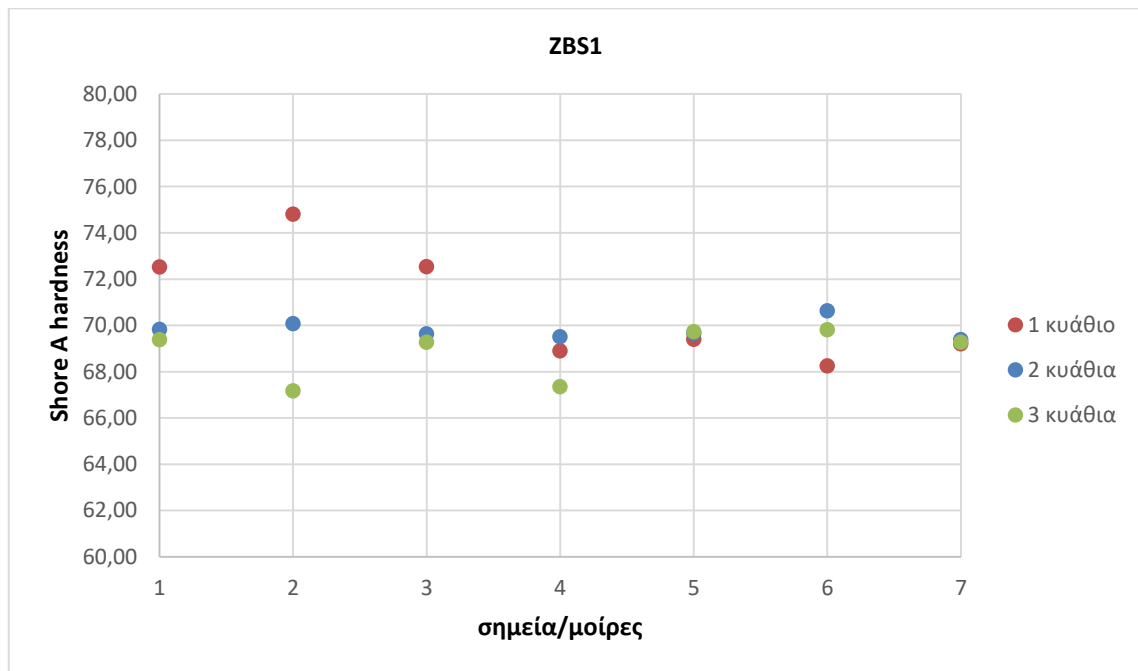
Σχήμα 3.1 Μέσος Όρος σκληρότητας μονωτήρα ZBS1 ανά σημείο/μείρες σε διαφορετικά επίπεδα κιαθίων
