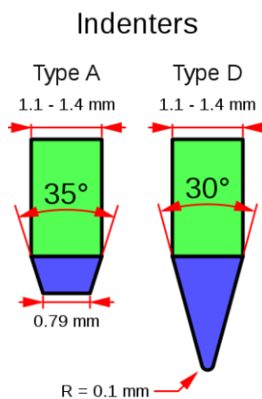
Εικόνα 2.14 Διαστάσεις διεισδυτών τύπου A και D [44]
