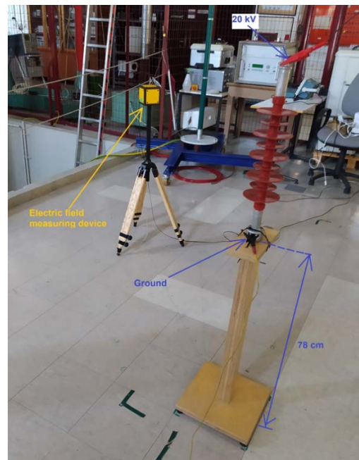
Σχήμα 4-1 : Διάταξη Εργαστηρίου
