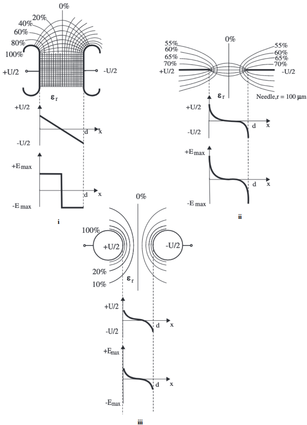
Σχήμα 2-4: Διαμορφώσεις Ηλεκτρικού πεδίου- (i) Ομοιόμορφο πεδίο ανάμεσα σε δύο παράλληλες πλάκες, (ii) Ασθενώς ανομοιόμορφο πεδίο ανάμεσα σε δύο σφαίρες, (iii) Ανομοιόμορφο πεδίο ανάμεσα σε δύο ηλεκτρόδια [32]
