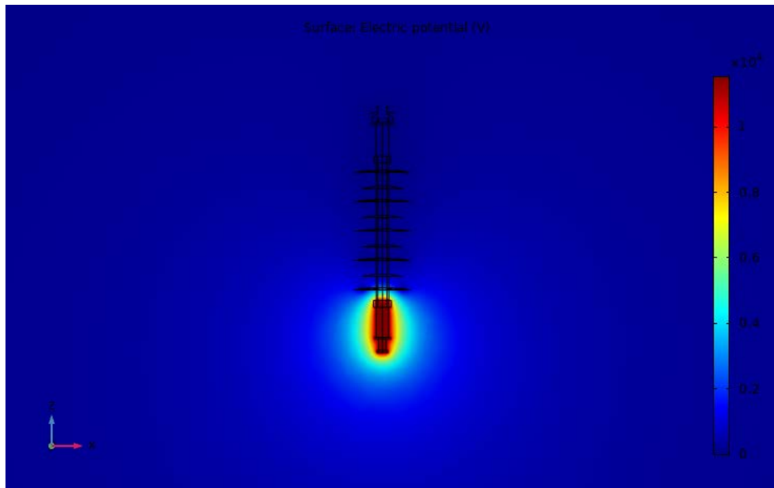
Σχήμα 4-38 : Κατανομή Δυναμικού Μονωτήρα Ανάρτησης Κλάσης 2
