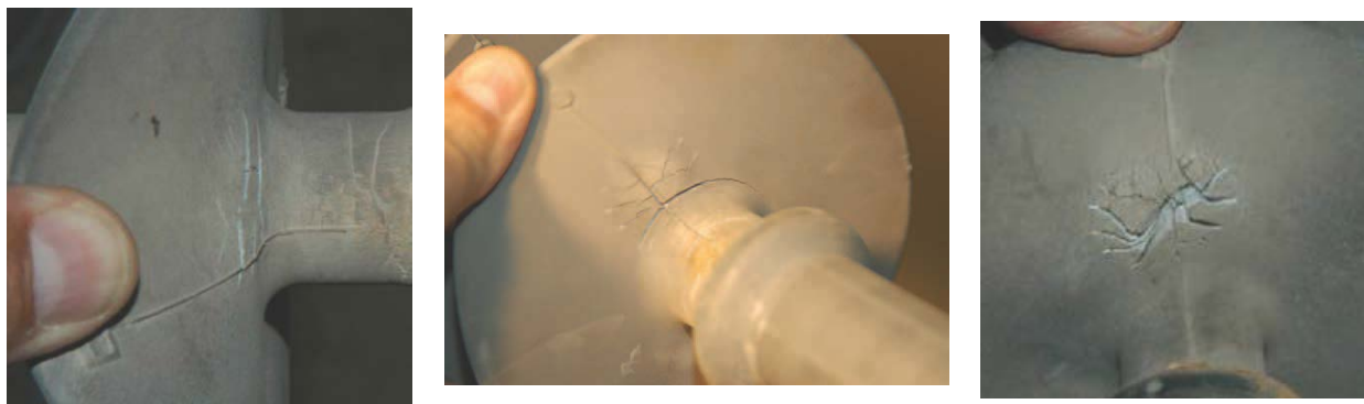
Σχήμα 1-20 : Σχισμένος Μονωτήρας [26]
