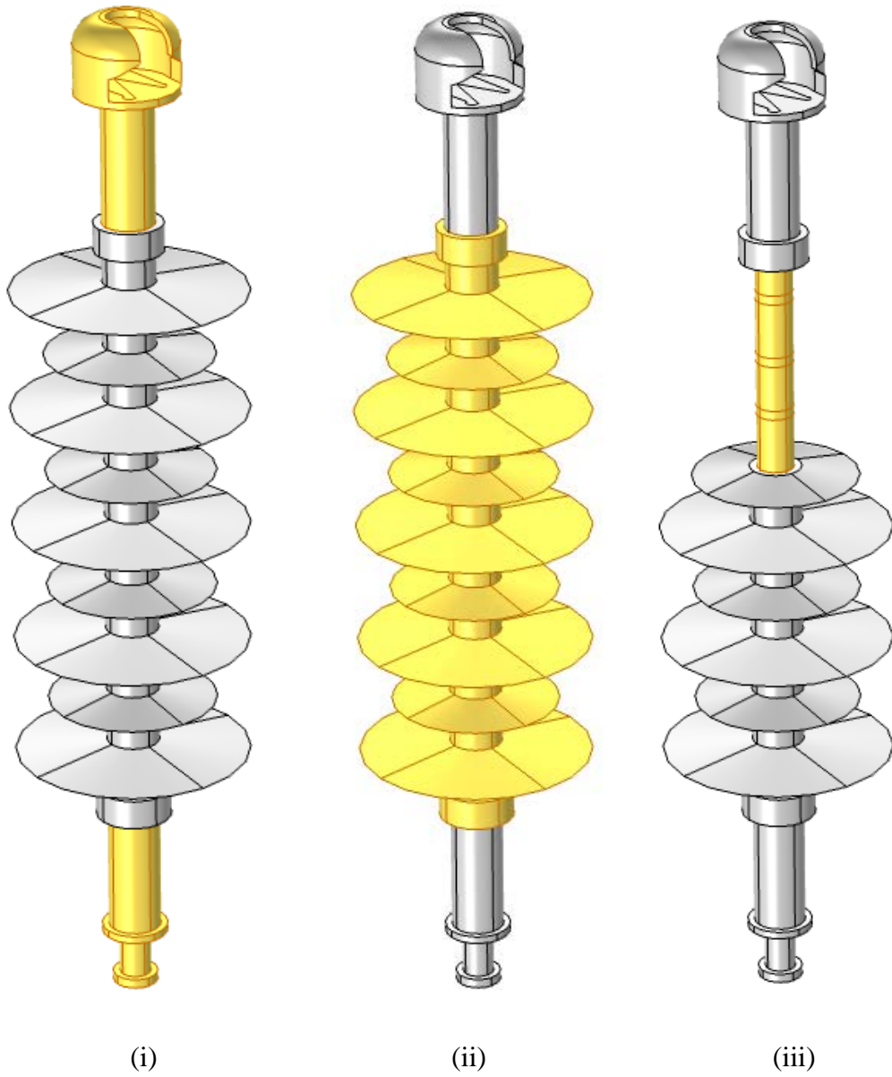
Σχήμα 3-11 : Τοποθέτηση υλικών (i) στα άκρα , (ii) στα κιάθια και (iii) στον εσωτερικό κύλινδρο μονωτήρα ανάρτησης
