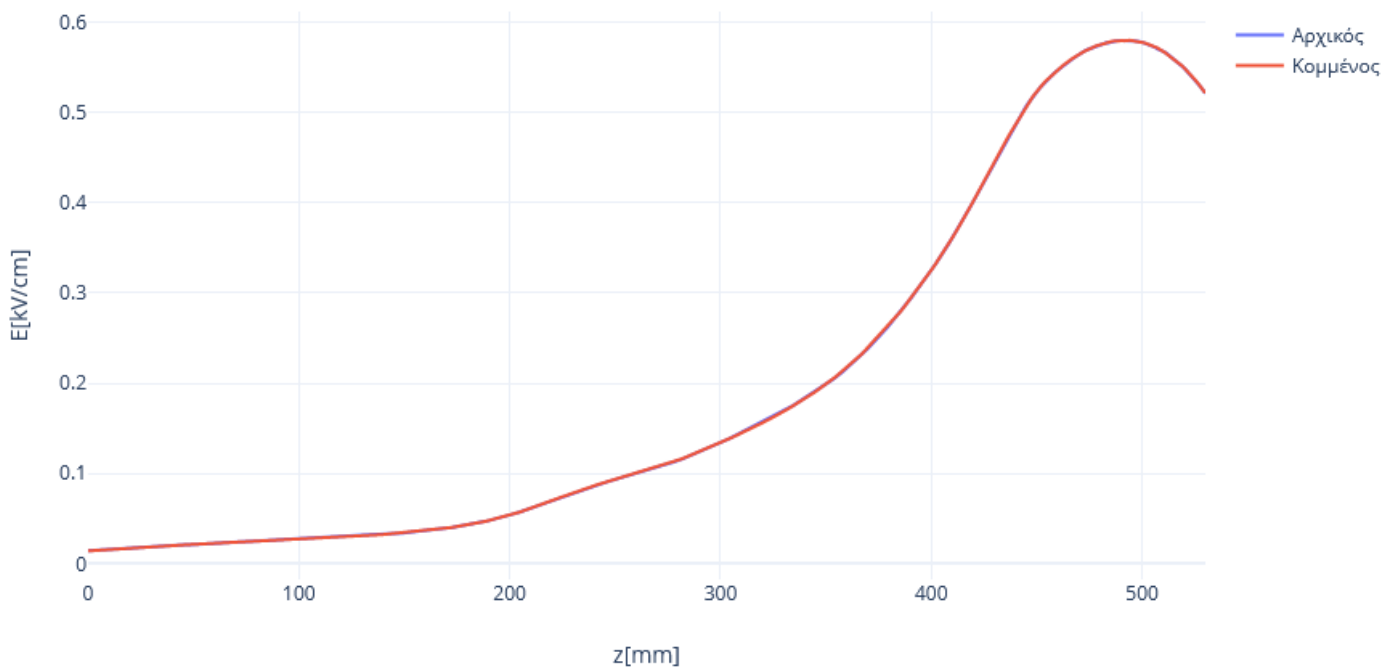
Σχήμα 5-12 : Σύγκριση Έντασης Ηλεκτρικού Πεδίου Μονωτήρα Γραμμής με και χωρίς κομμένα κιάτια για x=80, y=0
