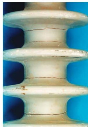
Σχήμα 1-12: Περιφερειακές Ρωγμές Εποξικού Περιβλήματος [20]
