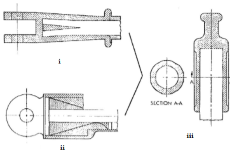
Σχήμα 1-16 : Χρήση σφήνας (i), συγκόλλησης (ii) και σύνδεσης με συμπίεση (swaged) (iii) για την προσάρτηση του μεταλλικού ακροδέκτη στον πυρήνα του μονωτήρα [20]
