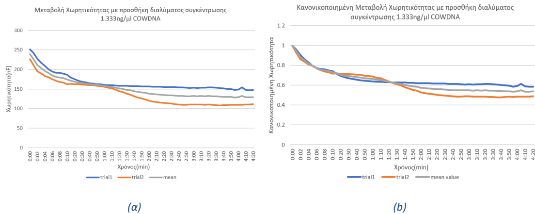
Σχήμα 67 (α) Μεταβολή Χωρητικότητας, (β) Κανονικοποιημένη Μεταβολή Χωρητικότητας πυκνωτών με ακινητοποιημένο COWFORW-COWREV εκκινήτη με προσθήκη διαλύματος συγκέντρωσης 1.333ng/μl COWDNA μετά από αποθήκευση 5 ημερών
