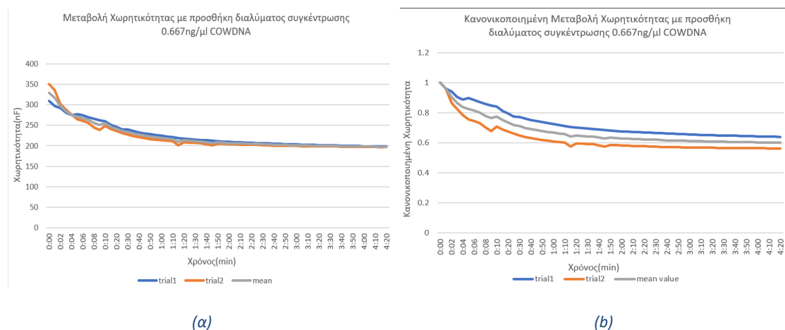
Σχήμα 68 (α) Μεταβολή Χωρητικότητας, (β) Κανονικοποιημένη Μεταβολή Χωρητικότητας πυκνωτών με ακινητοποιημένο COWREV εκκινήτη με προσθήκη διαλύματος συγκέντρωσης 0.667ng/μl COWDNA μετά από αποθήκευση 5 ημερών
