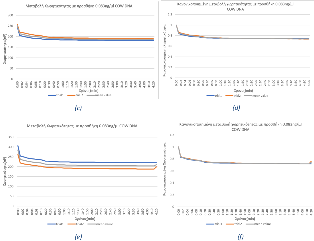
Σχήμα 55 ((a),(c),(e)) Μεταβολή Χωρητικότητας, ((b),(d),(f)) Κανονικοποιημένη Μεταβολή Χωρητικότητας πυκνωτών με ακινητοποιημένο ((a),(b)) COWFORW, ((c),(d)) COWREV, ((e),(f)) COWFORW-COWREV εκκινήτη με προσθήκη διαλύματος με συγκέντρωση 0.083ng/μl COW DNA
