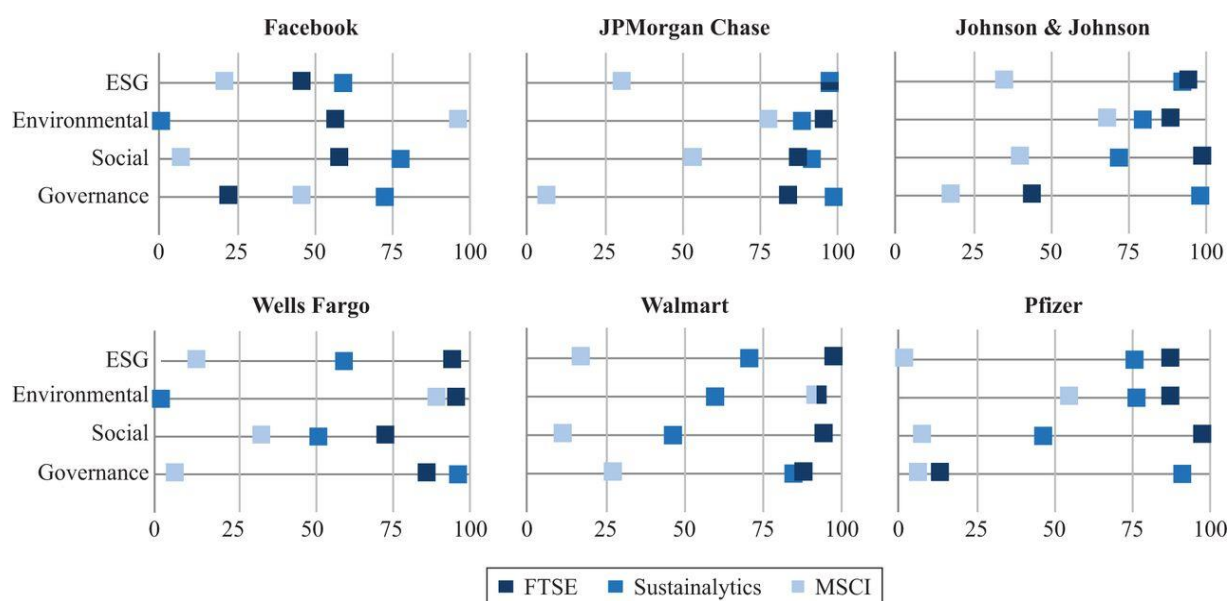
Διάγραμμα 3:Αποκλίσεις οργανισμών αξιολόγησης ESG μεταξύ μεγάλων αμερικάνικων εταιρειών. (D.3) 54
