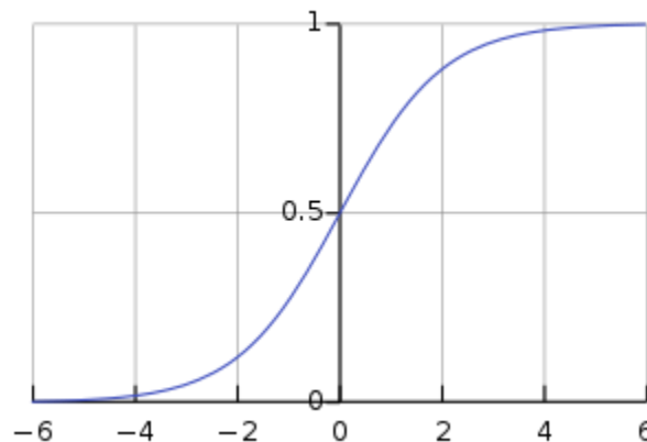
Σχήμα 6: Σιγμοειδής συνάρτηση [3]
