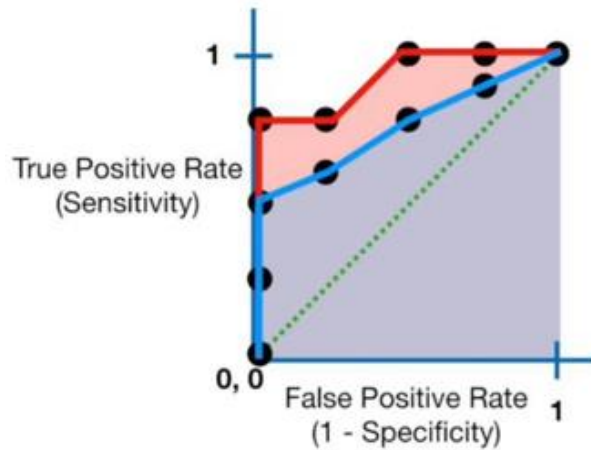
Σχήμα 2: Δύο διαφορετικά μοντέλα με τις αντίστοιχες ROC curves & AUC που παράγουν
