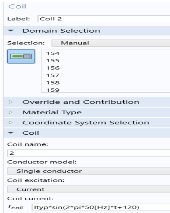
Εικόνα 7.27: Coil 2 (Φάση 2) COMSOL.
