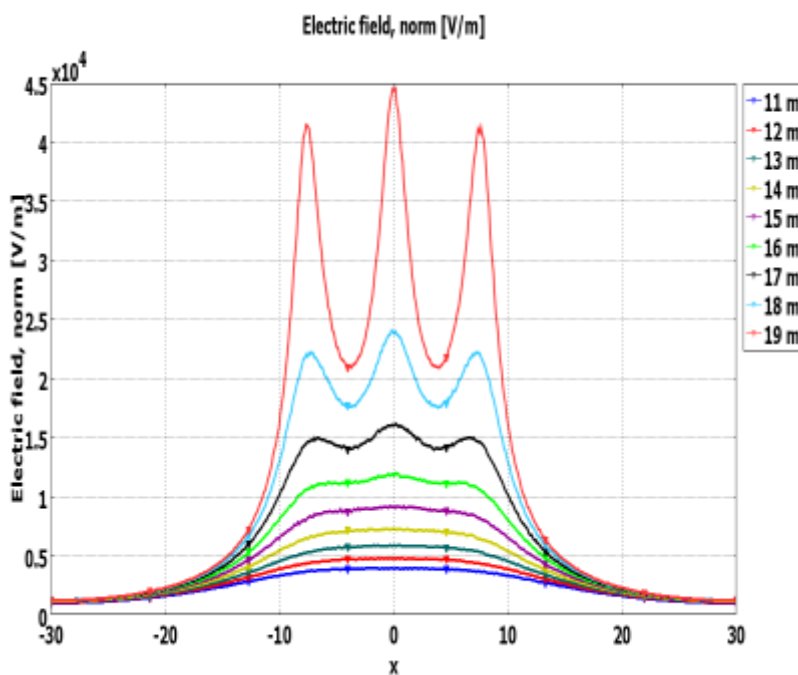
Σχήμα 8.22: Πλευρικά προφίλ ηλεκτρικού πεδίου για τα επίπεδα από 11m έως 19m.
