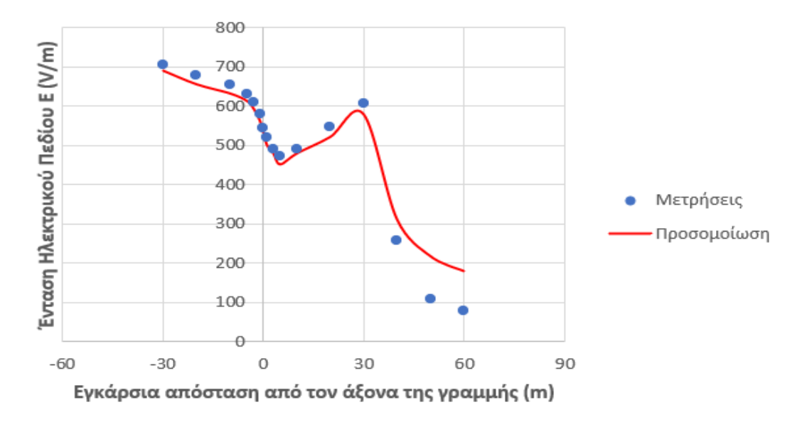
Σχήμα 8.33: Αποτελέσματα προσομοίωσης και μετρούμενες τιμές της έντασης του ηλεκτρικού πεδίου σε άξονα εγκάρσιο στο τμήμα της γραμμής ΑΑ228/60 και ΑΑ228/61.
