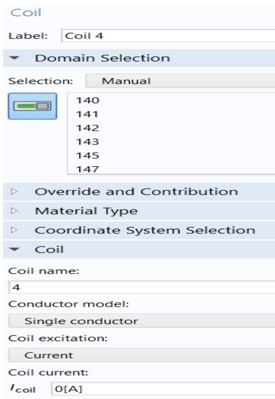
Εικόνα 7.29: Coil 4 (Γείωση) COMSOL.
