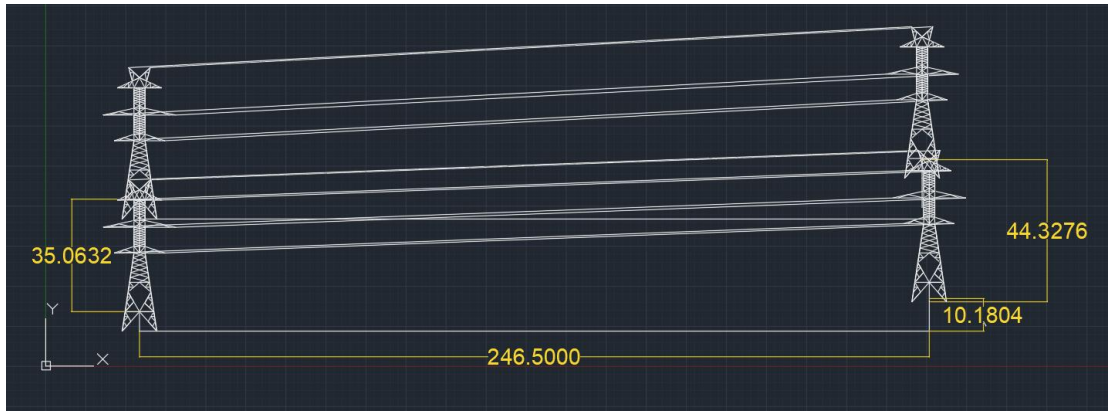
Εικόνα 6.3: Απεικόνιση της γραμμής μεταφοράς (Πάνω αριστερά είναι ο Πυλώνας ΚΑΣ54 ακριβώς από κάτω είναι ο Πυλώνας ΑΡΚ59 και στη δεξιά μεριά πάνω είναι ο Πυλώνας ΚΑΣ55 και ακριβώς από κάτω ο Πυλώνας ΑΡΚ60).
