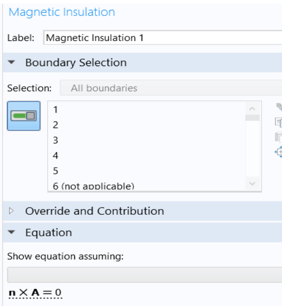
Εικόνα 7.23: Magnetic Insulation 1 COMSOL.
