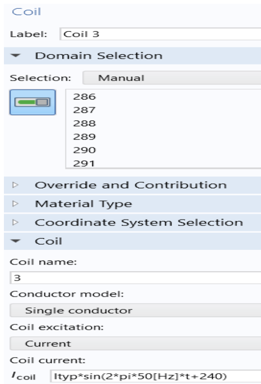
Εικόνα 7.28: Coil 3 (Φάση 3) COMSOL.
