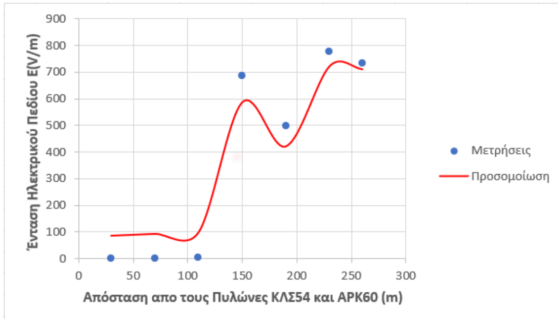
Σχήμα 8.2: Αποτελέσματα προσομοίωσης και μετρούμενες τιμές της έντασης του ηλεκτρικού πεδίου σε άξονα κατά μήκος του τμήματος της γραμμής ΚΛΣ 55-ΚΛΣ54 και ΑΡΚ 59-ΑΡΚ 60.
