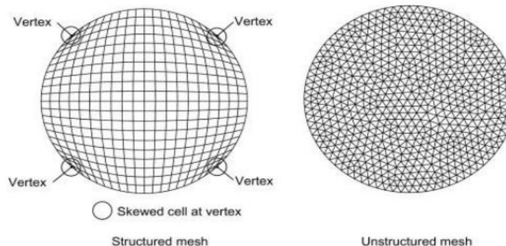
Εικόνα 7.35: Δομημένο και Αδόμητο Πλέγμα από Manual COMSOL Multiphysics [1].
