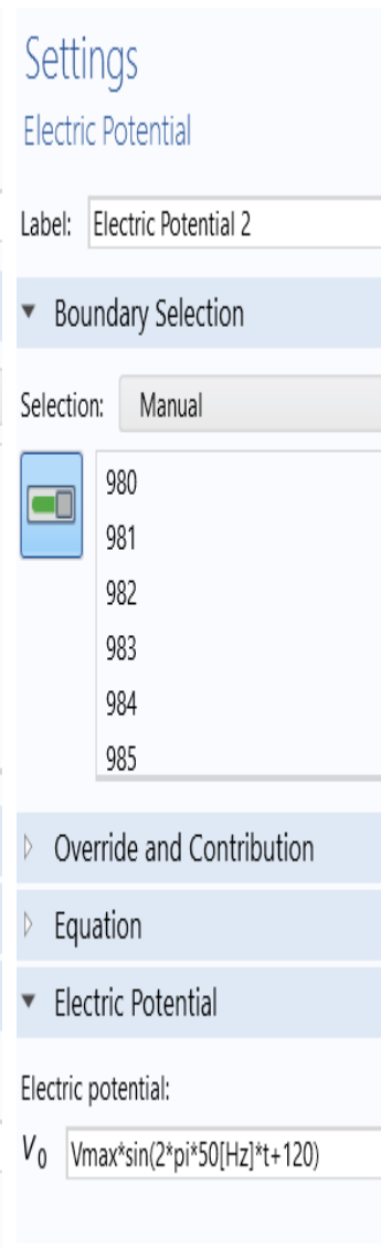
Εικόνα 7.20: Electric Potential 1 (Φάση 2) COMSOL.
