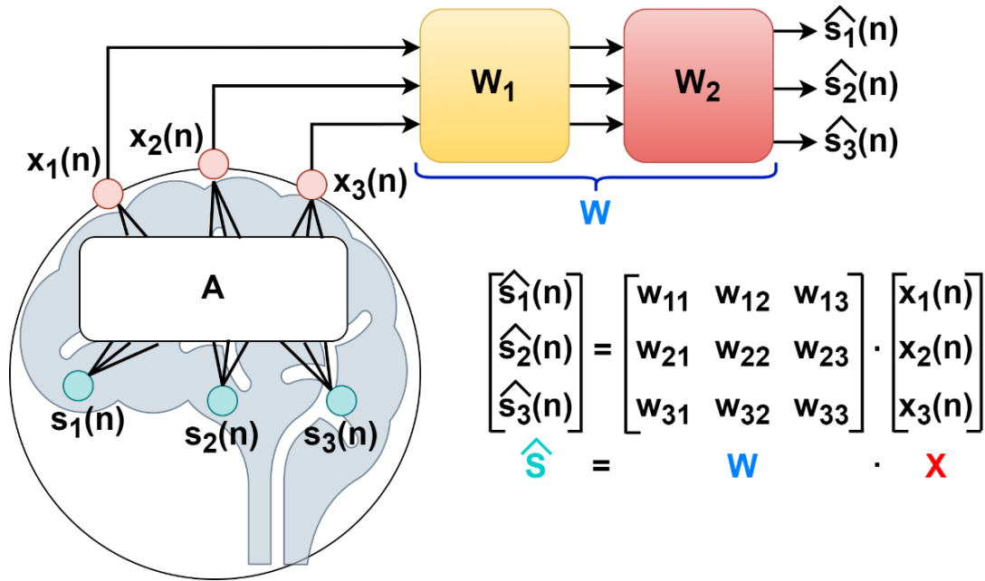
Σχήμα 2. Γραμμική μείξη πηγών κατά τον τυφλό διαχωρισμό πηγών στο EEG.
