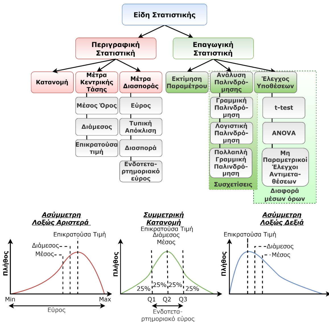
Σχήμα 1. Είδη Στατιστική, θεμελιώδεις στατιστικοί δείκτες και μέθοδοι ανά είδος και γραφική αναπαράσταση των στατιστικών μέτρων σε τρεις γενικές κατηγορίες κατανομών.
