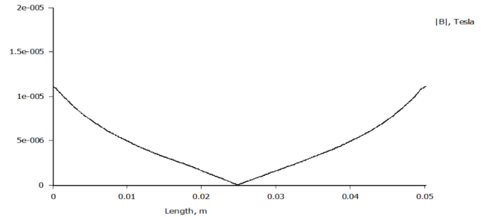
(β) 50 Hz
