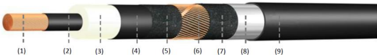
Εικόνα 3. Σχηματική αναπαράσταση τυπικού καλωδίου ισχύος: (1) εσωτερικός αγωγός, (2) εσωτερικό ημιαγώγιμο, (3) μόνωση, (4) εξωτερικό ημιαγώγιμο, (5) ημιαγώγιμη υδροφοβική ταινία, (6) metallic screen-shield, (7) ημιαγώγιμη υδροφοβική ταινία, (8) αλουμινένια ταινία, (9) εξωτερικός πολυμερικός μανδύας
