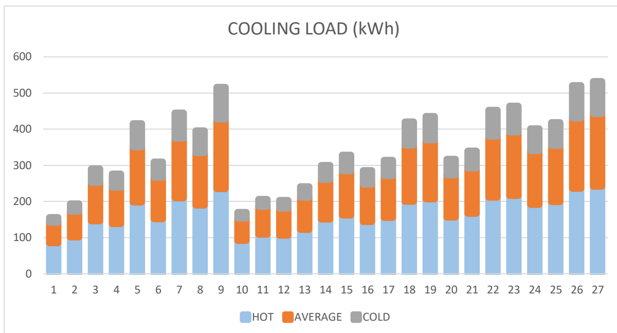
Εικόνα 4.29: Γραφική φορτίου ψύξης
