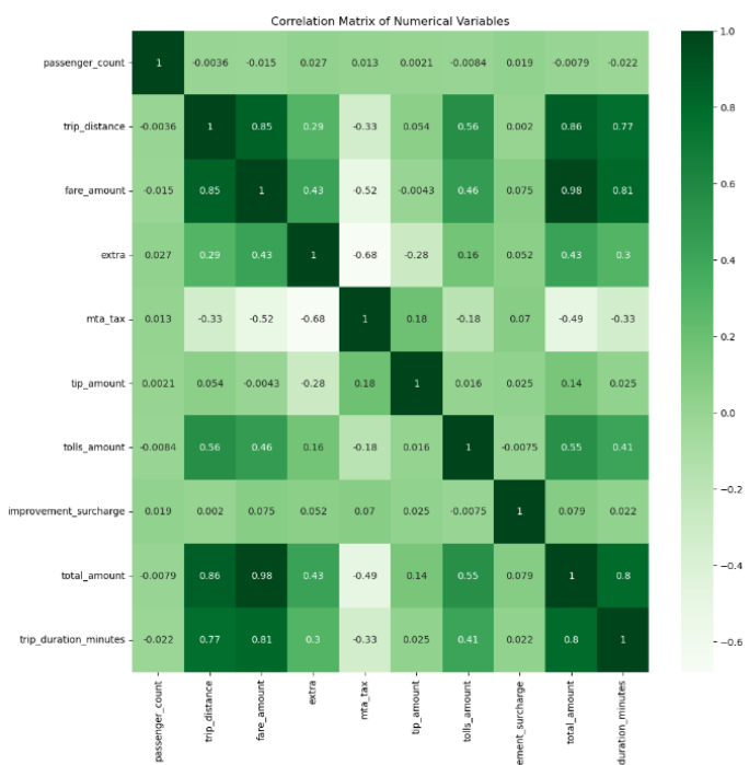
Εικόνα 38. Πίνακας συσχέτισης αριθμητικών χαρακτηριστικών για τα ταξί της Νέας Υόρκης
