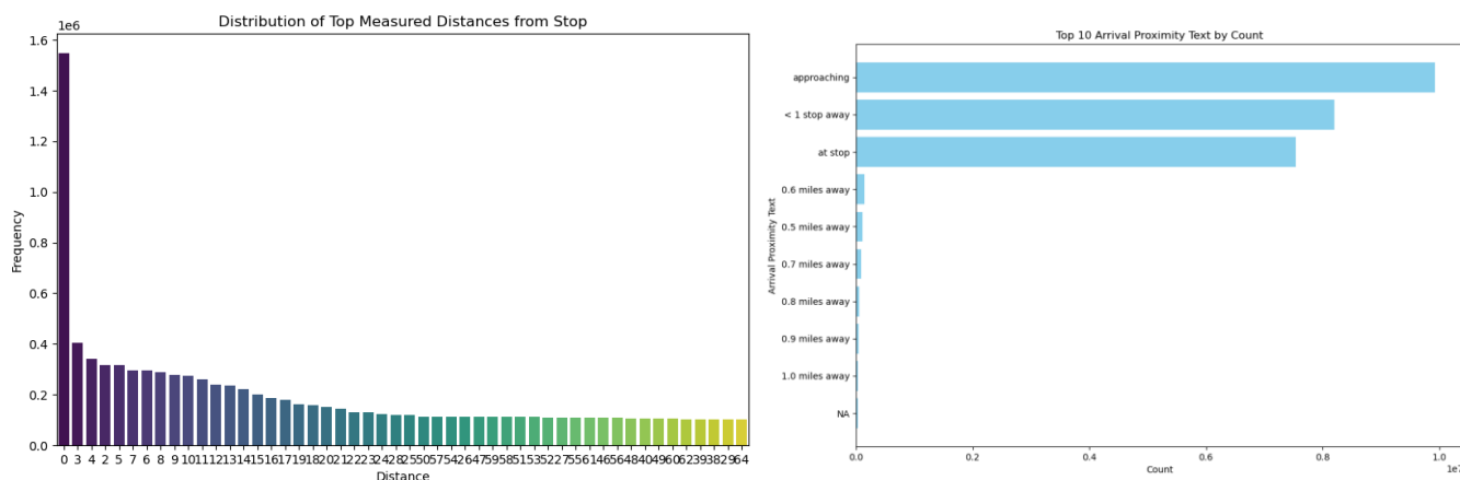
Εικόνα 30. Διάγραμμα συχνοτήτων των χαρακτηριστικών που μετράνε την απόσταση από την στάση. Αριστερά σχετική απόσταση από στάση, Δεξιά κατηγορική σχετική απόσταση από στάση.
