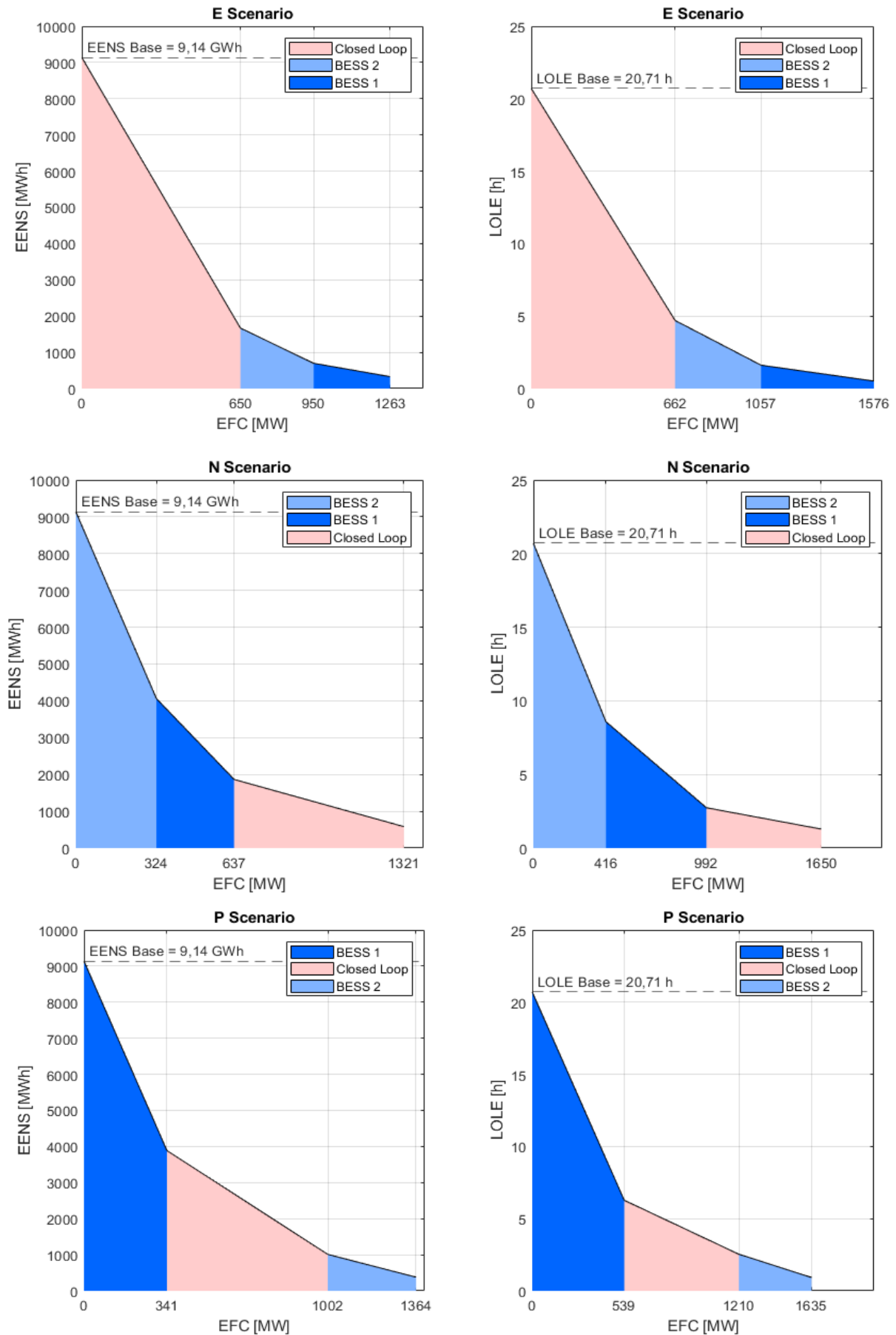
Σχήμα 37: Σταδιακός Υπολογισμός Capacity Value της κάθε μονάδας αποθήκευσης συναρτήσει του EENS και του LOLE για τα σενάρια σειριακής λειτουργίας E, N, P.
