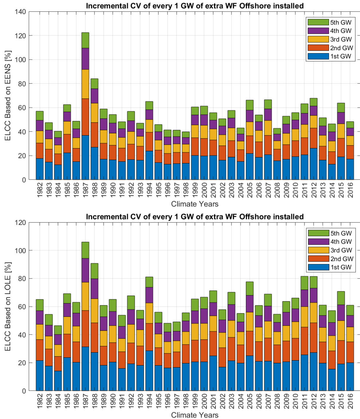
Σχήμα 43: Αποτελέσματα ELCC για σενάρια επιπλέον διείσδυσης υπεράκτιων ΑΠ με βάση το (α) EENS και (β) το LOLE
