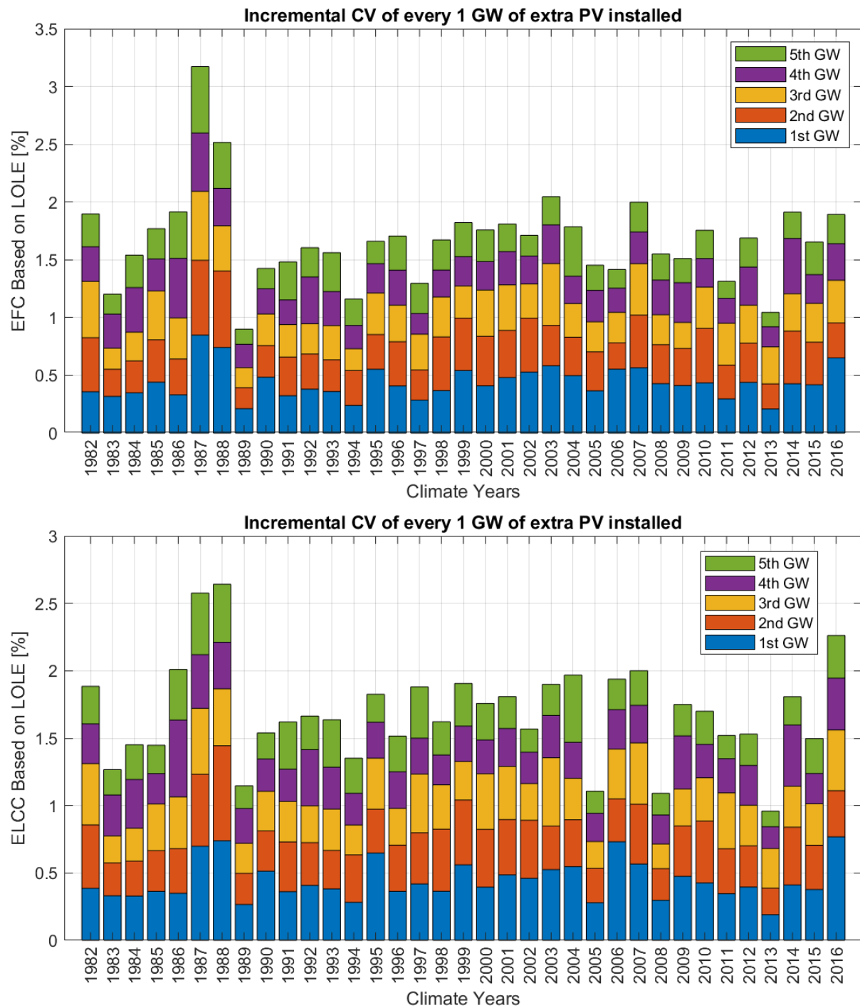
Σχήμα 39: Αποτελέσματα ELCC για σενάρια επιπλέον διείσδυσης ΦΒ με βάση το (α) EENS και (β) το LOLE
