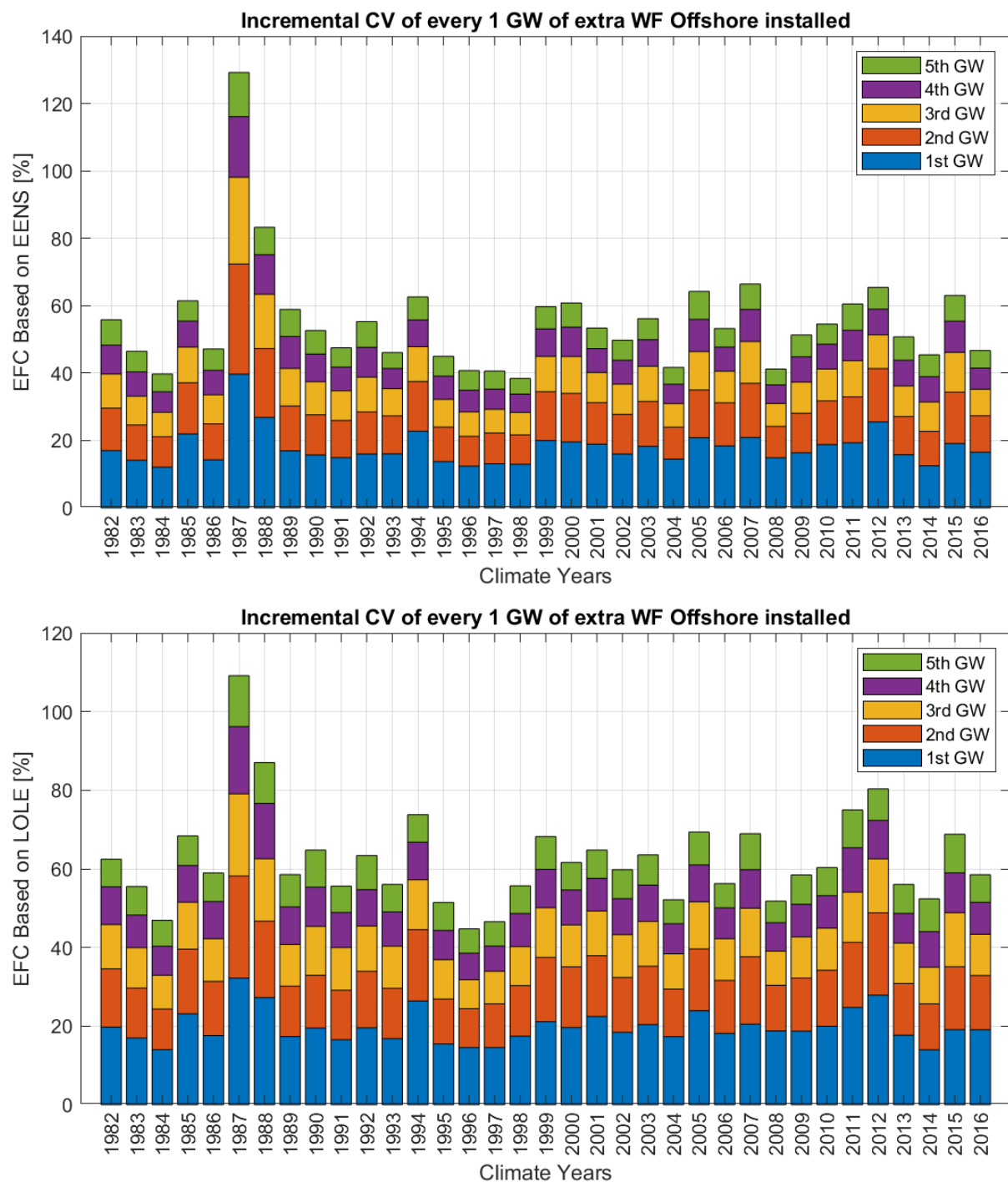
Σχήμα 42: Αποτελέσματα EFC για σενάρια επιπλέον διεύθυνσης υπεράκτιων ΑΠ με βάση το (α) EENS και (β) το LOLE
