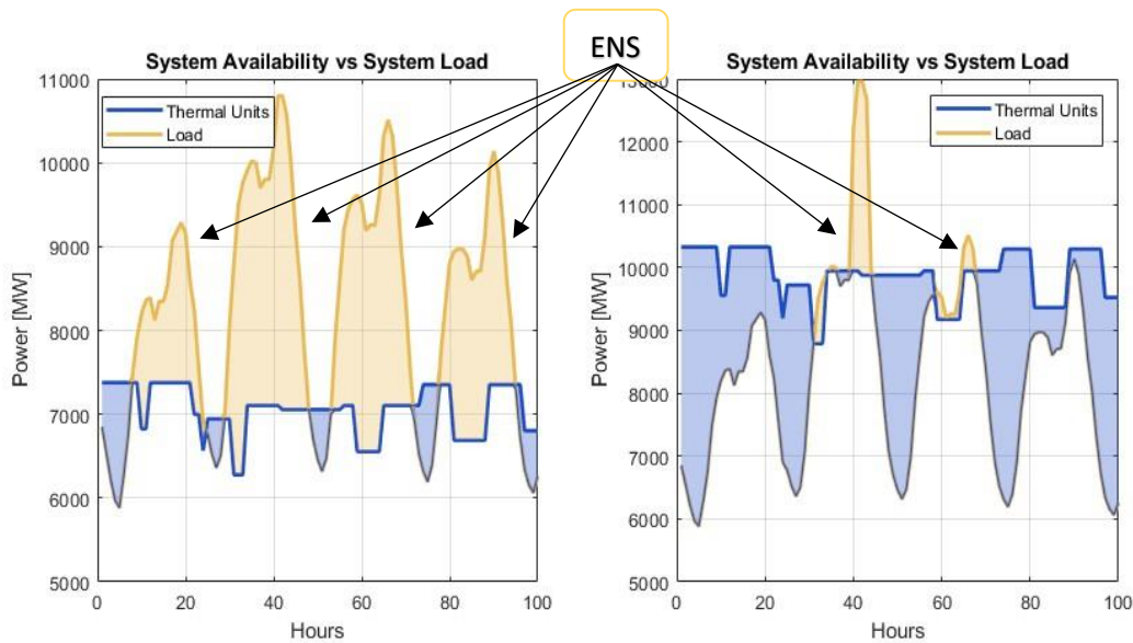
Σχήμα 11: α) Ανεπάρκειες ομοιόμορφα κατανεμημένες στο σύστημα παραγωγής, β) υψηλή ανεπάρκεια σε ώρα αιχμής
