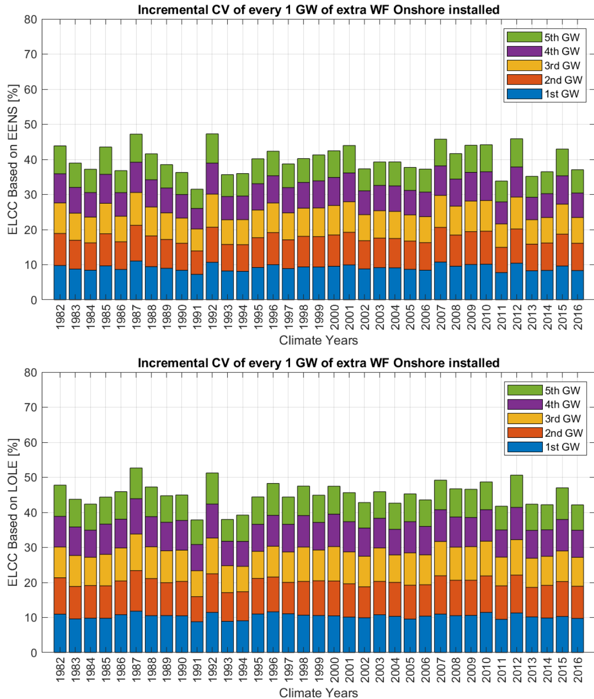
Σχήμα 41: Αποτελέσματα ELCC για σενάρια επιπλέον διεύθυνσης χερσαίων ΑΠ με βάση το (α) EENS και (β) το LOLE
