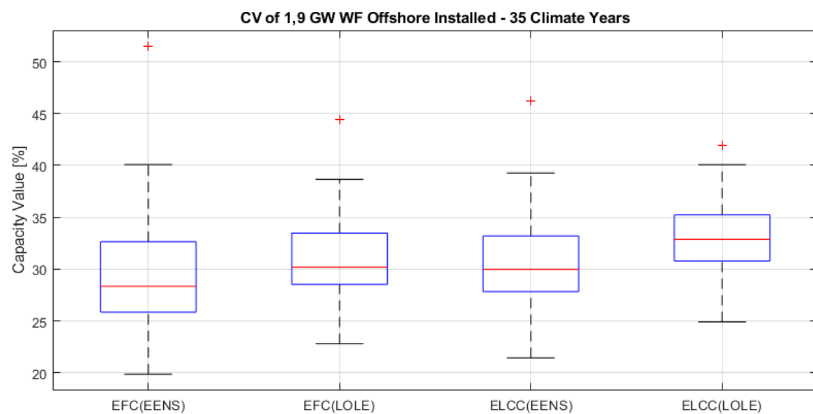
Σχήμα 24: Υπολογισμός Capacity Value για τις υφιστάμενες ΑΠΕ και για τα 35 κλιματικά έτη.
