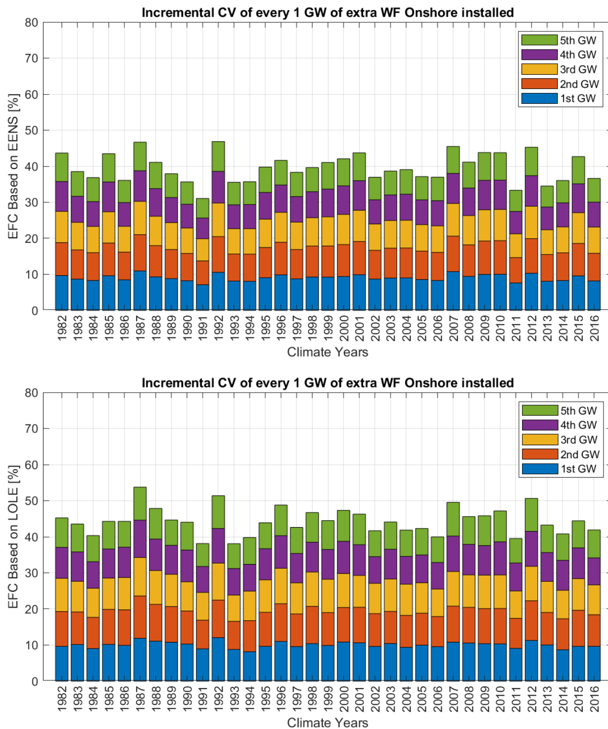
Σχήμα 40: Αποτελέσματα EFC για σενάρια επιπλέον διεύθυνσης χερσαίων ΑΠ με βάση το (α) EENS και (β) το LOLE
