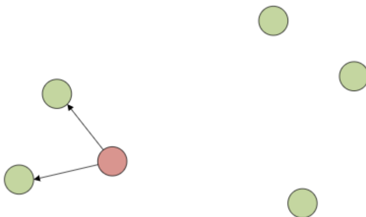
Εικόνα 1: Ο κανόνας των κ-Πλησιέστερων Γειτόνων, για \kappa=2
