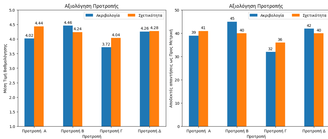
Εικόνα 33: Αποτελέσματα Αξιολόγησης Προτροπής Μεγάλου Γλωσσικού Μοντέλου
