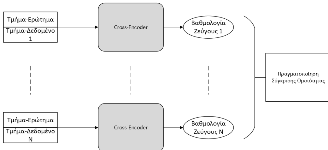
Εικόνα 12: Σύγκριση Ομοιότητας Μεταξύ Ενός Τμήματος-Ερώτημα και N Τμημάτων-Δεδομένων, με Χρήση Cross-Encoder
