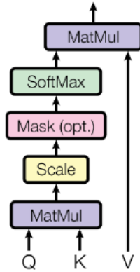
Εικόνα 5: Μηχανισμός Προσοχής Κλιμακωτού Εσωτερικού Γινομένου [16]
