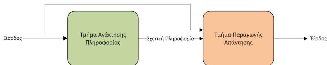
Εικόνα 23: Περιληπτική Λειτουργία του Μοτίβου Ανάπτυξης RAG
