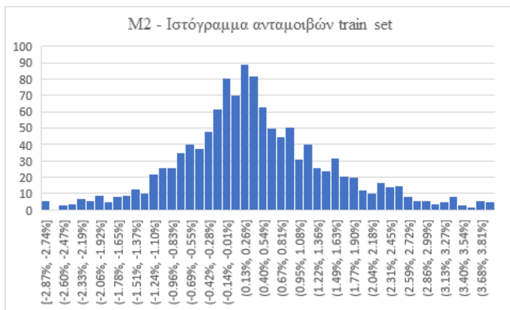
Σχήμα 5.11 M2 - Ιστόγραμμα ανταμοιβών train set
