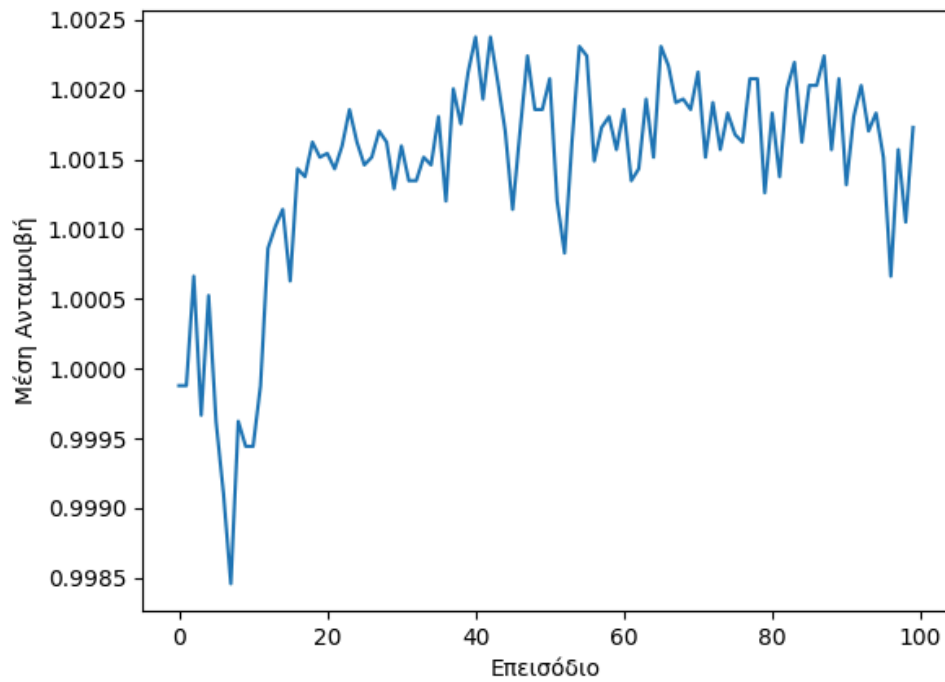
Σχήμα 5.9 M2 - Μέση ανταμοιβή ανά επεισόδιο στο test set
