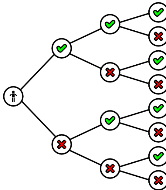
Σχήμα 3.4 Δέντρα Αποφάσεων
