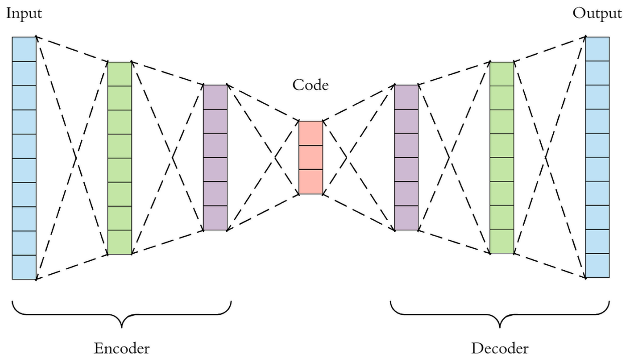
Σχήμα 3.10 Αυτοενσωματωτής
