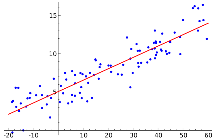
Σχήμα 3.1 Γραμμική Παλινδρόμηση
