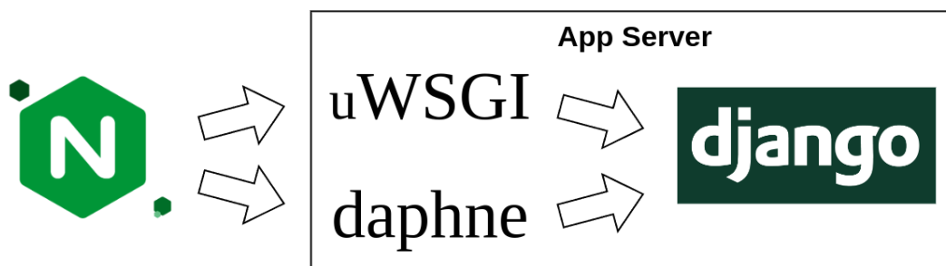
Εικόνα 8.1: Εσωμάτωση του Django στον App Server [56], [57].
