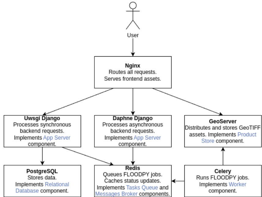
Εικόνα 11.2: Δομή των Docker Containers της εγκατάστασης στο περιβάλλον παραγωγής.
