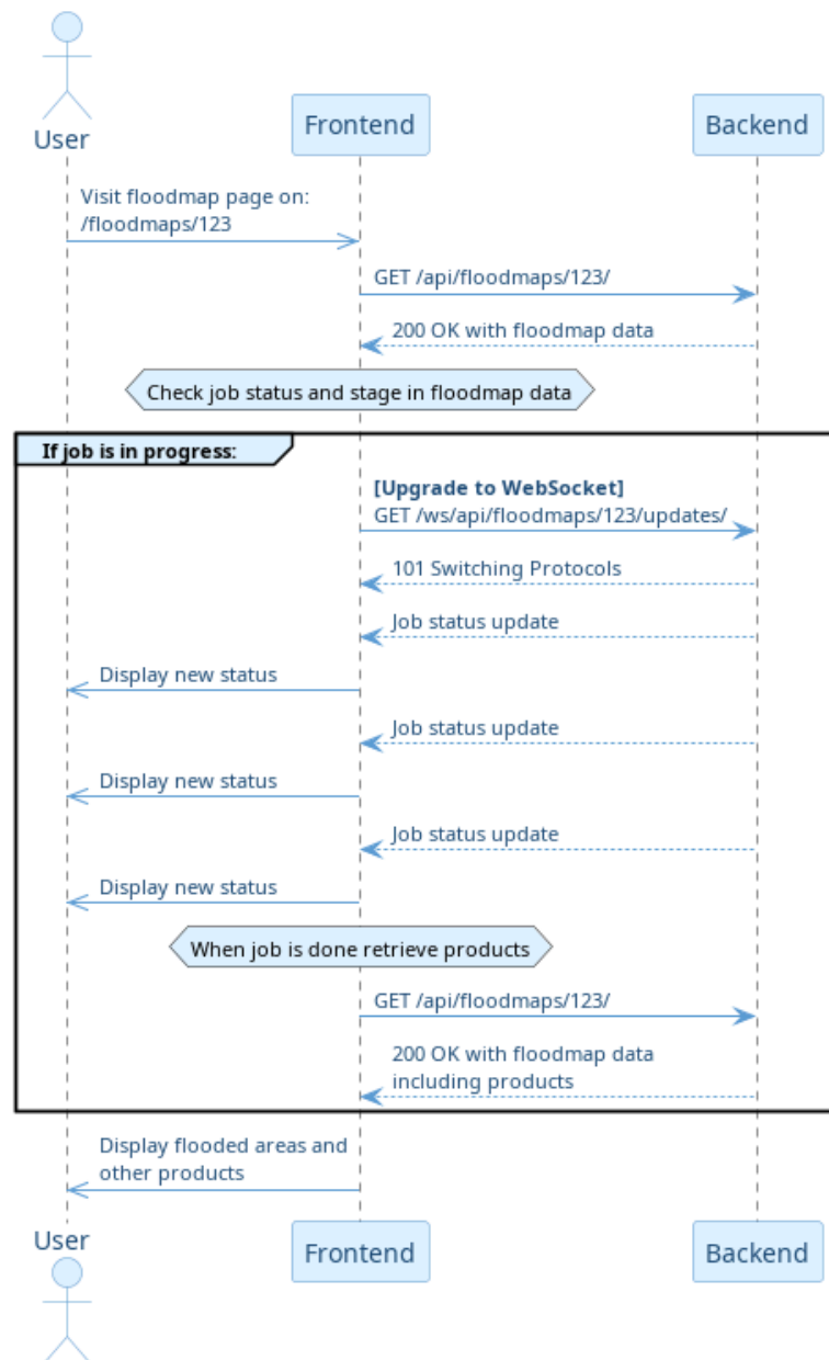
Εικόνα 5.6: Αλληλεπίδραση χρήστη, frontend και backend κατά την παρουσίαση μιας αποθηκευμένης χαρτογράφησης.
