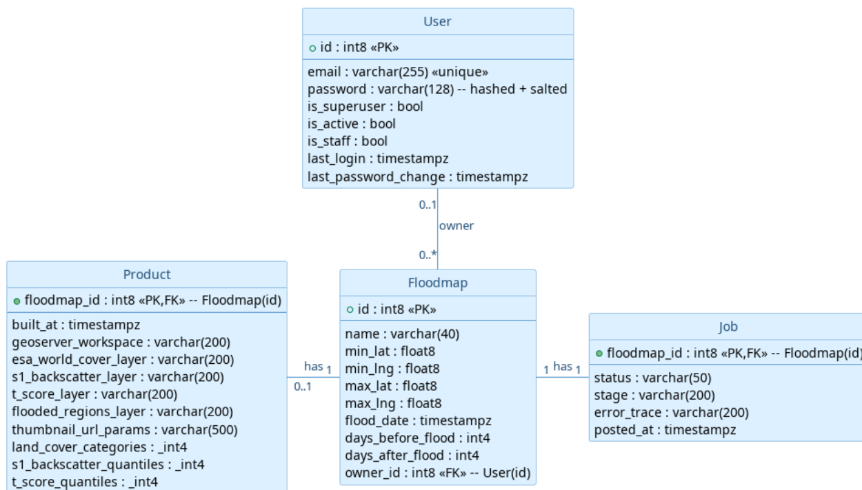
Εικόνα 9.1: Πίνακες της σχεσιακής βάσης δεδομένων του backend.
