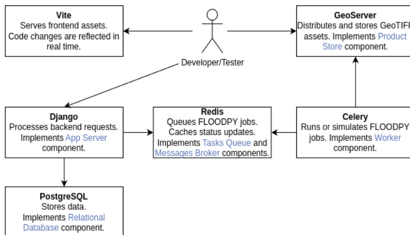
Εικόνα 11.1: Δομή των Docker Containers της εγκατάστασης στο περιβάλλον ανάπτυξης.
