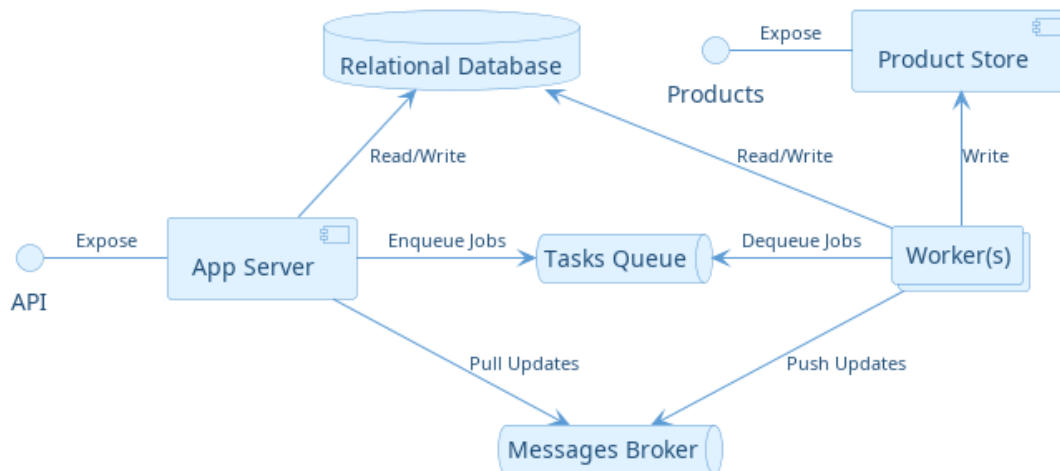
Εικόνα 9.2: Αρχιτεκτονική του backend.
