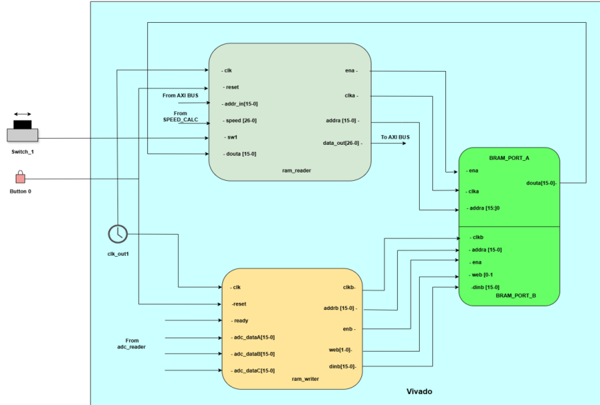
Εικόνα 4.14: Περιγραφική απεικόνιση μεταφοράς δεδομένων στο περιβάλλον Vitis.
