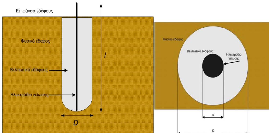
Σχήμα 5.2: Ηλεκτρόδιο γείωσης τοποθετημένο μέσα στο βελτιωτικό έδαφος.
