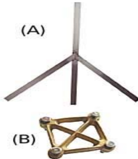
Σχήμα 1.26: Ακτινικός γειωτής
