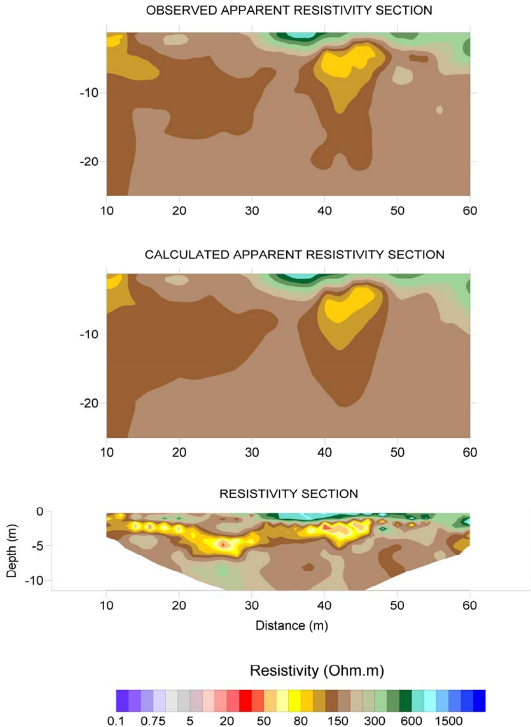
Σχήμα 5.39: Γράφημα ηλεκτροτομογραφίας στο χώρο του πειράματος.
