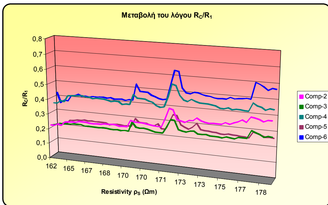
Σχήμα 5.33: Σχέση αντίστασης γείωσης - ειδικής αντίστασης εδάφους.
