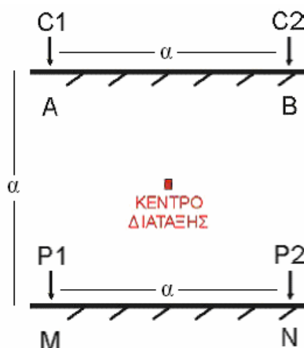
Σχήμα 2.11: Τετραγωνική διάταξη.
