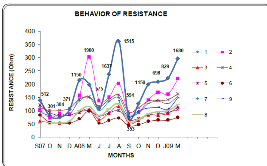
Σχήμα 4.2: Μεταβολή της αντίστασης γείωσης των υπό εξέταση ηλεκτροδίων σε συνάρτηση με το χρόνο, σε ασβεστολιθικό βραχώδες έδαφος [13].
