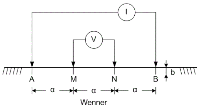
Σχήμα 2.5: Διάταξη Wenner [1].
