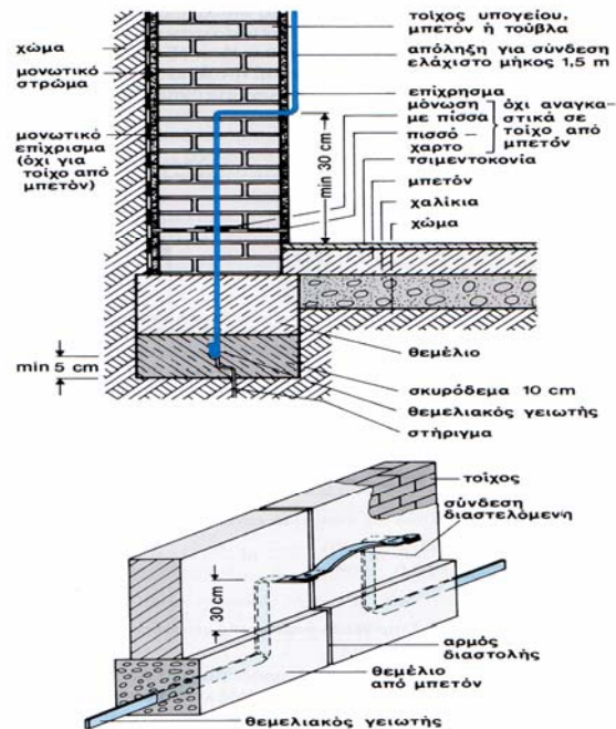
Σχήμα 1.36: Λεπτομέρειες θεμελιακής γείωσης.
