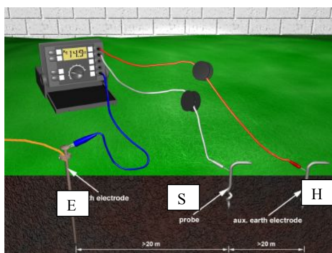
Εικόνα 2.2: Συνδεσμολογία μέτρησης της ειδικής αντίστασης με τη μέθοδο των τριών ηλεκτροδίων [10].
