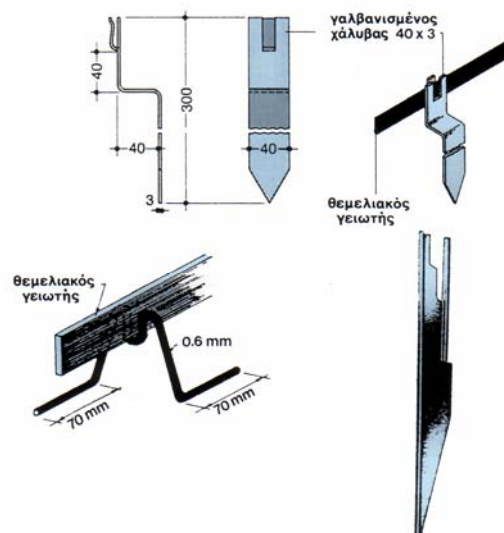
Σχήμα 1.37: Στηρίγματα θεμελιακής γείωσης.
