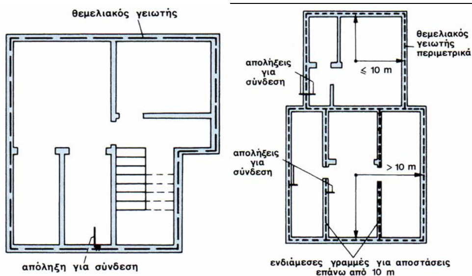
Σχήμα 1.35: Κατόψεις θεμελιακών γειώσεων με και χωρίς εγκάρσια και διαμήκη τμήματα.
