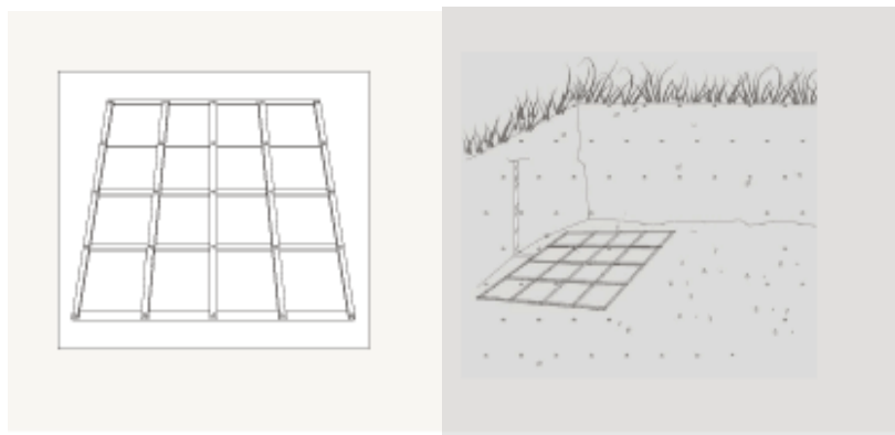
Σχήμα 1.27: Γειωτής πλέγματος
