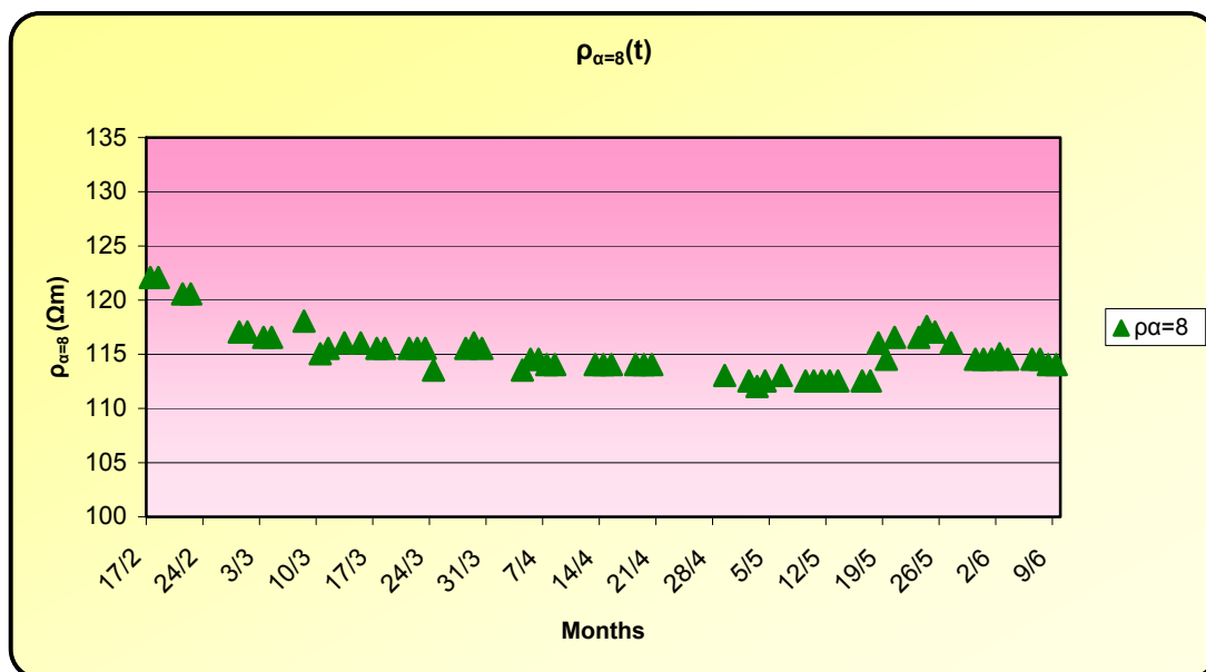
Σχήμα 5.5: Μεταβολή της \rho_s με το χρόνο για \alpha=8m .
