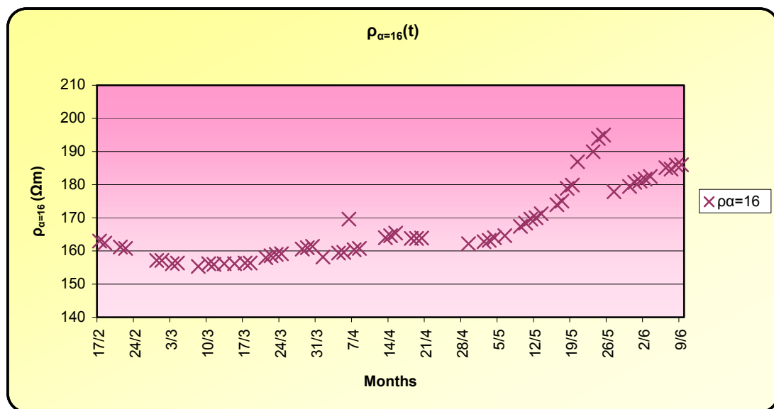
Σχήμα 5.7: Μεταβολή της \rho_s με το χρόνο για \alpha=16m .
