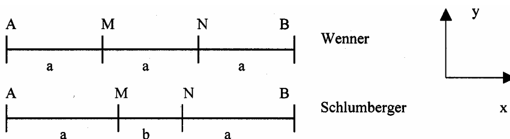
Σχήμα 2.6: Διάταξη τεσσάρων ηλεκτροδίων κατά Wenner και Schlumberger [2].
