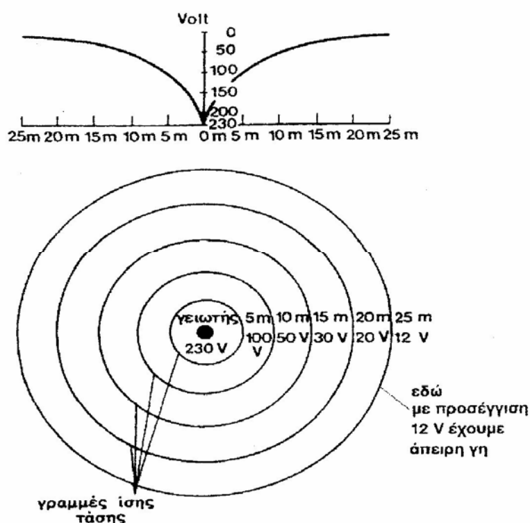
Σχήμα 3.1: Χοάνη δυναμικού.
