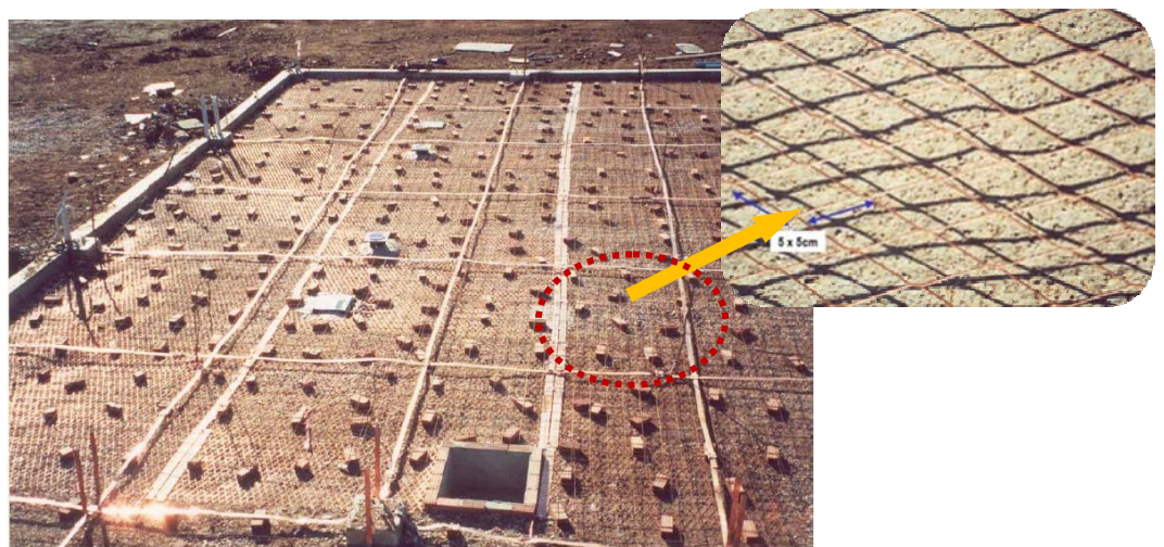
Εικόνα 1.6: Θεμελιακή γείωση πλέγματος.
