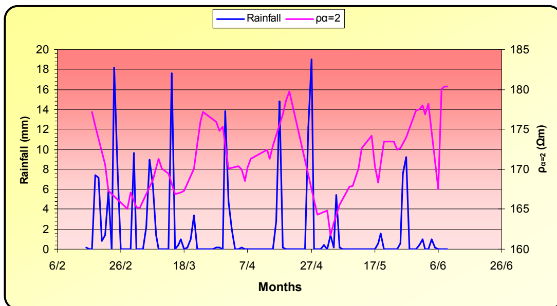
Σχήμα 5.9: Μεταβολή της \rho_s με τη βροχόπτωση για \alpha=2m .
