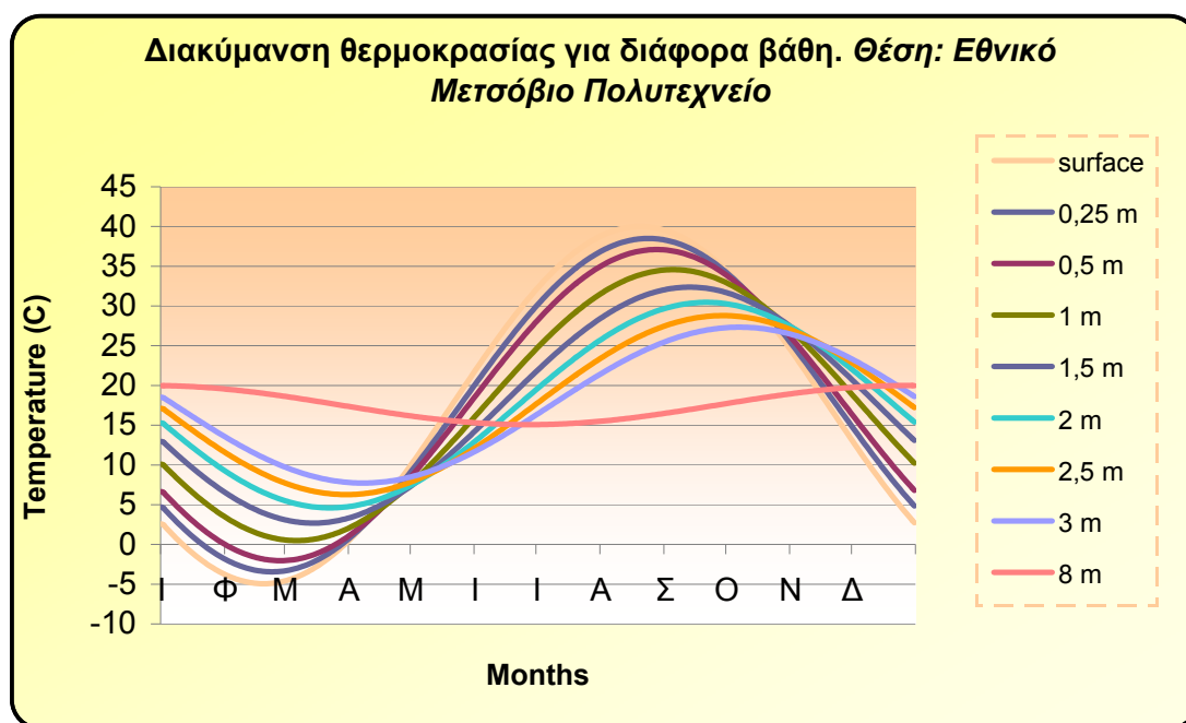
Σχήμα 5.35: Διακύμανση της θερμοκρασίας εδάφους για διάφορα βάθη.
