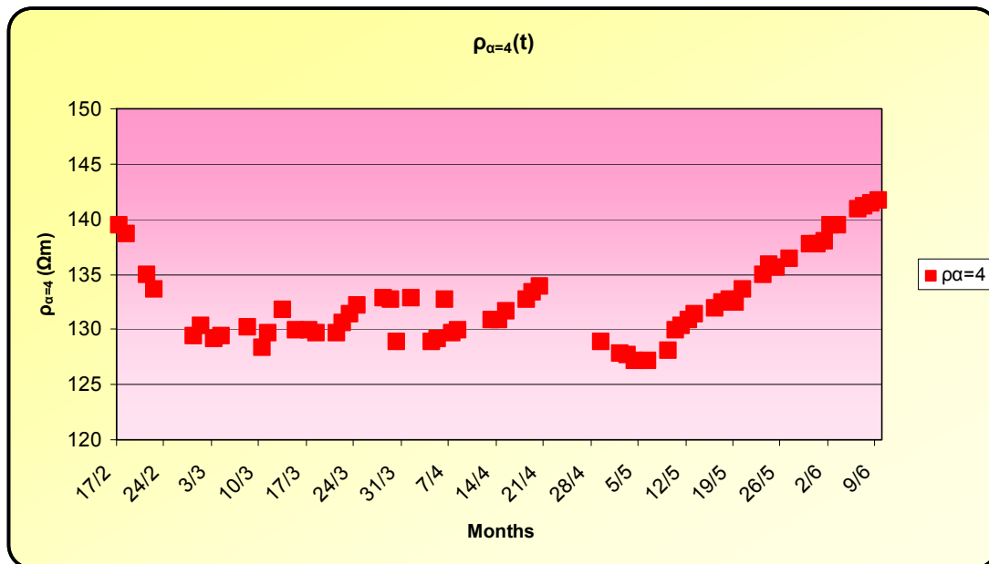
Σχήμα 5.4: Μεταβολή της \rho_s με το χρόνο για \alpha=4m .
