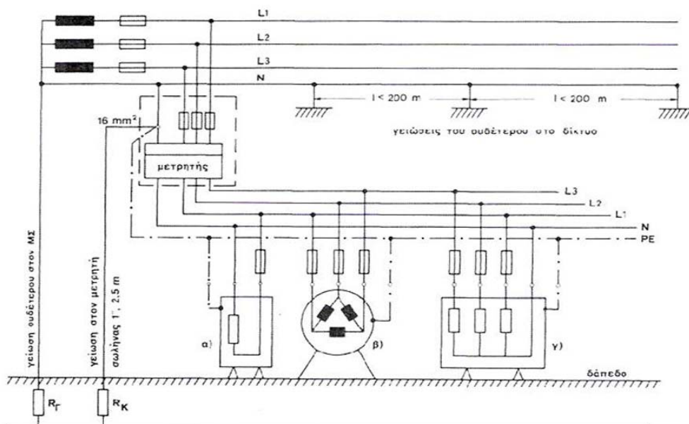
Σχήμα 1.4: Σχηματική παρουσίαση συστήματος προστασίας με ουδετέρωση.
