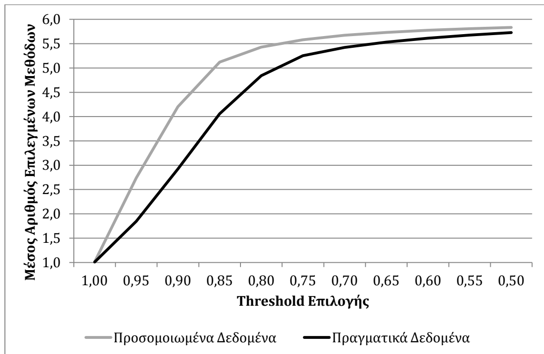
Σχήμα 7.3 - Σύγκριση προσομοιωμένων και πραγματικών δεδομένων ως προς το μέσο αριθμό επιλεγμένων μεθόδων για τη συμμετοχή στο βέλτιστο συνδυασμού σε συνάρτηση με το επιλεγμένο threshold
